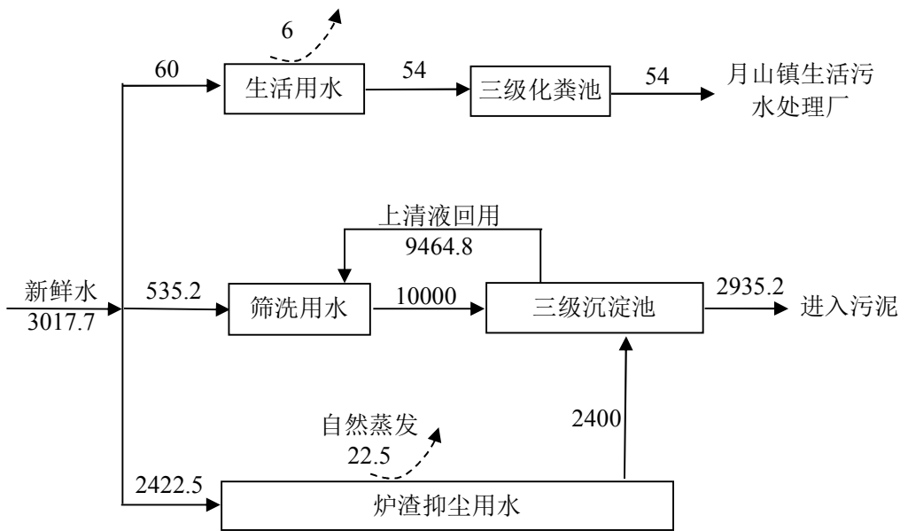
图 2-1 项目水平衡图 (单位: m³/a)
