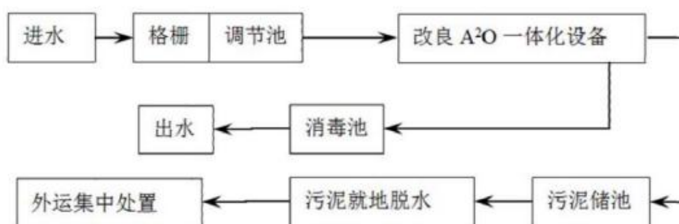
图 4-1 月山镇生活污水处理厂水处理工艺流程图
