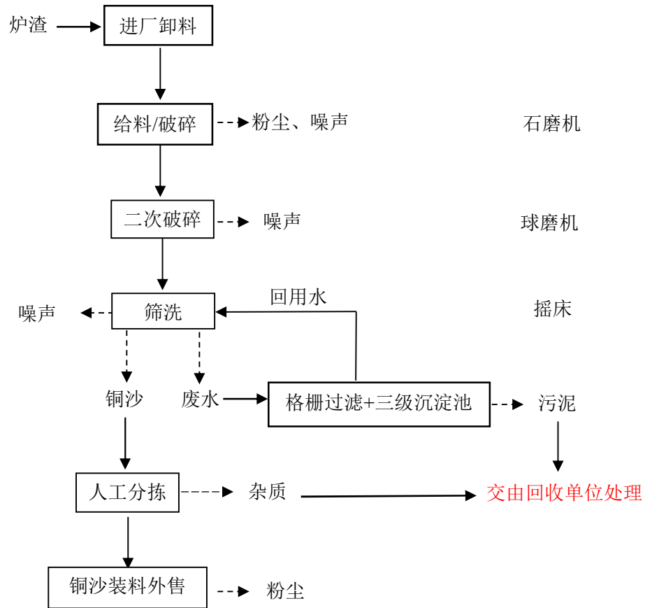
图2-3 项目炉渣筛洗工艺流程图
