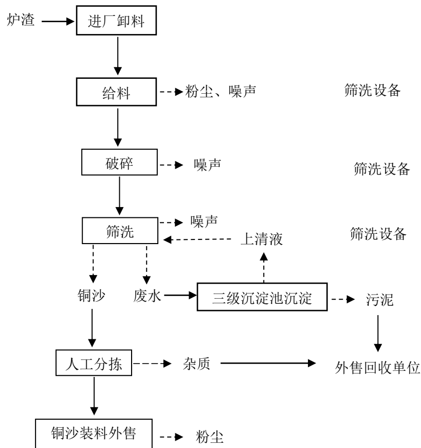
②炉渣筛洗工艺流程及说明（已批复，未建设）
