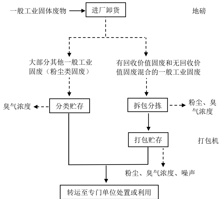
图2-3 项目储运工艺流程图
