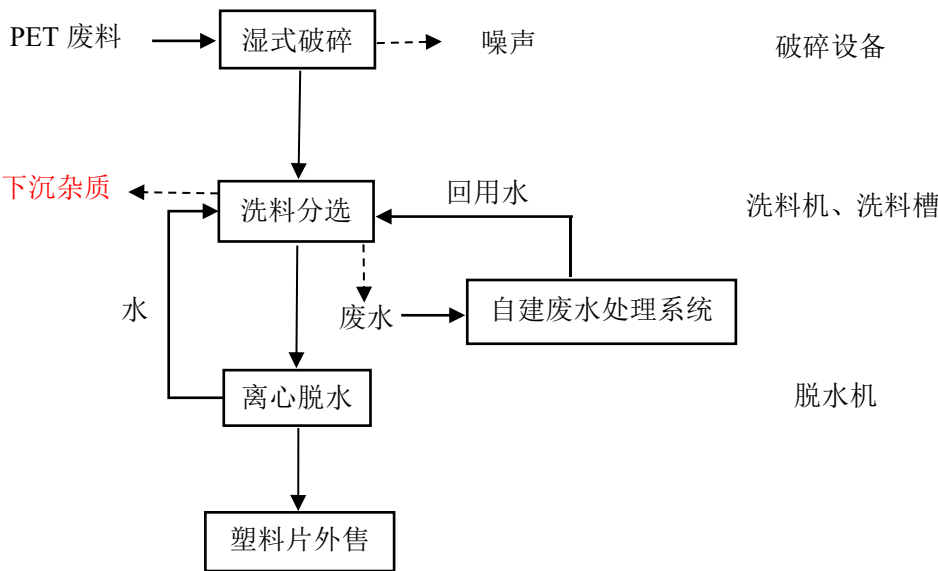
图2-5 项目废塑料筛洗工艺流程图
