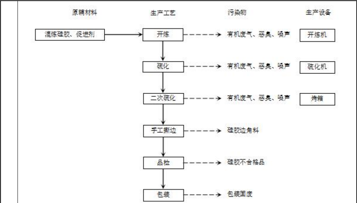
图2-4 硅胶制品生产工艺流程图
