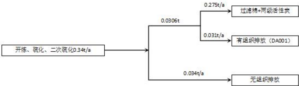
图 2-1 项目 VOC 平衡图 (t/a)
