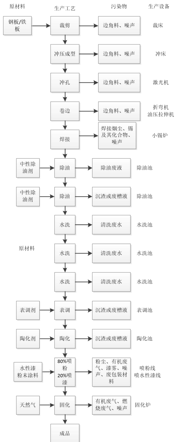
图 2-4 项目燃气灶工艺流程图
