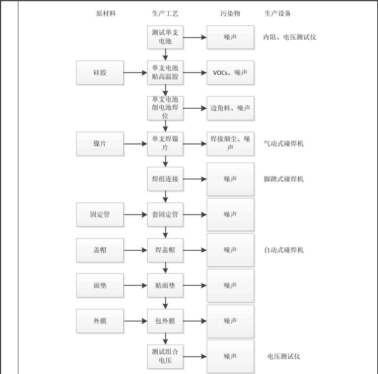
图 2-3 项目锂电池组工艺流程图
