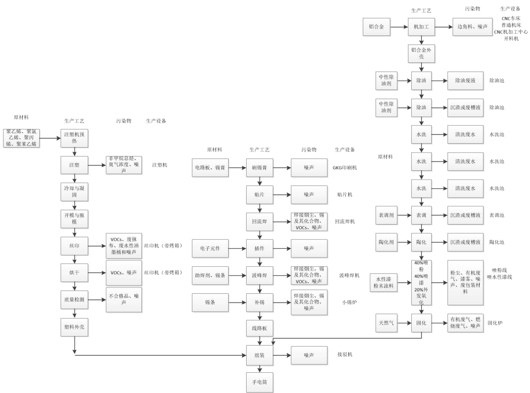
图 2-2 项目手电筒工艺流程图
