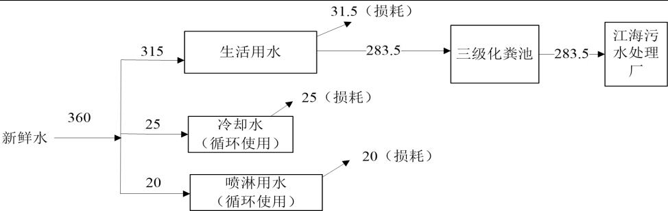
图2-1 原项目水平衡图
