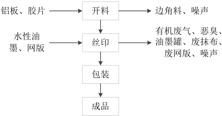
图 2-3 铝铭牌、功能面板生产工艺流程图
