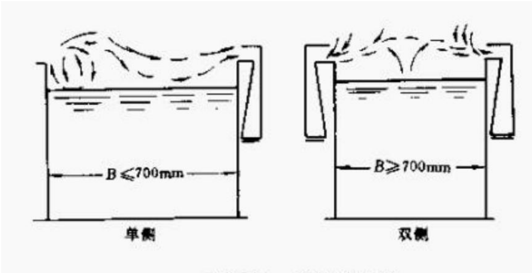
图 4-1 槽边集气罩示意图
