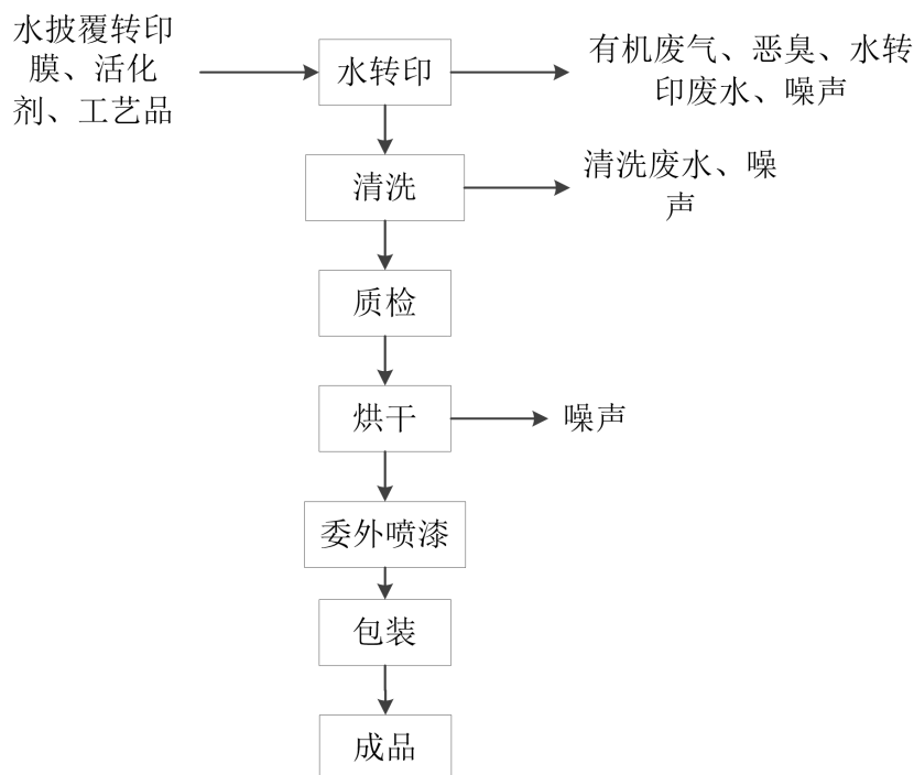
图 2-5 工艺品生产工艺流程图
