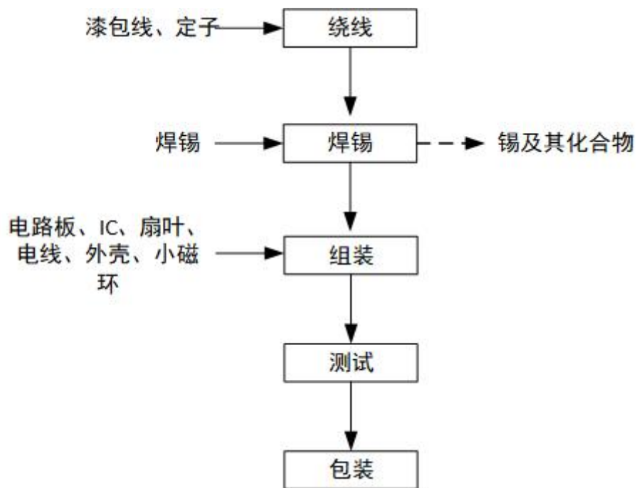
图 2-4 风扇生产工艺流程图
