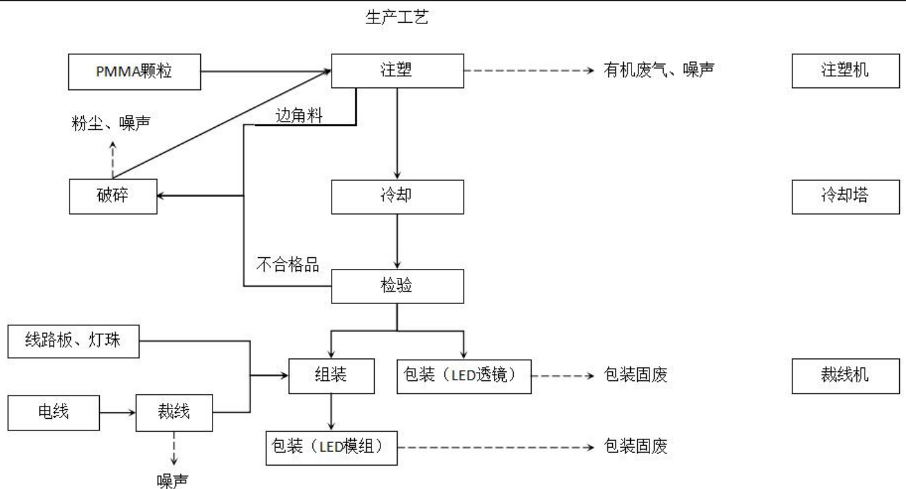
图2-3 LED透镜、LED模组生产工艺流程图
