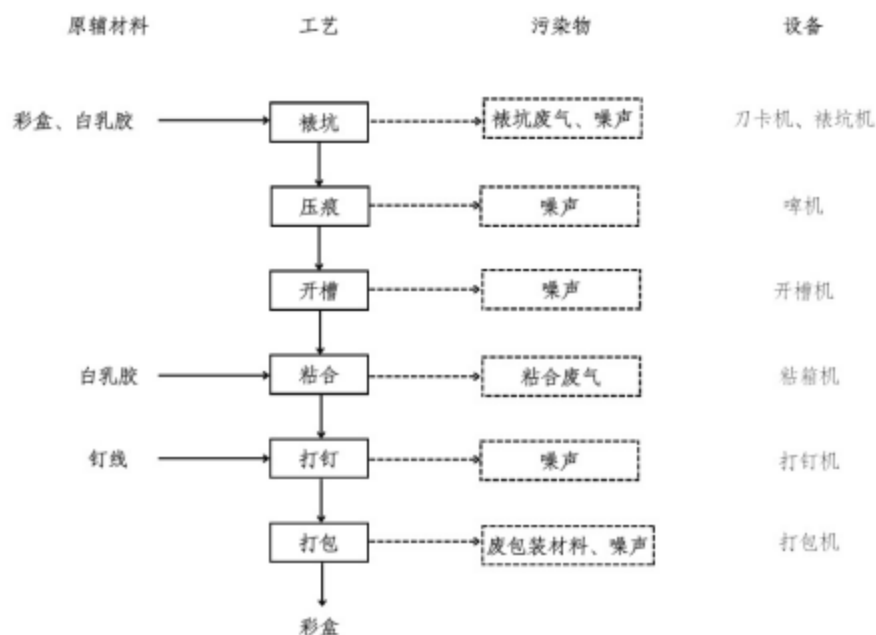
图3. 彩盒生产工艺流程图
