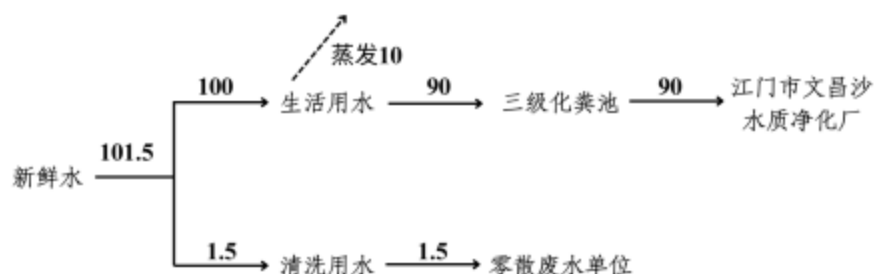
图 1. 项目水平衡图 (t/a)
