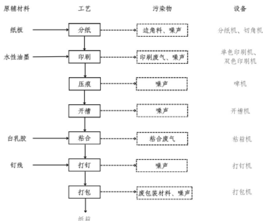
图2. 纸箱生产工艺流程图
