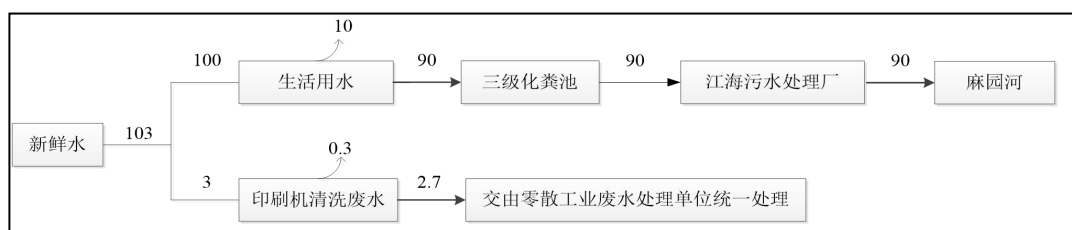
图 2-1 项目水平衡图 (m 3 /a)
