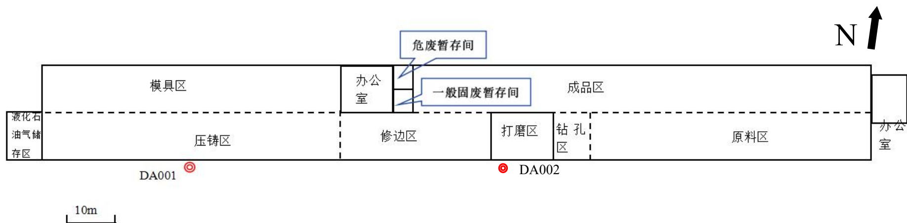
附图 4 项目生产车间平面布置图
