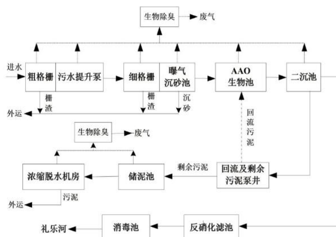
图 4-2 污水厂工艺流程图
