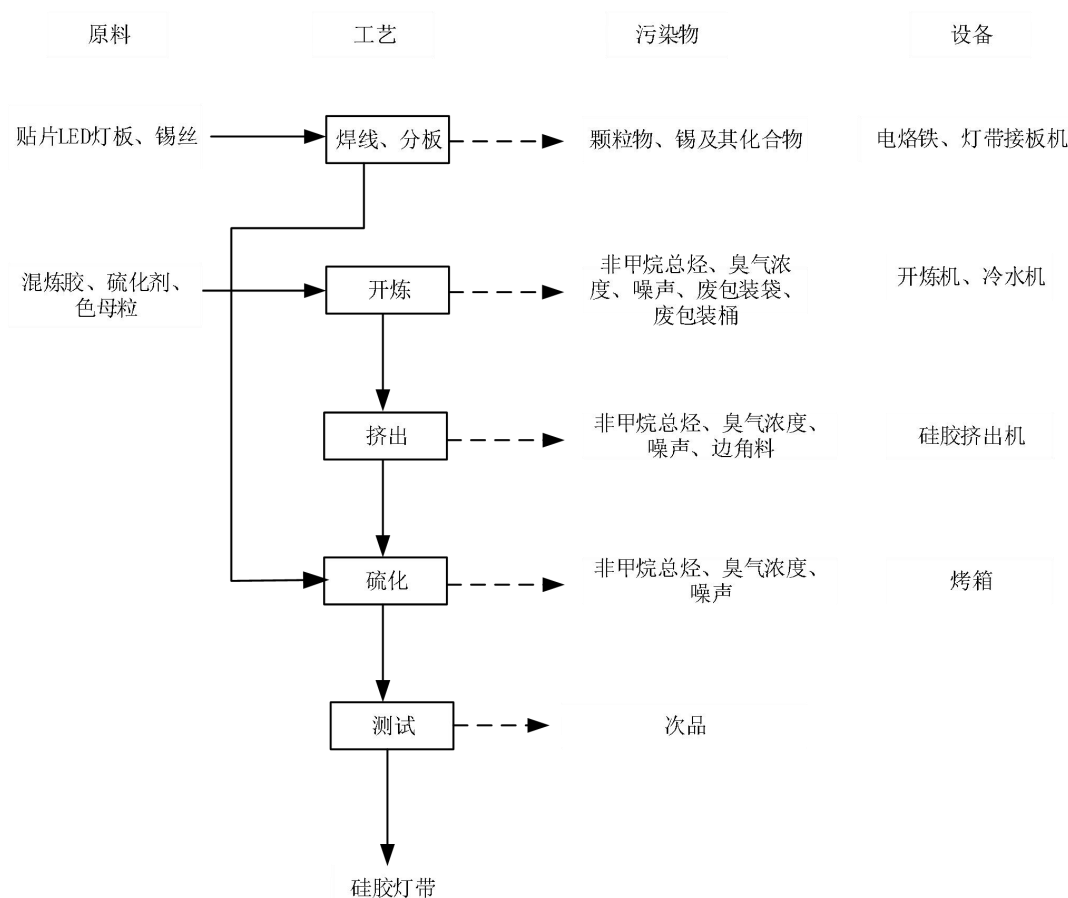
图 2-3 硅胶灯带生产工艺流程图
