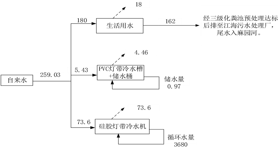
图 2-1 全厂用水平衡图 (单位: t/a)
