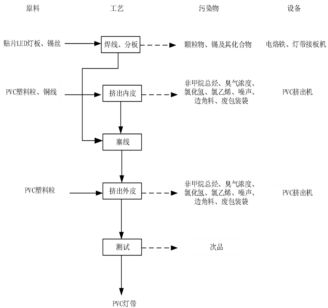
图 2-2 PVC 灯带生产工艺流程图
