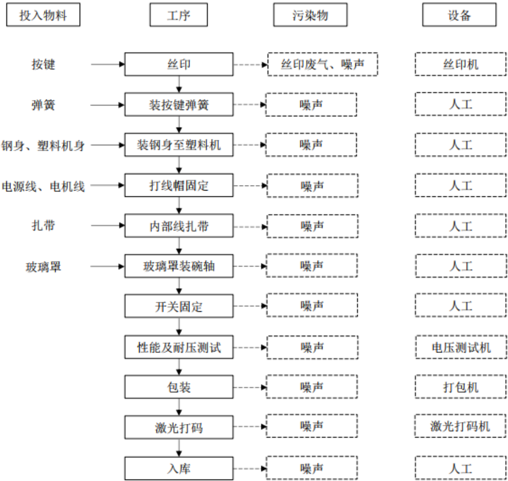
图 2-6 搅拌机组装工艺流程图
