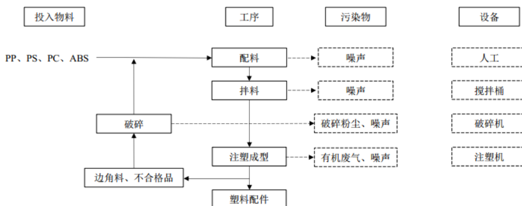
图 2-5 塑料配件生产工艺流程图
