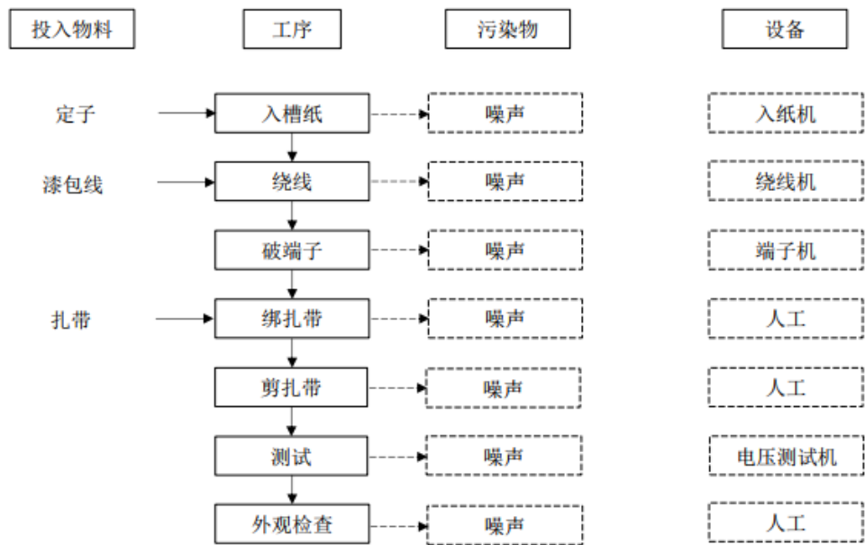
图 2-3 定子生产工艺流程图
