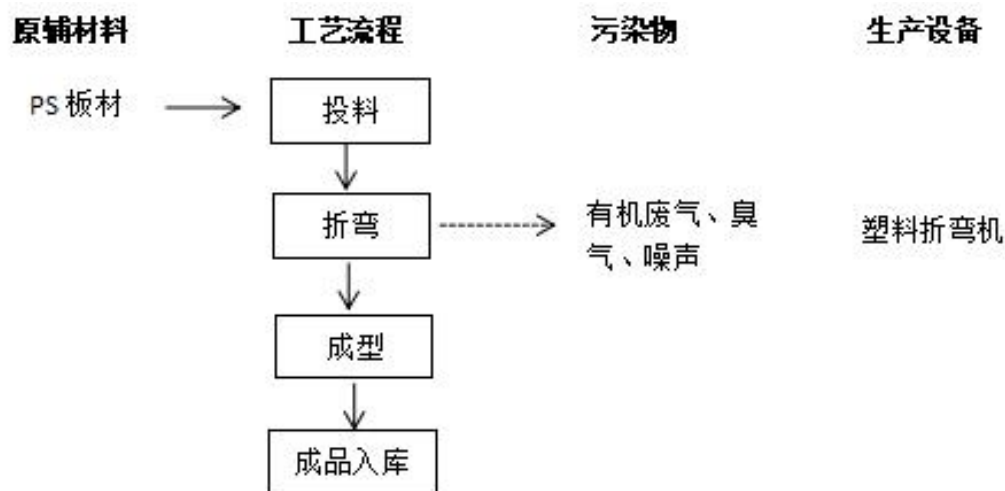
图 2-3 项目铁壳净化灯挤压工艺流程图
