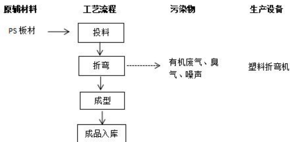
图 2-4 项目压花罩工艺流程图
