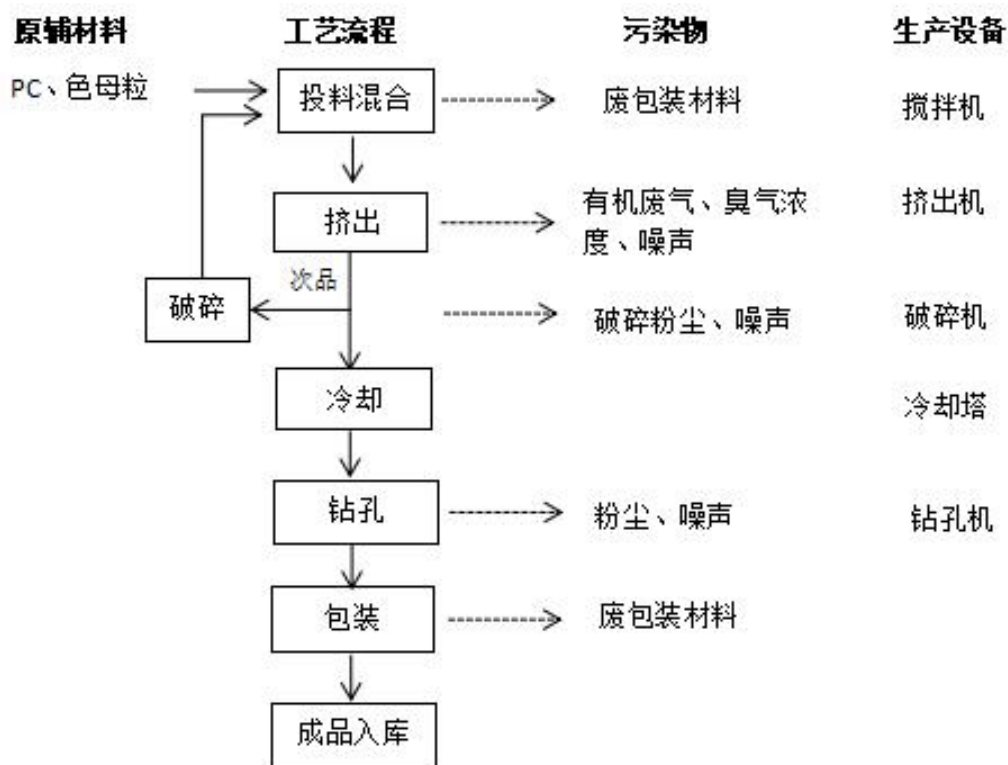
图 2-2 项目 PC 罩、PC 双色管工艺流程图
