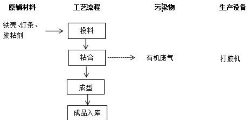
图 2-5 项目贴灯条工艺流程图
