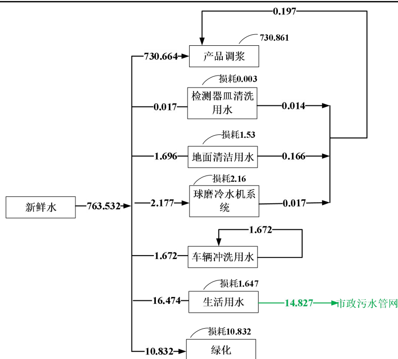
图2.1-1 水平衡图单位: m³/d
