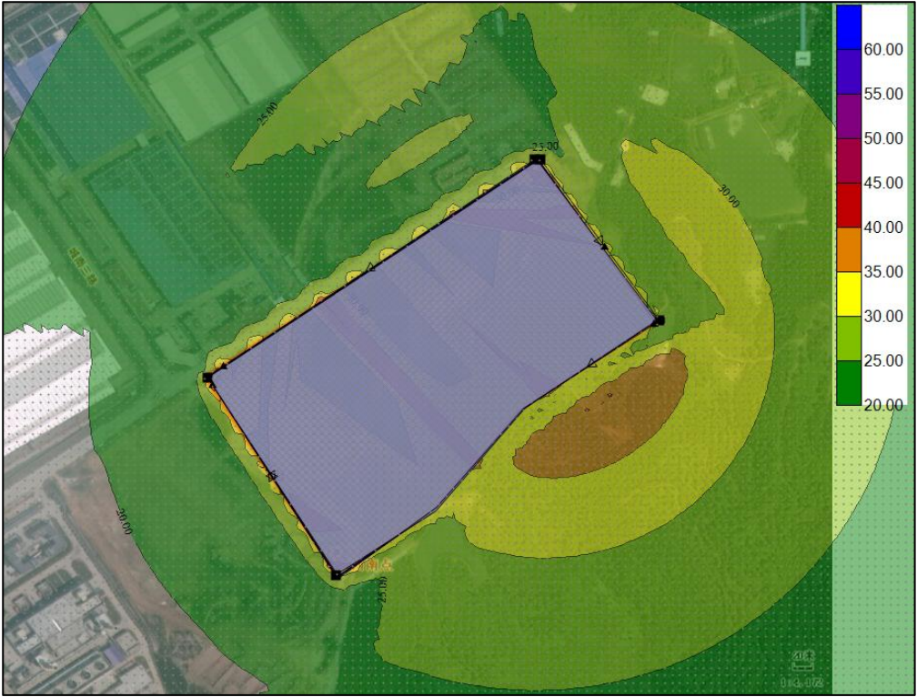
图4.2-3 项目噪声贡献值预测等值线图
