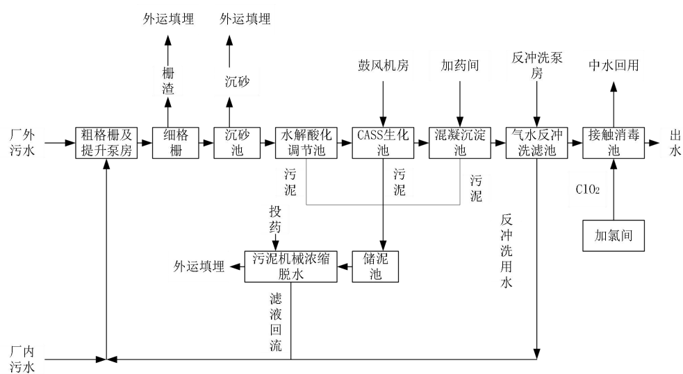
图4.2-1现状污水处理工艺流程图
