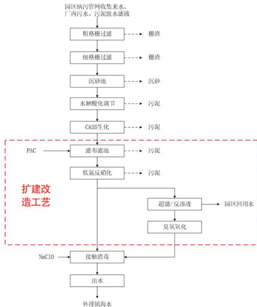
图4.2-2 扩建后污水处理工艺流程图
