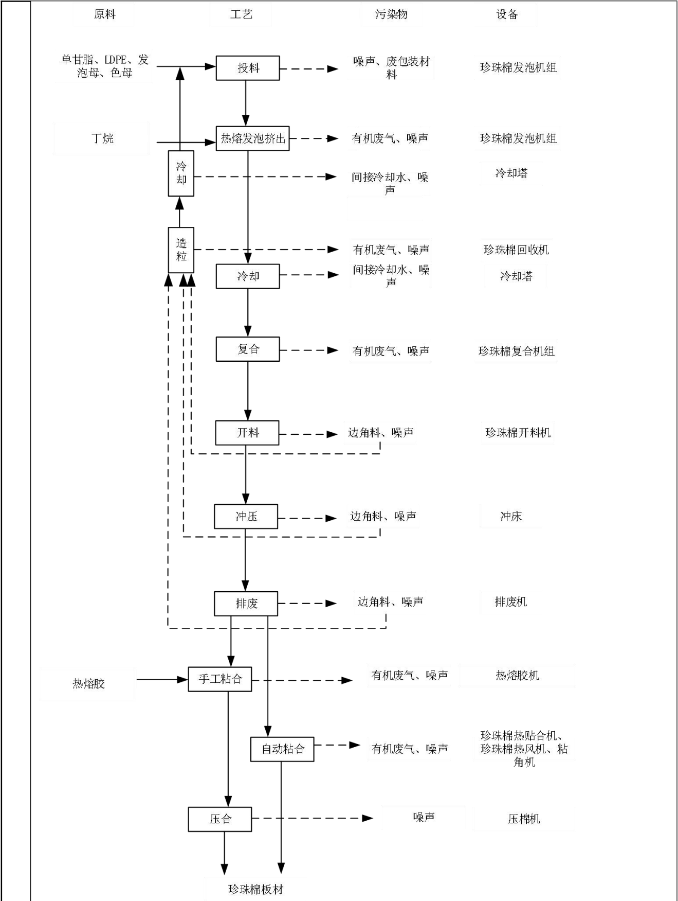
图 2-3 珍珠棉板材生产工艺流程图
