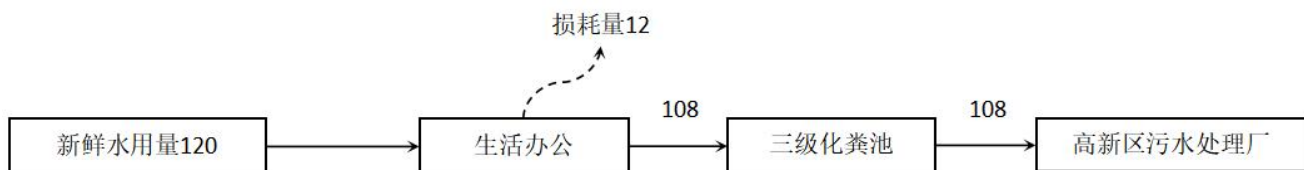
图 2-2 项目水平衡图 (t/a)
