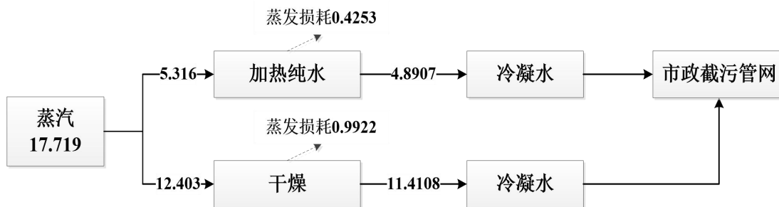
图 2-2 改扩建前项目蒸汽平衡图 (t/d)
