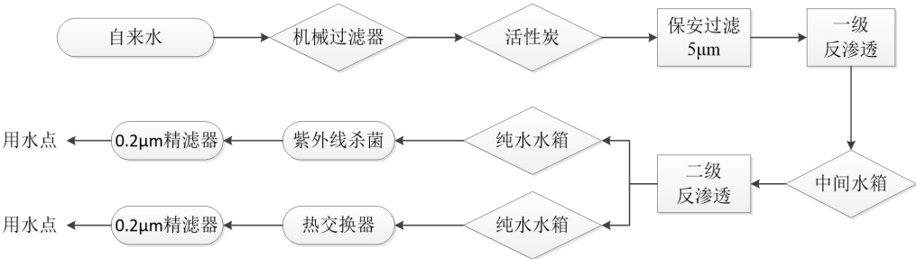
图 2-6 纯水制备工艺流程图
