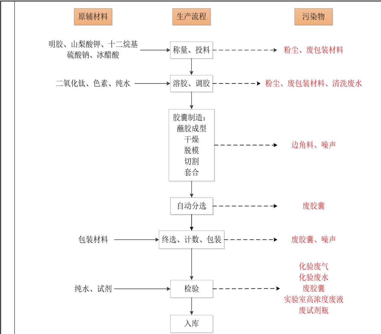
图 2-6 现有项目生产工艺流程图
