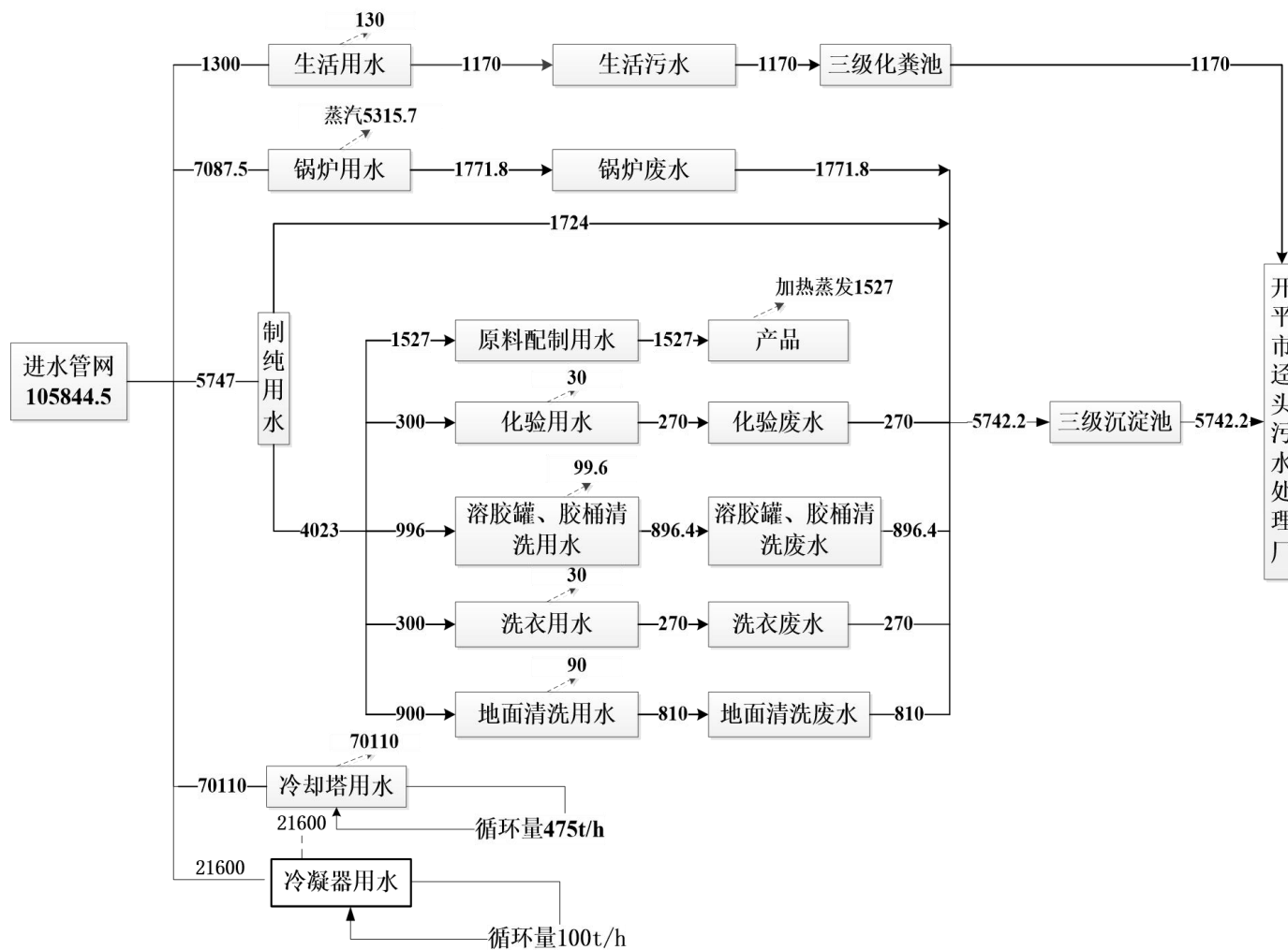
图 2-4 改扩建后项目总水平衡图 (t/a)
