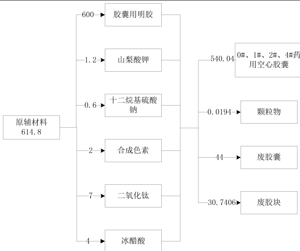
图 2-1 项目物料平衡图 (t/a)
