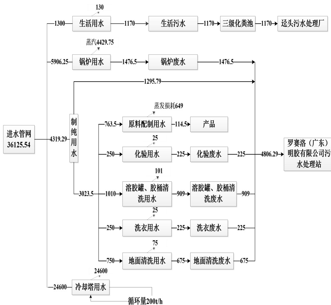
图 2-3 改扩建前项目水平衡图 (单位: t/a)
