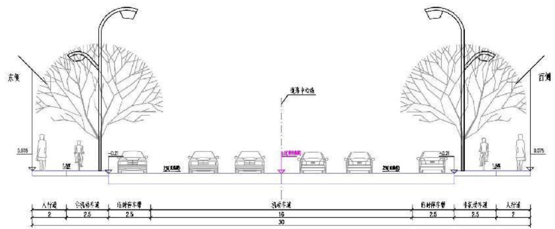
图2-2 横断面布置
