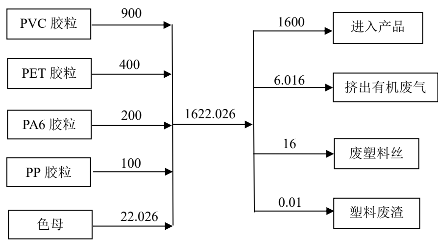
图 2-1 项目物料平衡图 (单位: t/a)
