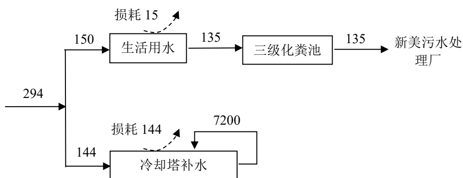
图 2-2 项目用水平衡图 (单位: \text{m}^3/\text{a} )
