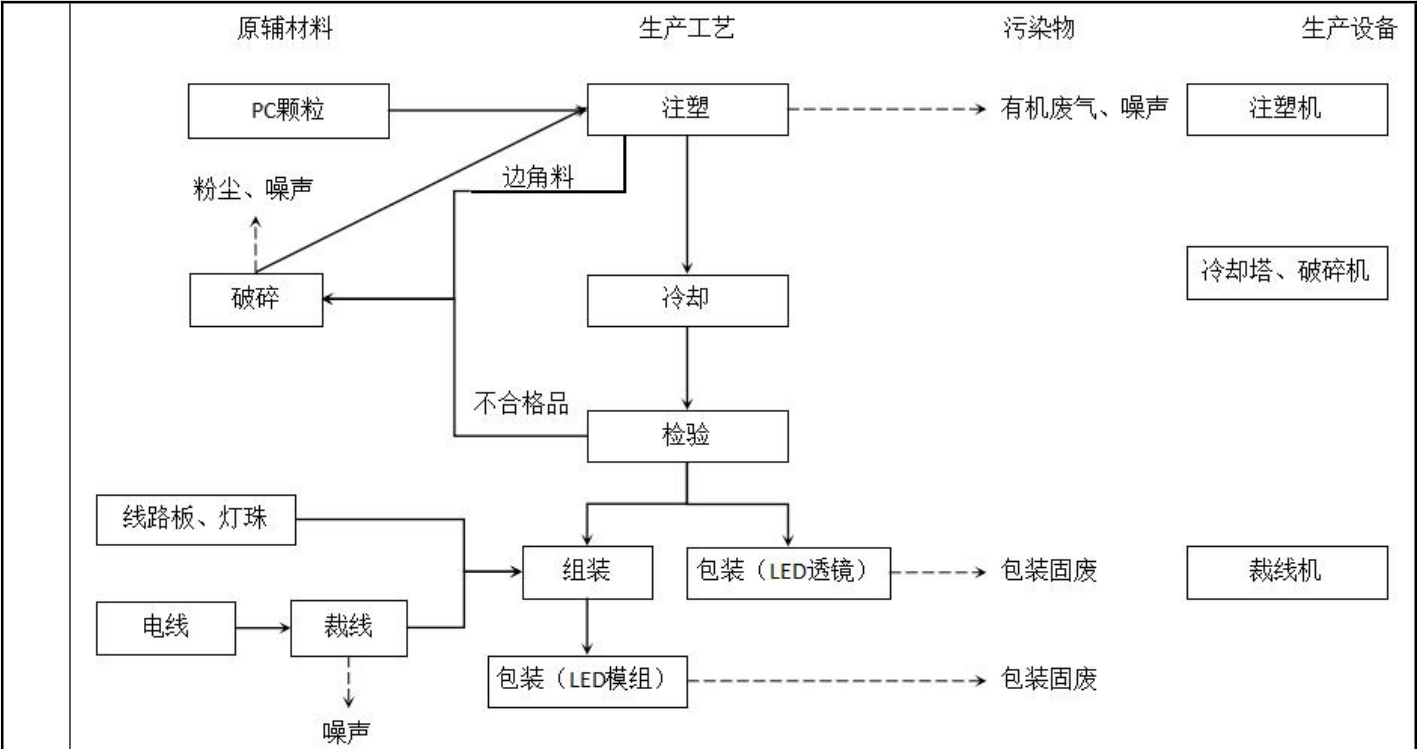
图2-3 LED透镜、LED模组生产工艺流程图
