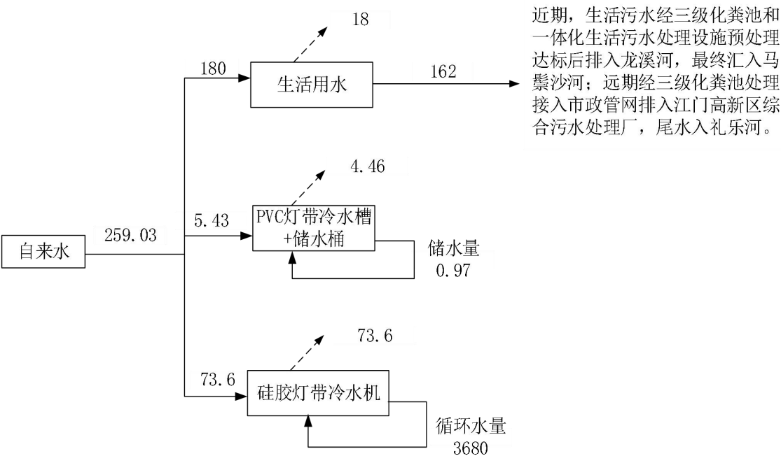
图 2-1 全厂用水平衡图（单位：t/a）
