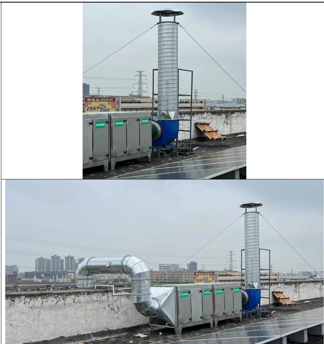
图 4-1 项目挤出、注塑工位废气收集、处理措施示意图
