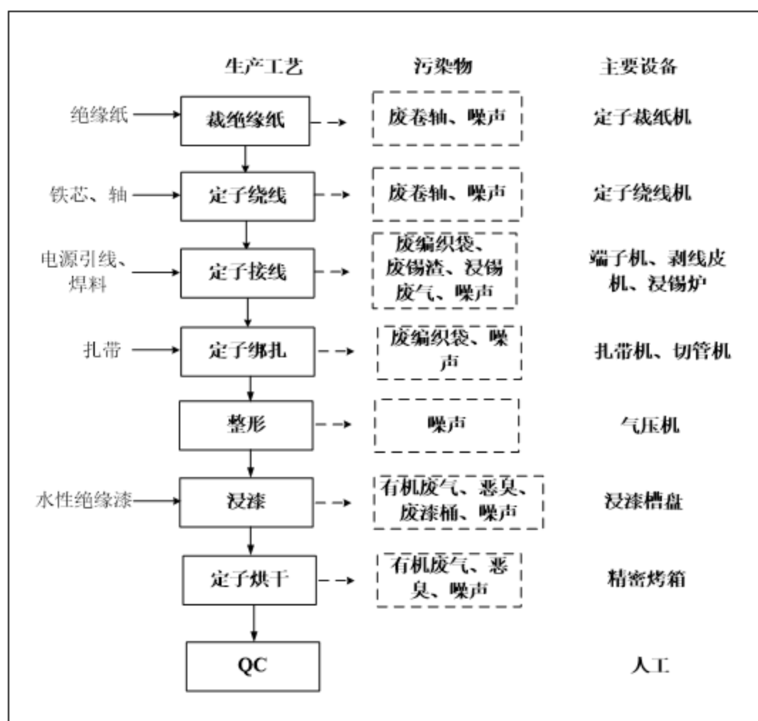
图 2-3 定子工艺流程图
