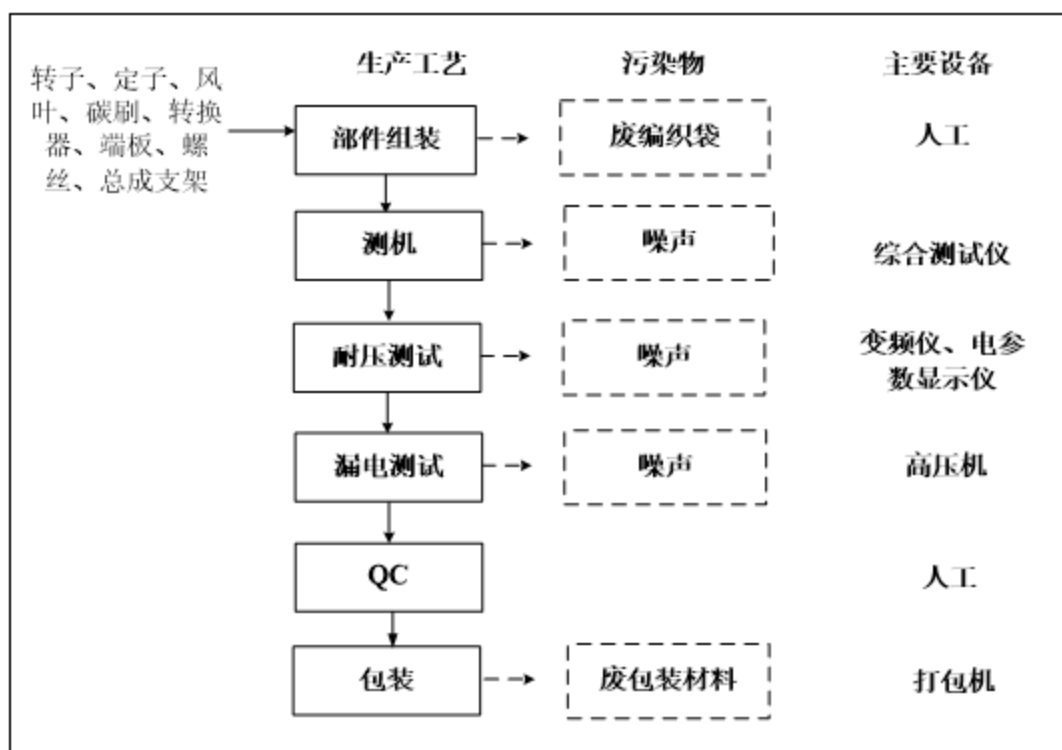
图 2-4 总装工艺流程图
