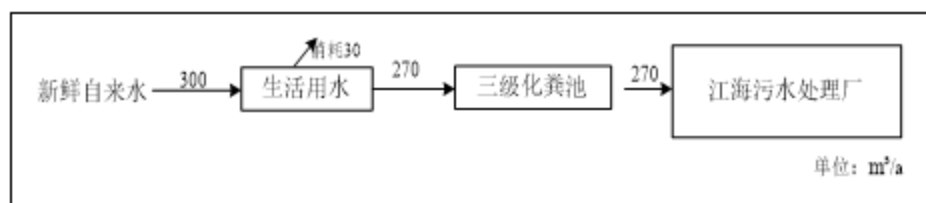
图 2-1 项目水平衡图
