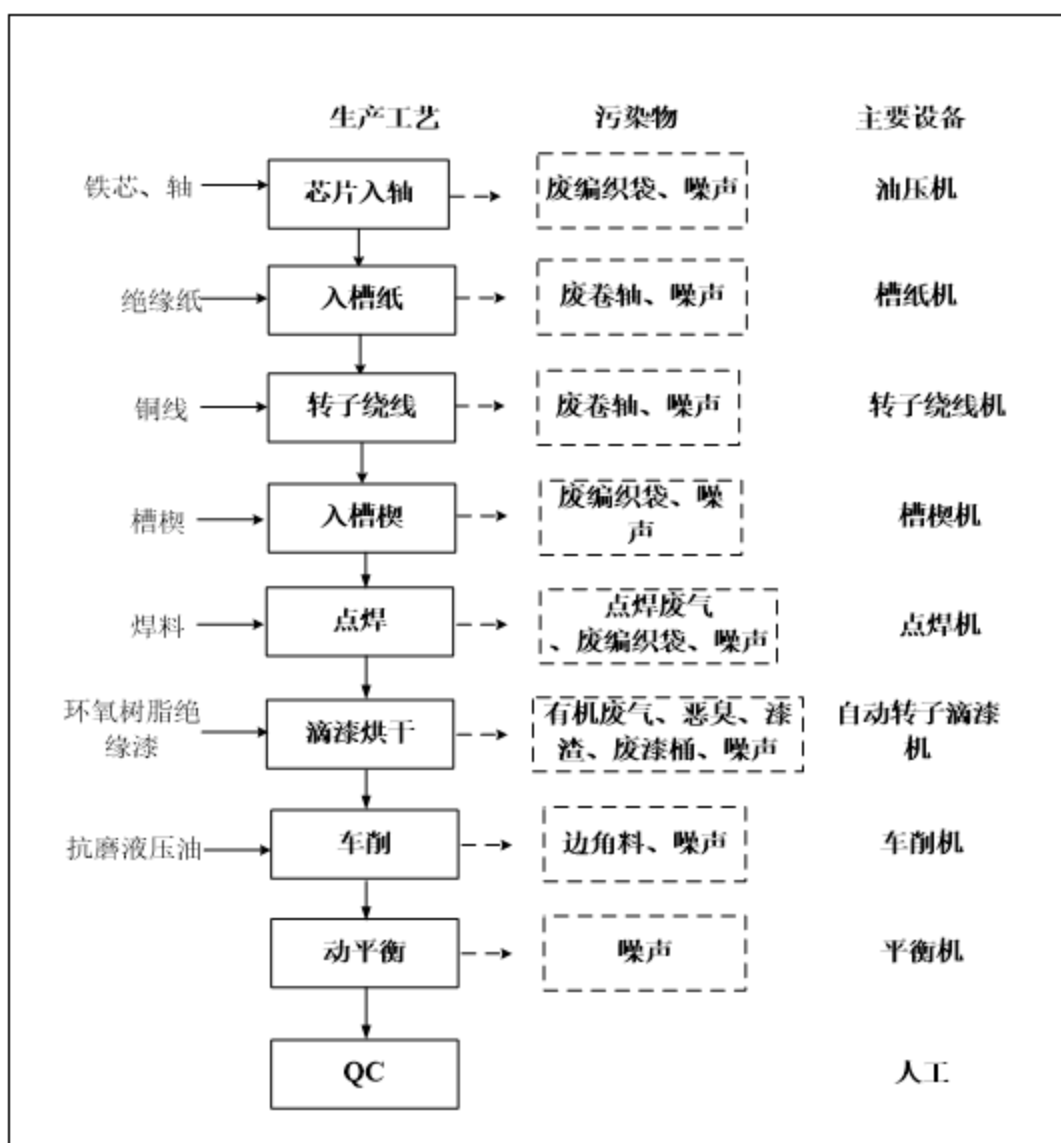
图 2-2 转子工艺流程图
