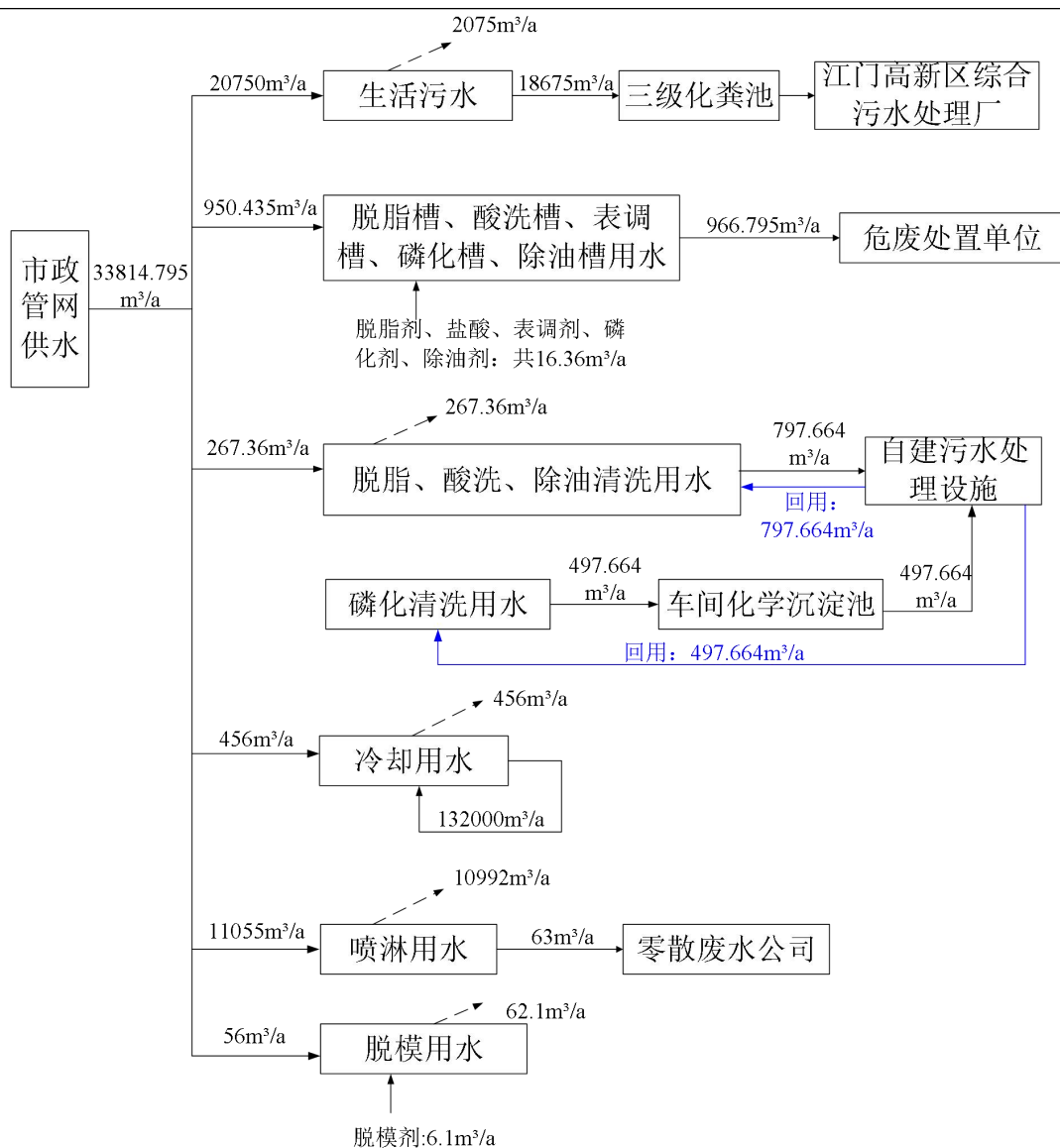
图 2-2 扩建后全厂水平衡图
