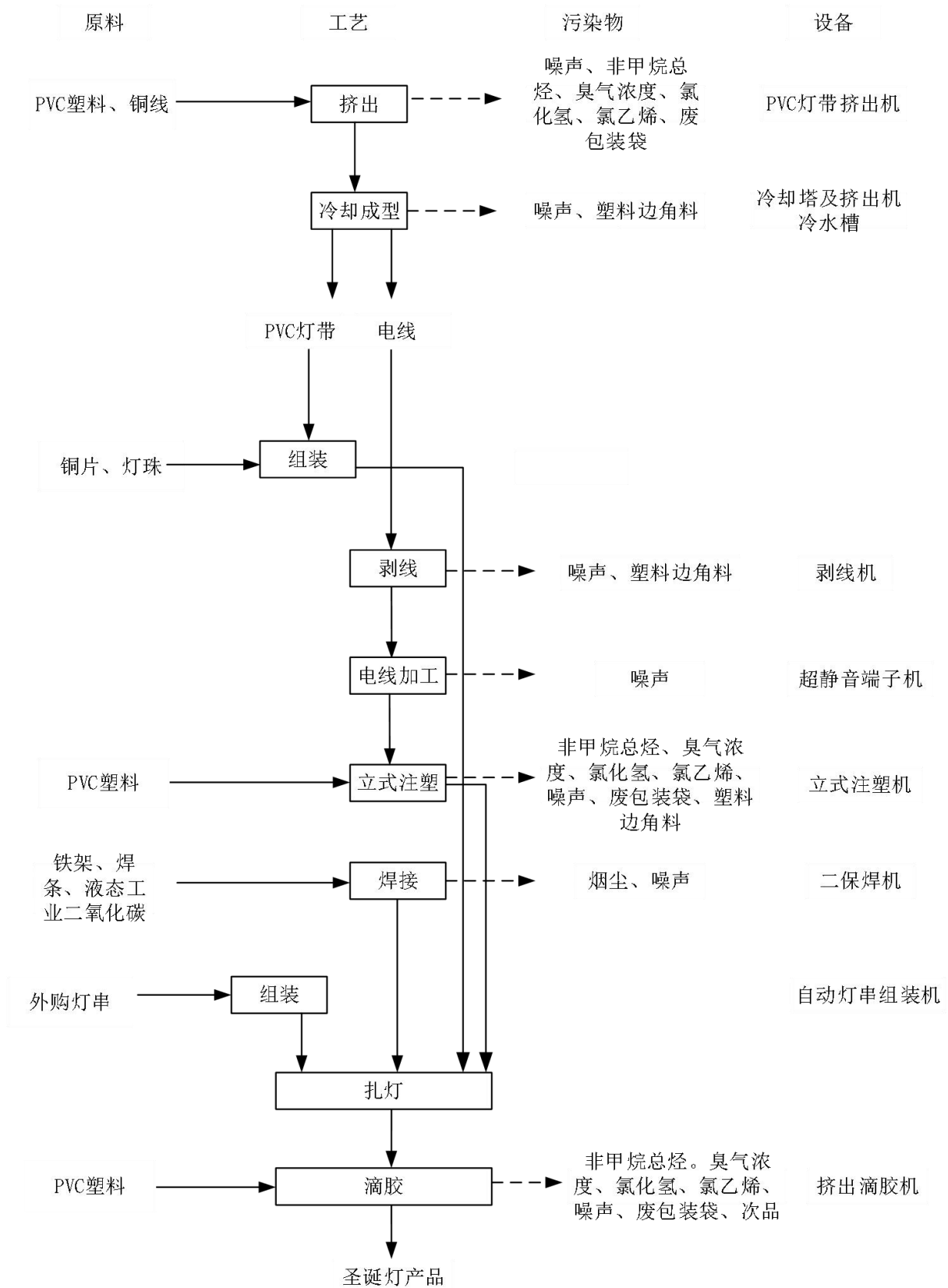
图 2-1 圣诞灯产品生产工艺流程图
