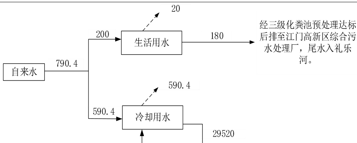
图 2-1 全厂用水平衡图（单位：t/a）
