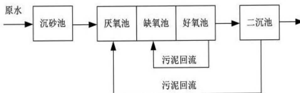
图 4-1 江门高新区综合污水处理厂污水处理工艺
