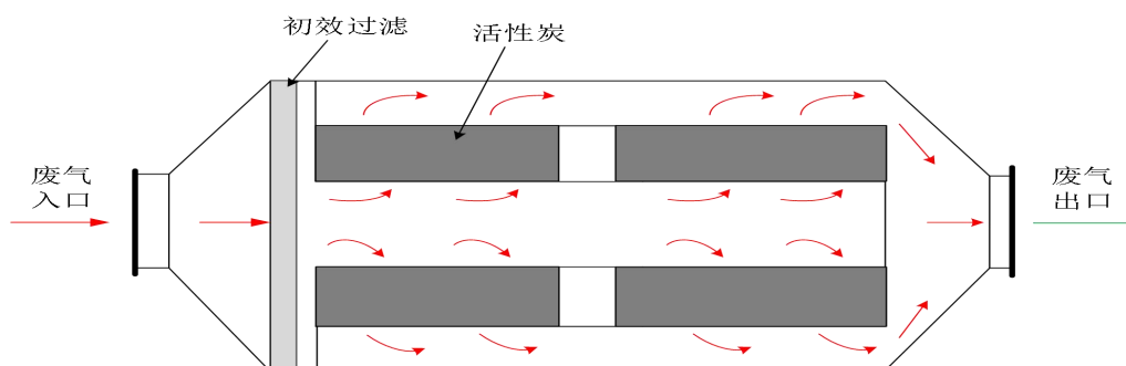
图 4-1 单个活性炭箱内部气体流向示意图
