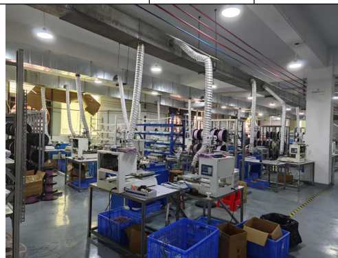
焊线工序收集方式照片
