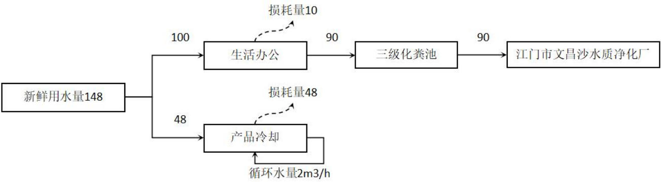
图 2-2 项目水平衡图 (t/a)
