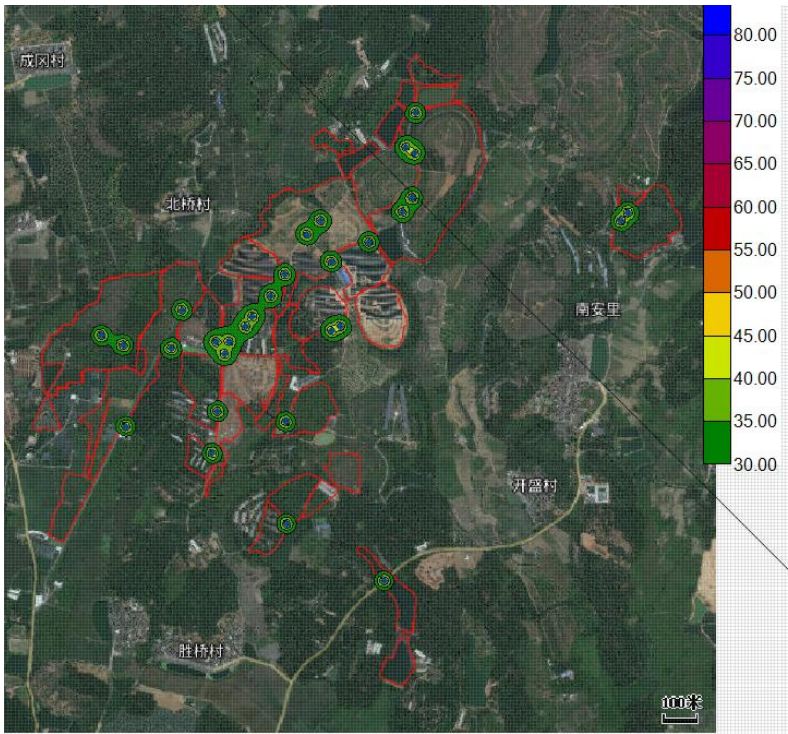
图 4-3 光伏片区声等值线图（地块 1、地块 2、地块 3）
