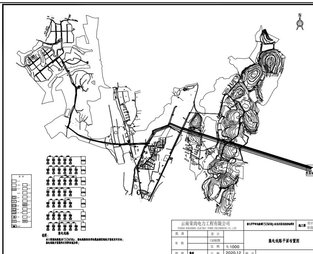
图 2-3 变动前 35kV 电缆集电线路路径
