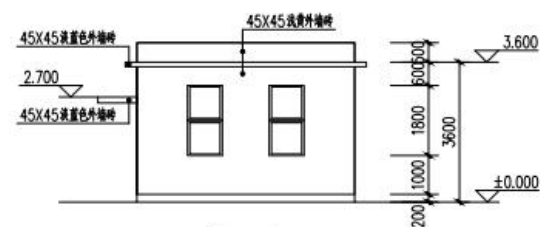
侧立面图 1:100
