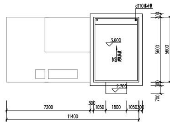
监控室屋顶平面图 1:100
