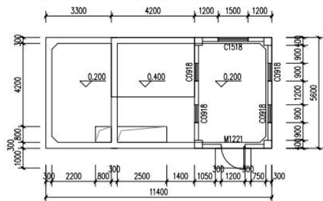
监控室首层平面图 1:100
