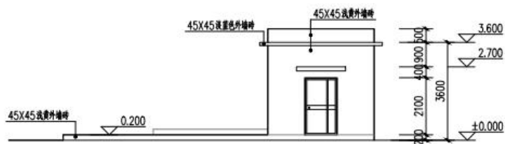
正立面图 1:100
