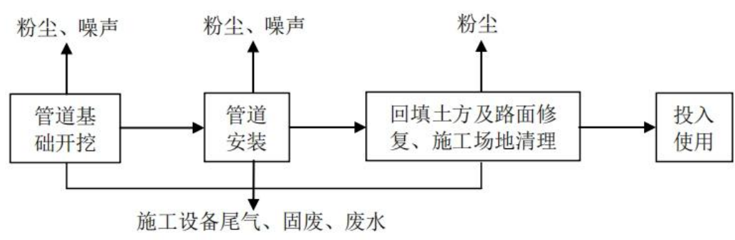
图 2-5 污水管网施工工艺流程及产污节点图（施工期）
