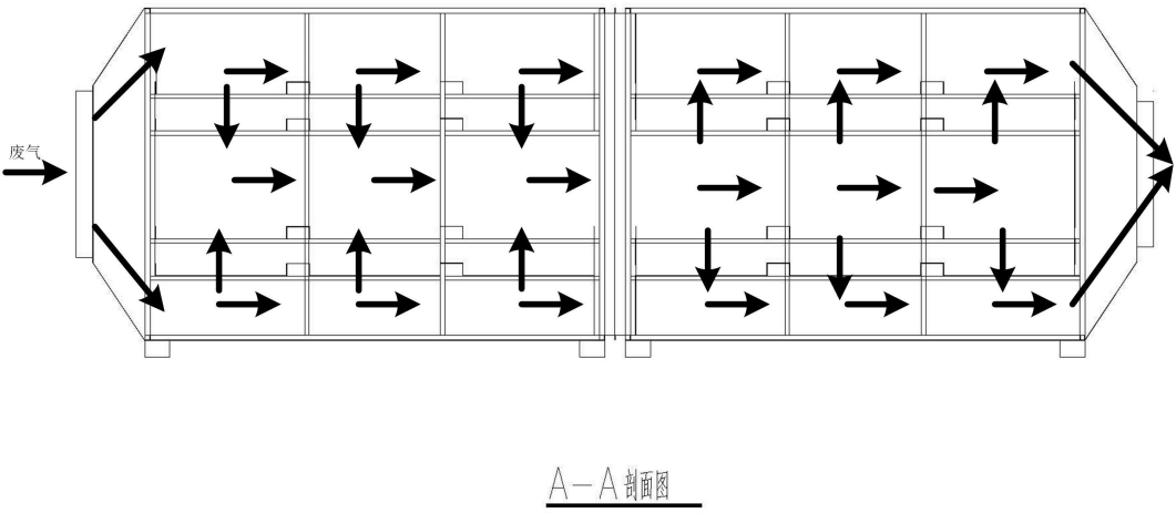
图 4-2 二级活性炭箱设计风道示意图
