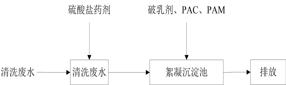
图 4-2 自建废水处理设施处理工艺流程
