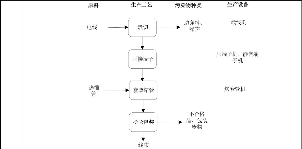
图 2-5 线束生产流程图
