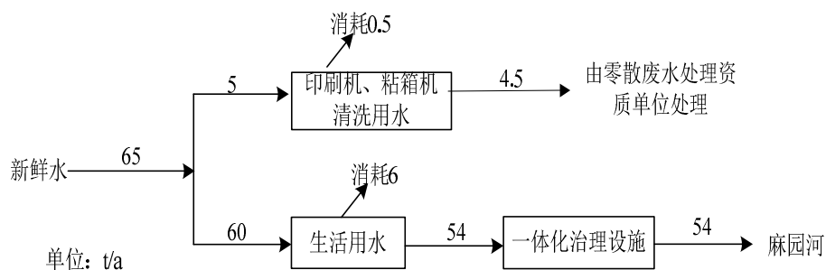
图2-1 水平衡图
