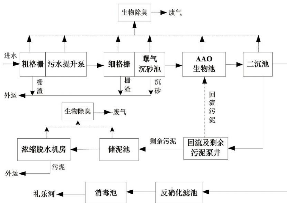
图 12. 江门高新综合污水处理厂废水处理工艺流程图
