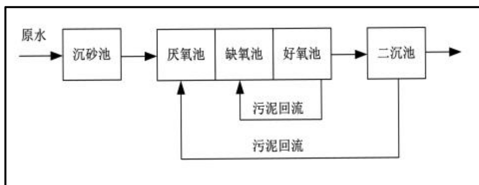
图 4-1 江海（高新）污水处理厂处理工艺流程
