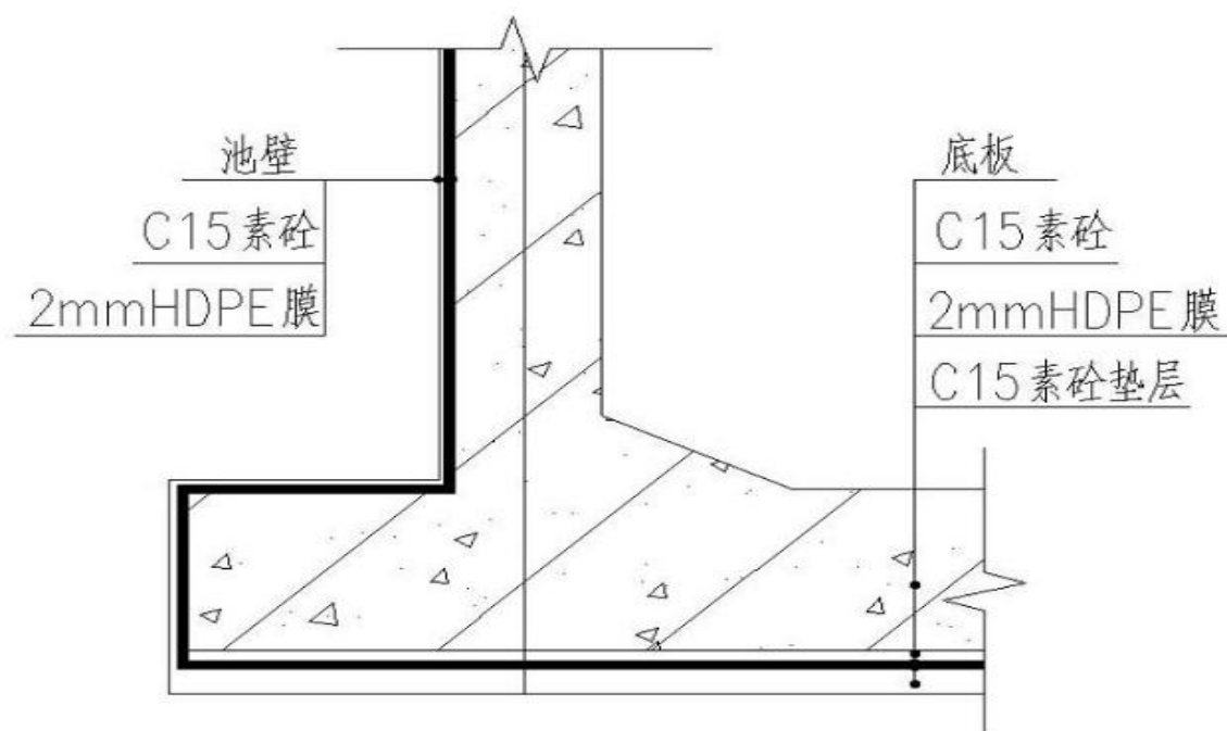
图 5-1 事故油池池底池壁防渗结构
