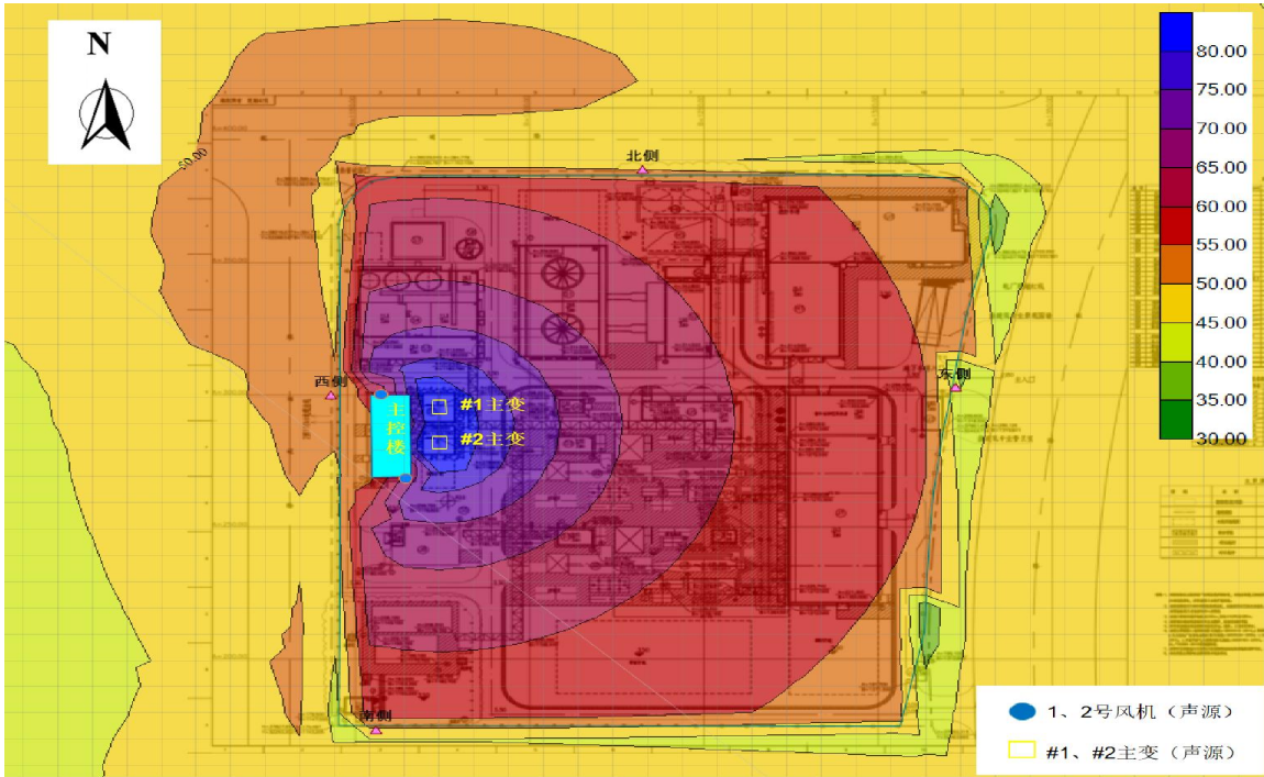
图 4-1 噪声贡献值等值线图
