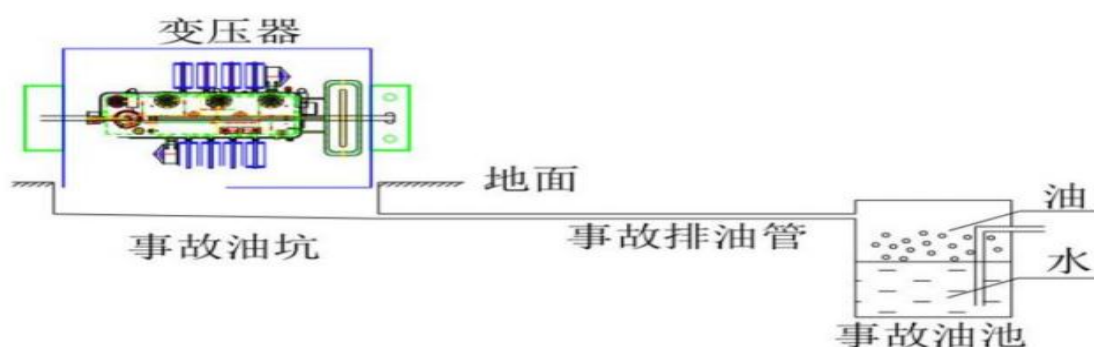
图 4-2 本项目事故排油示意图
