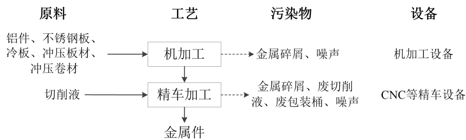
图 2-3 金属件件工艺流程图
