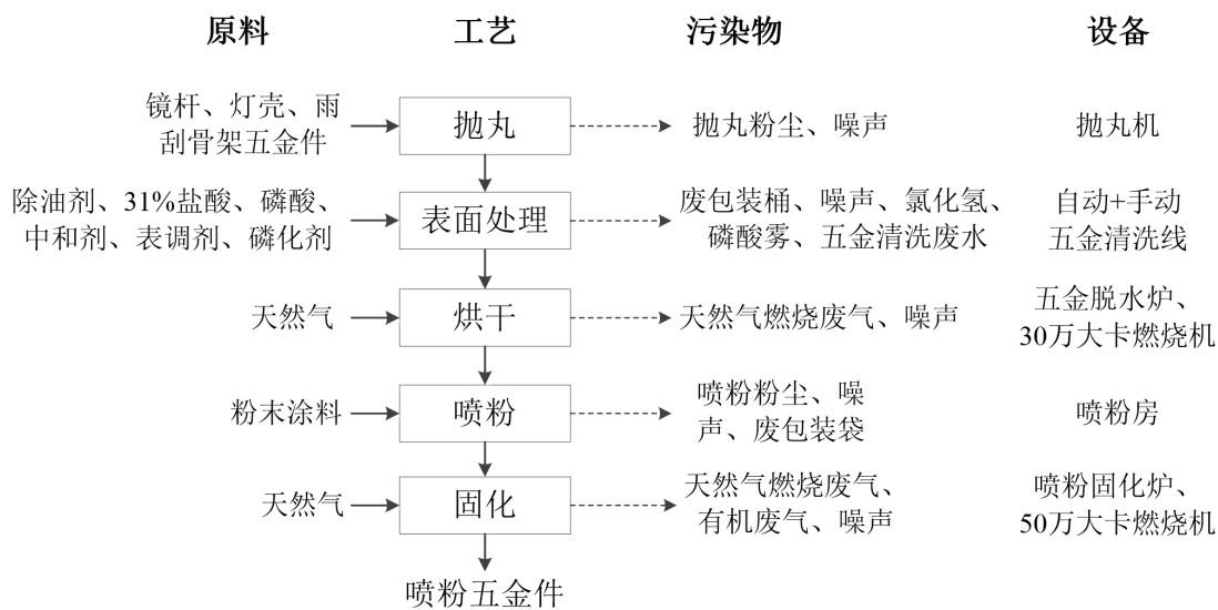
图 2-4 喷粉五金件工艺流程图
