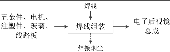
图 2-10 电子后视镜总成工艺流程图
