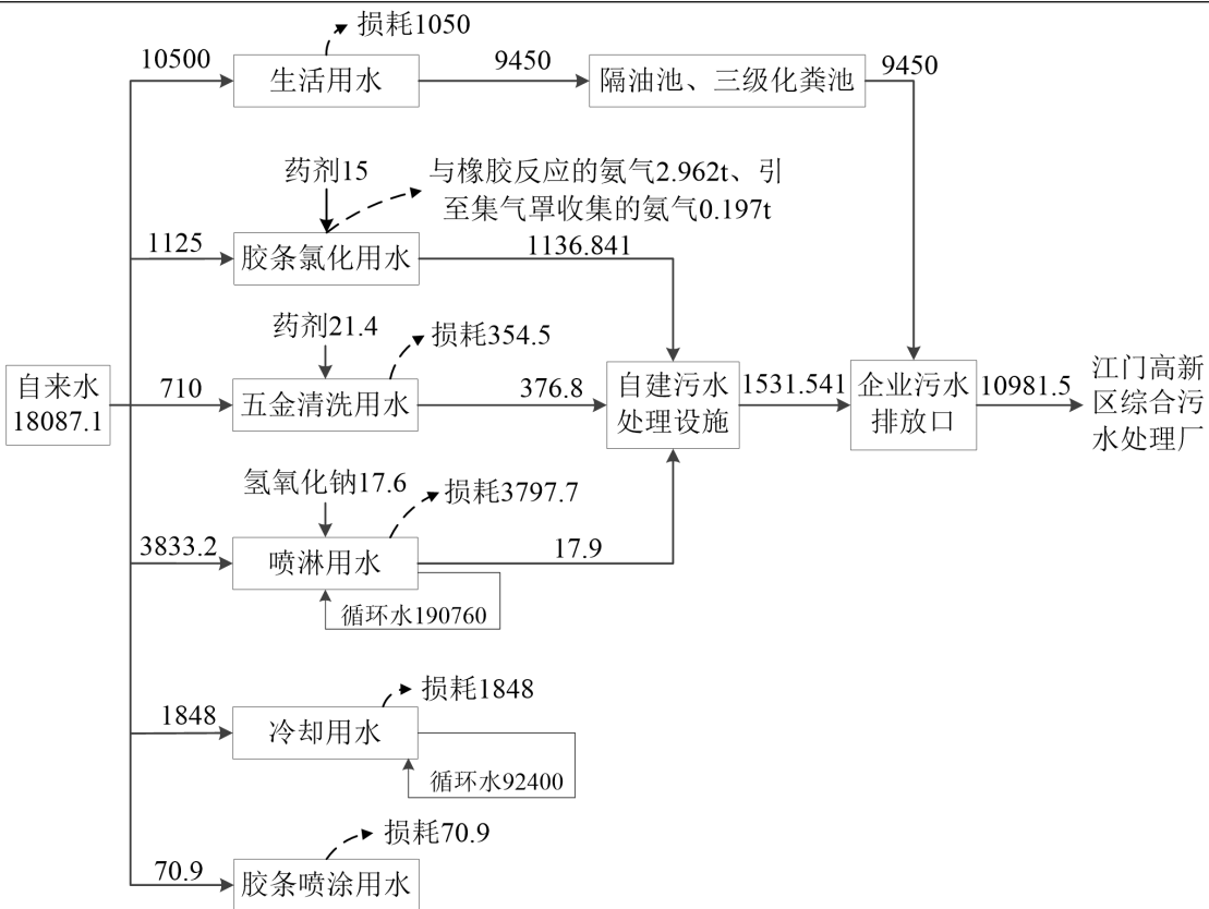
图 2-1 本项目全厂用水平衡图（单位：t/a）
