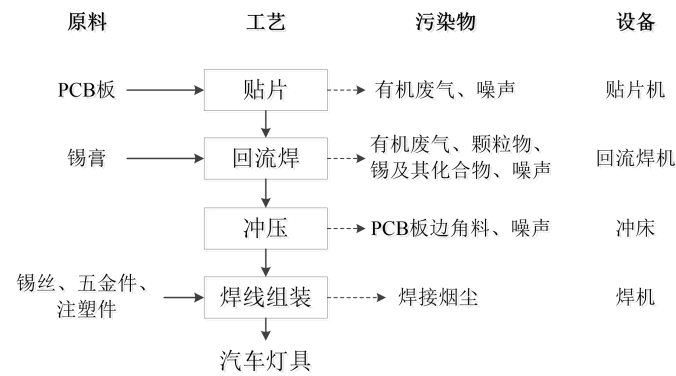
图 2-7 汽车灯具工艺流程图
