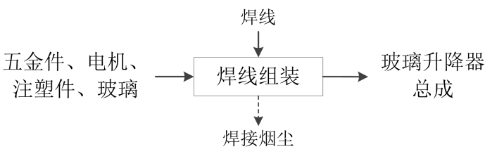
图 2-11 玻璃升降器总成工艺流程图
