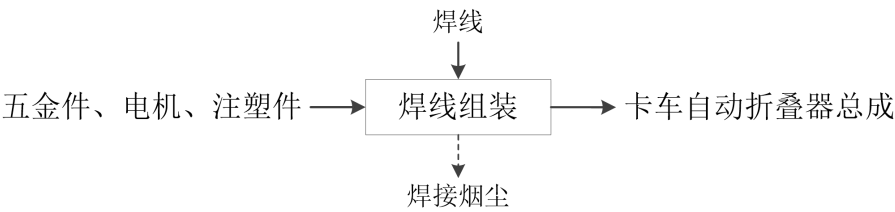
图 2-8 卡车自动折叠器总成工艺流程图
