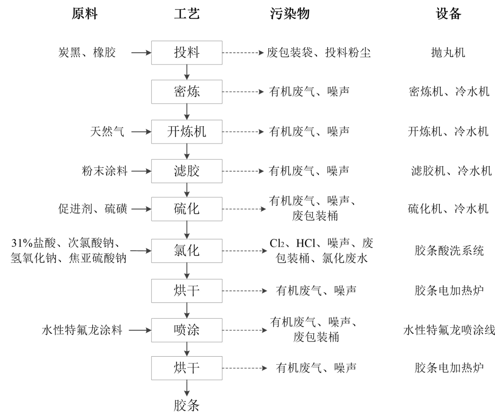
图 2-5 胶条工艺流程图
