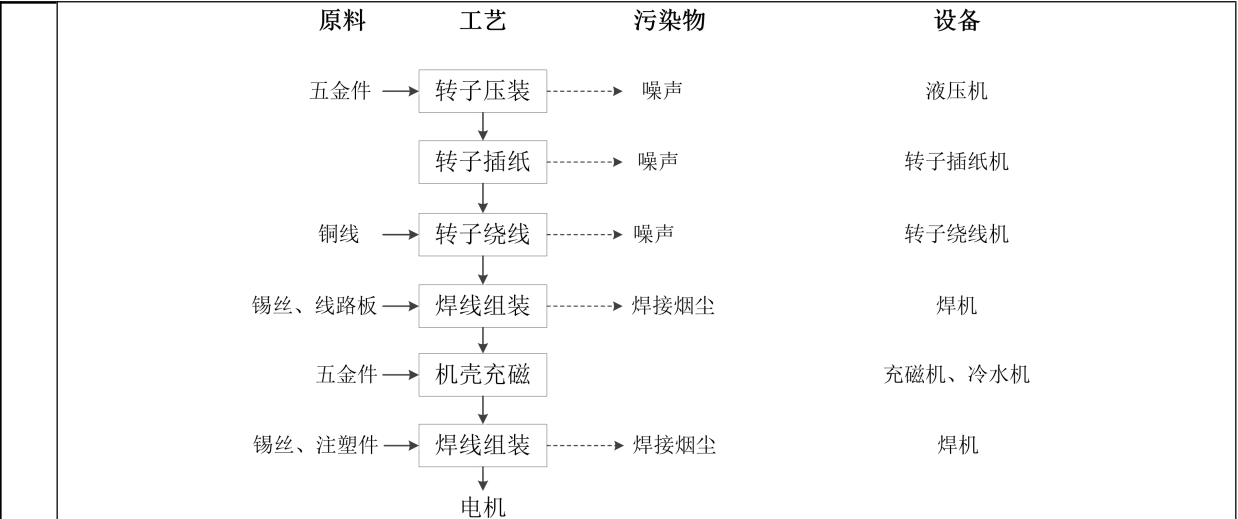
图 2-7 汽车电机工艺流程图
