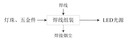
图 2-6 汽车 LED 光源工艺流程图
