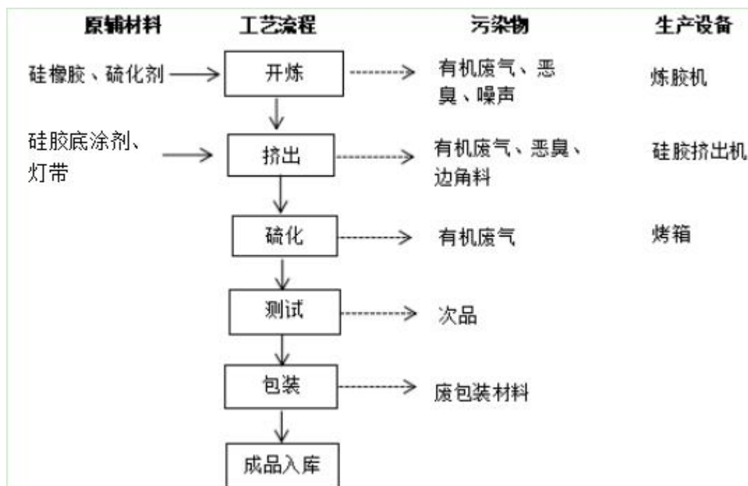
图 2-2 项目硅胶灯带生产工艺流程图
