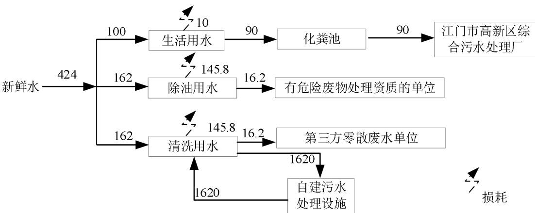
图 1. 扩建项目水平衡图 (t/a)
