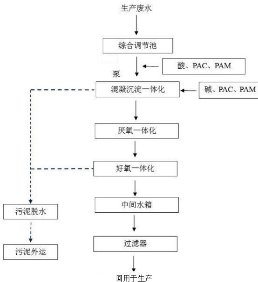
图 5. 废水处理工艺图
