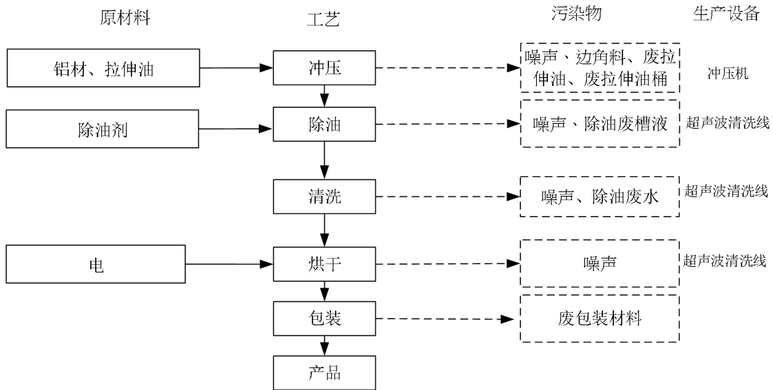
图 3. 生产工艺流程图
