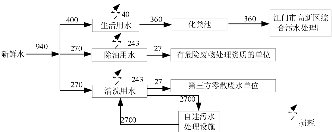
图 2. 扩建后全厂水平衡图 (t/a)
