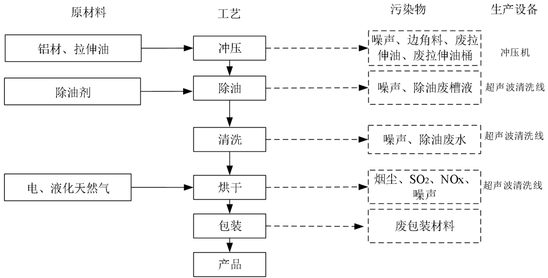
图 4. 生产工艺流程图
