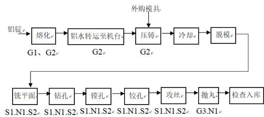
图 2-7 原有项目摩托车发动机外壳工艺流程
