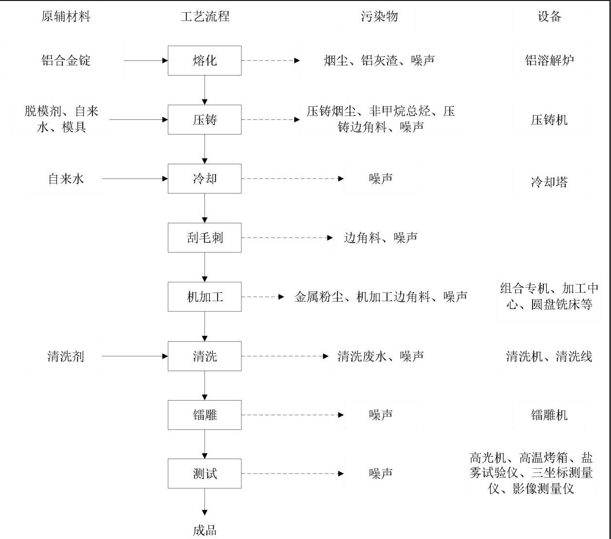
图 2-5 铝合金消费电子类配件生产工艺流程及产污环节图
