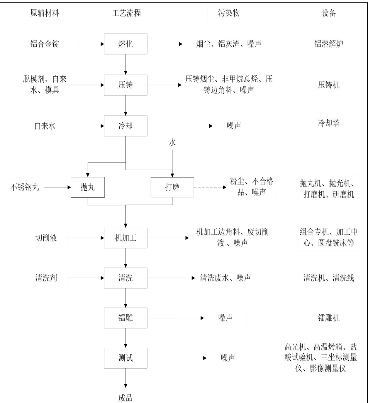
图 2-4 摩配类配件、腔体类配件、芯体类配件生产工艺流程（二）及产污环节图 工艺流程说明：
