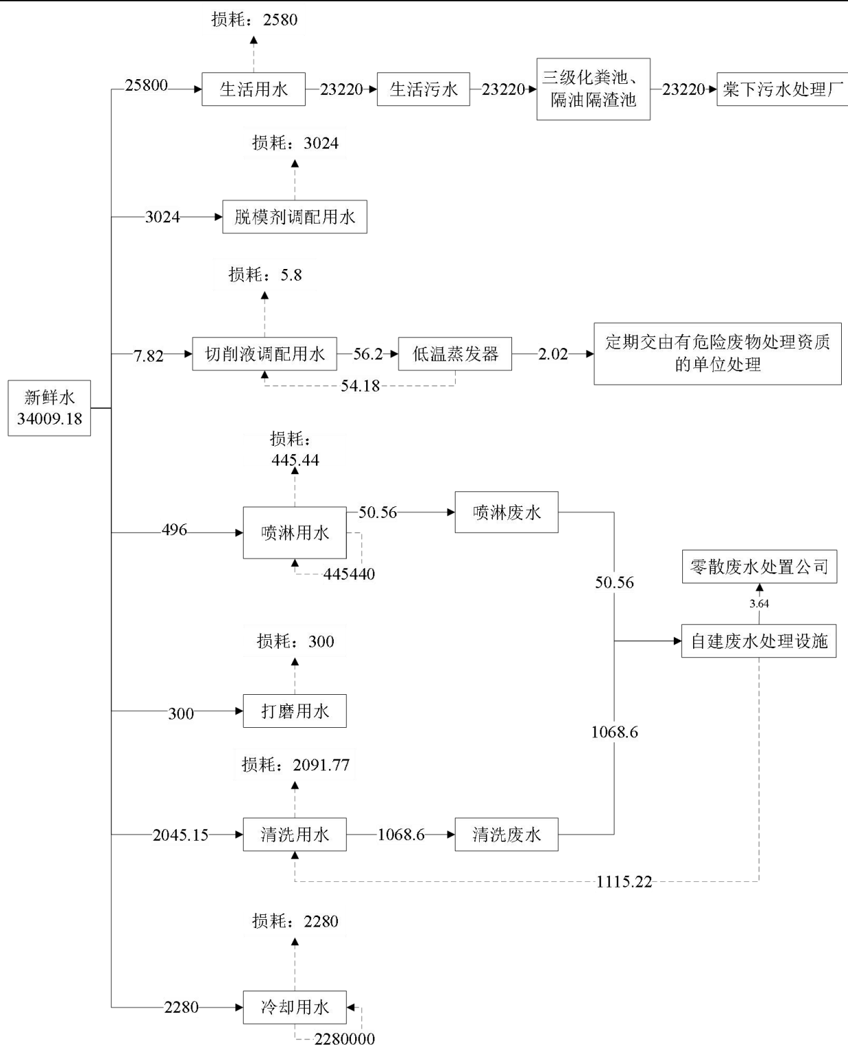
图 2-2 改扩建后项目水平衡图
