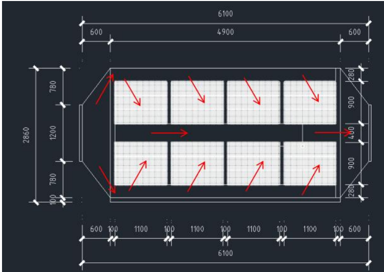
图 4-1 活性炭箱风道示意图
