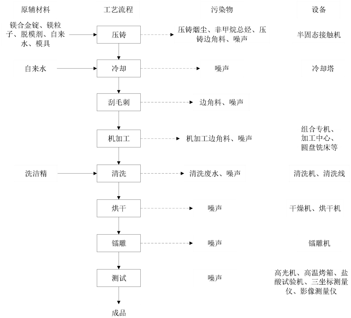
图 2-5 镁合金消费电子类配件生产工艺流程及产污环节图 工艺流程说明：
