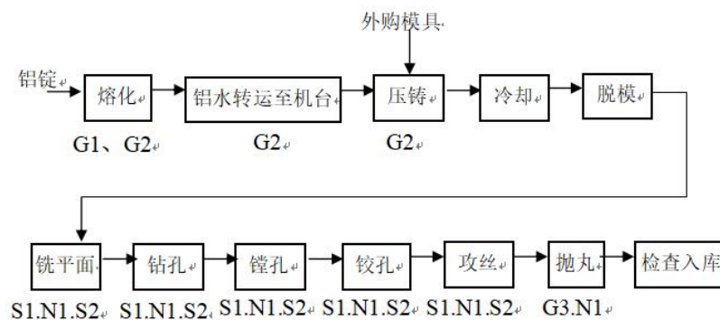
图 2-7 原有项目镁合金制品工艺流程
