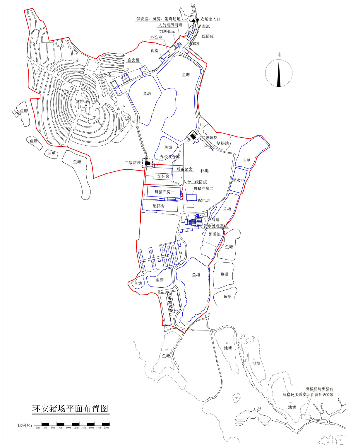
图 2.2-1a 现有项目总平面布置图
