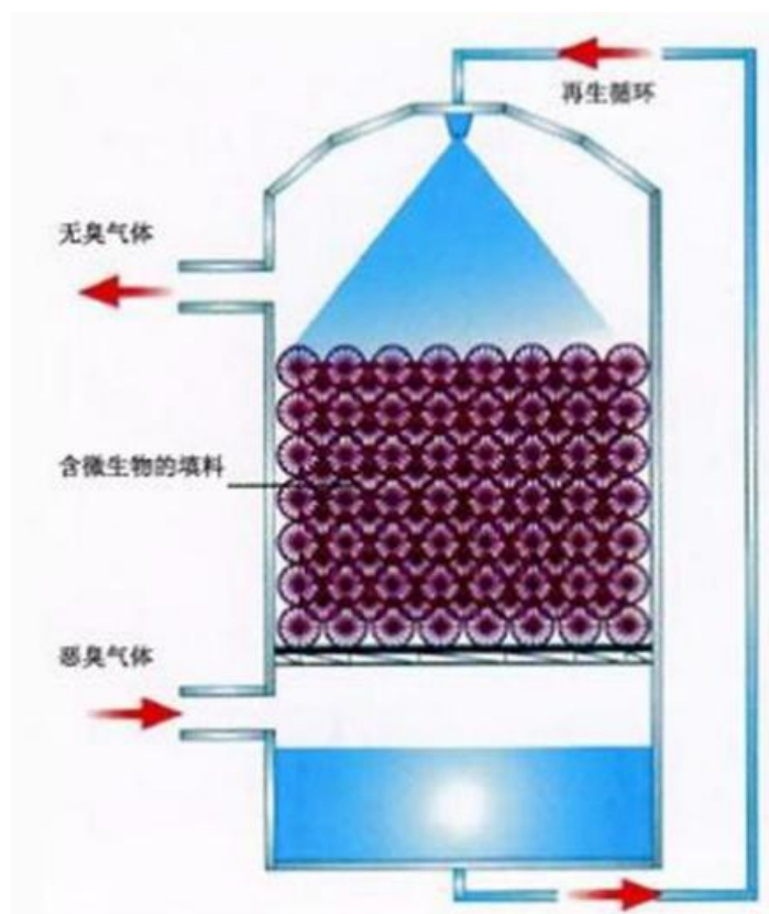
图 7.1-2 喷淋除臭原理图
