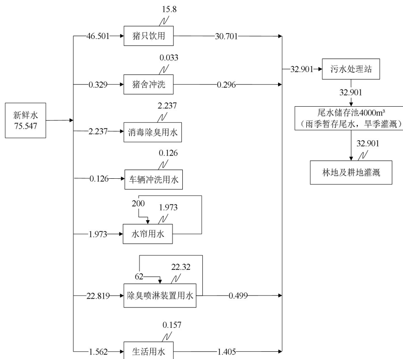
图 3.4-1 本项目水平衡图 单位：m 3 /d
