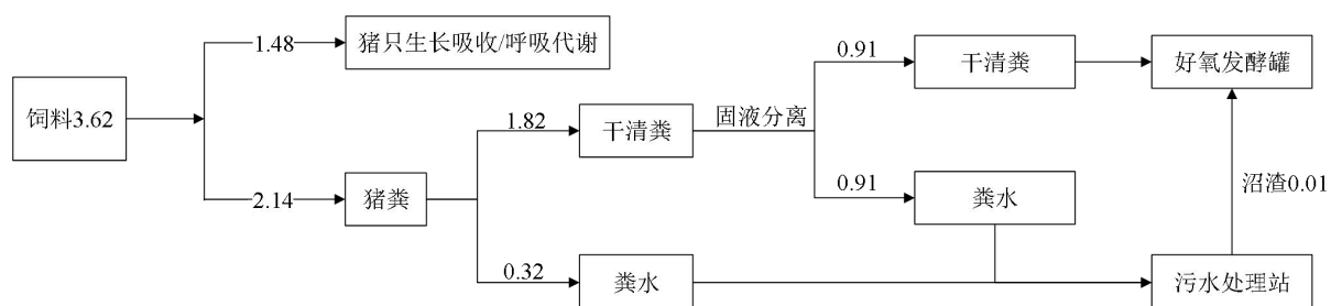
图 2.4-1 现有项目物料平衡图 单位：t/d
