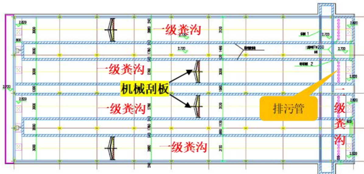
图 3.3-2 育肥舍粪沟分布示意图
