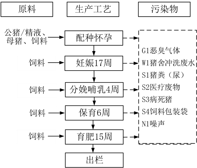
图 3.3-5 本项目总工艺流程图
