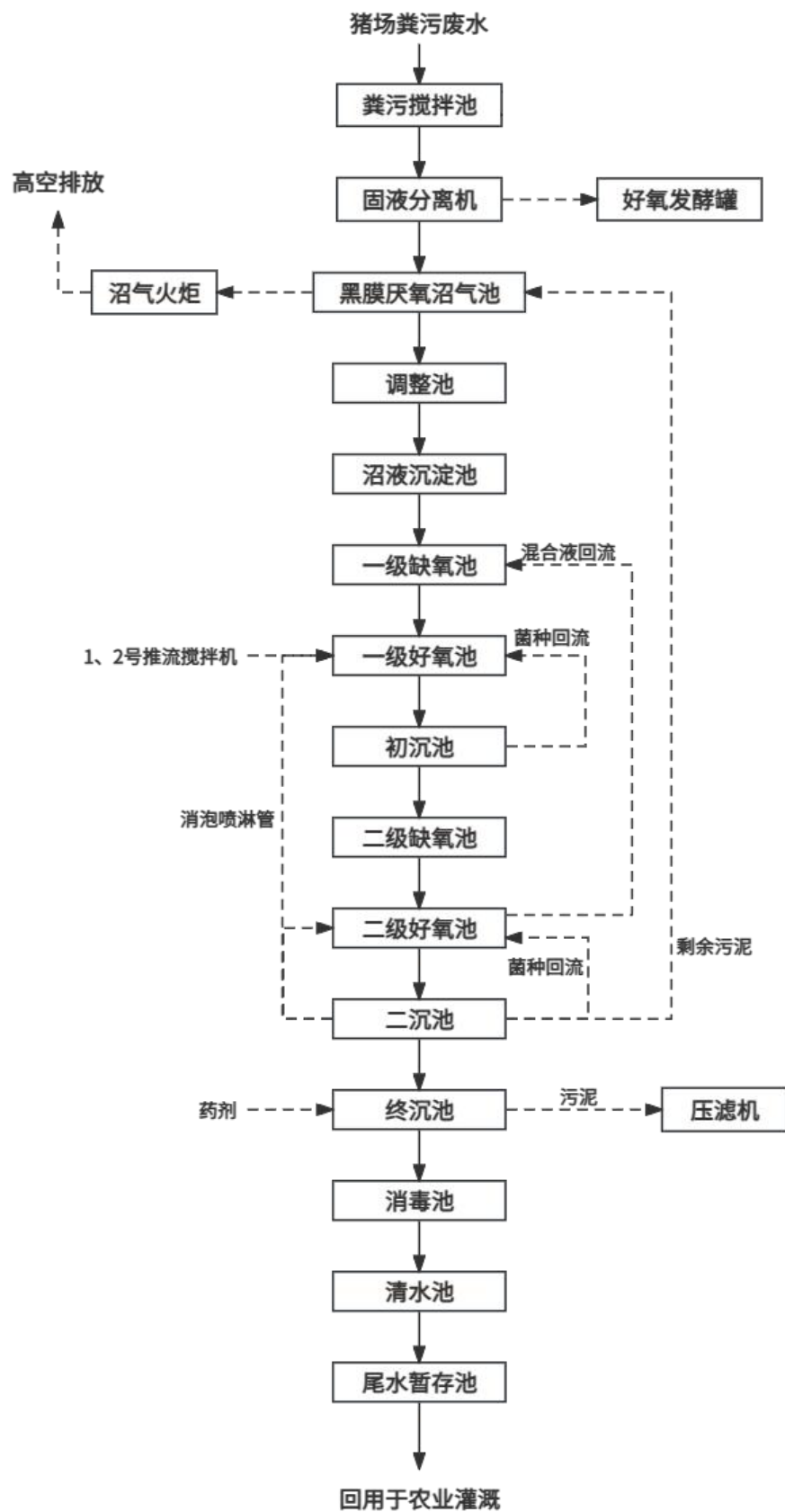
图 7.2-1 废水处理工艺流程图
