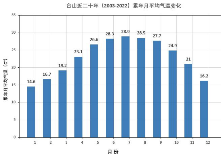
图 6.1-4 台山市（2003-2022）各月平均温度变化曲线图
