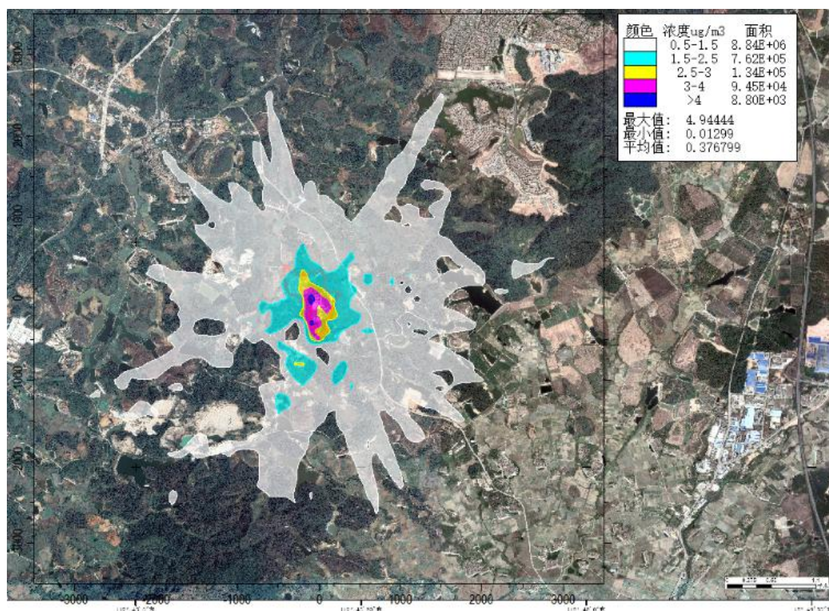
图 6.1-24 硫化氢最大 1h 贡献浓度分布图（非正常工况）
