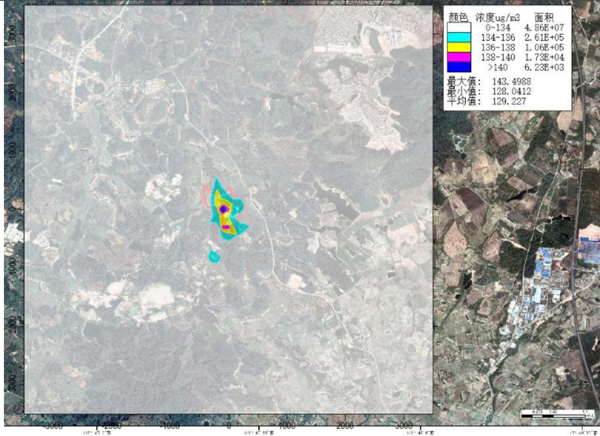
图 6.1-21 叠加后氨 1 小时浓度分布图
