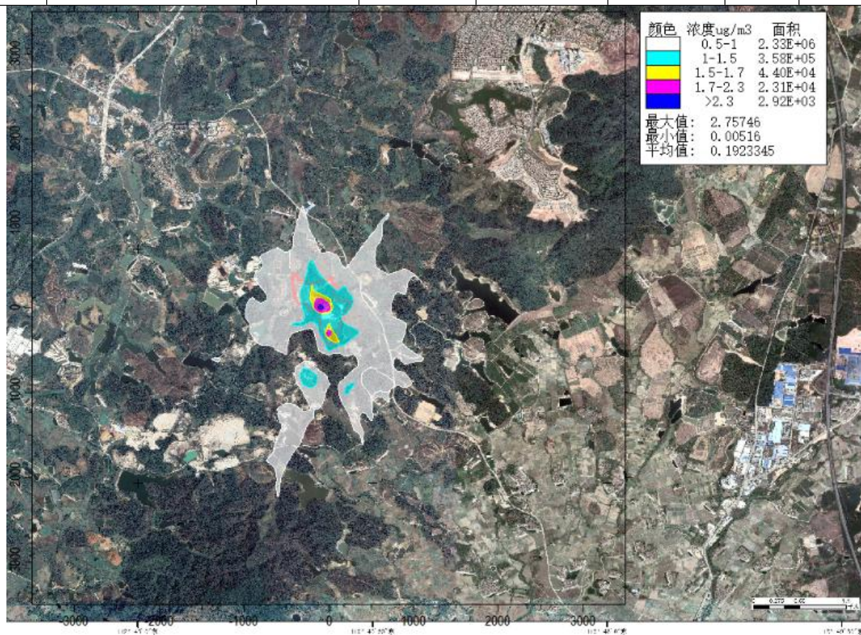
图 6.1-16 硫化氢新增污染源最大 1 小时均值浓度分布
