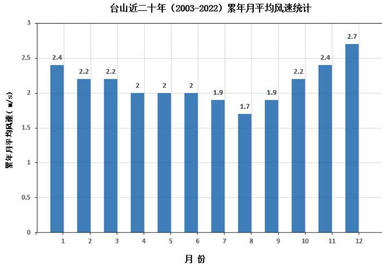
图 6.1-2 台山市近 20 年各月平均风速变化曲线图
