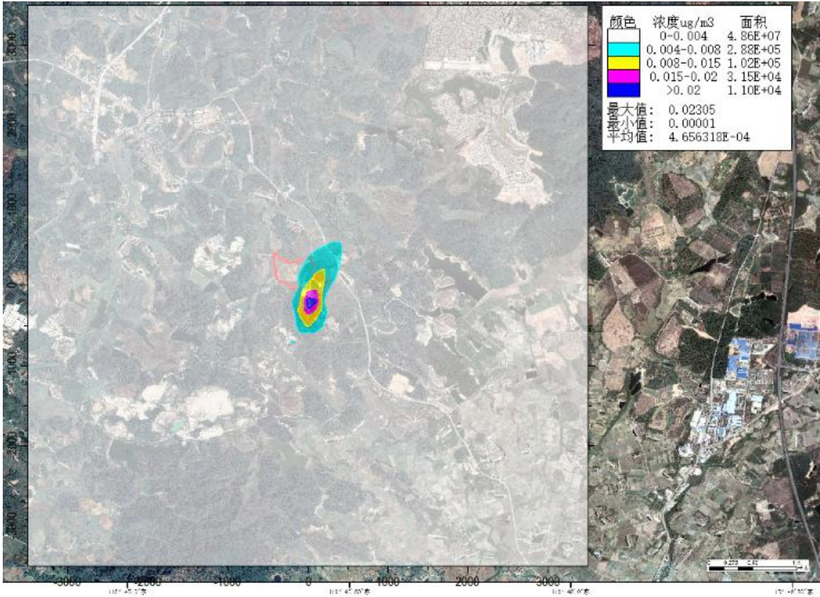
图 6.1-14b PM 2.5 新增污染源最大年均值浓度分布图
