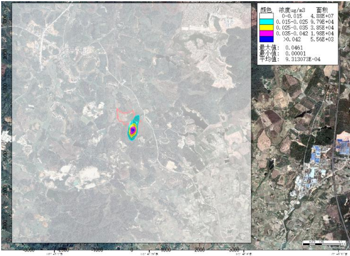
图 6.1-13b \text{PM}_{10} 新增污染源最大年均值浓度分布图
