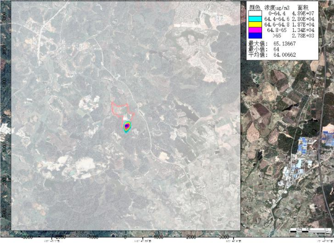
图 6.1-18a 叠加后 NO 2 98%保证率日平均最大落地浓度分布图
