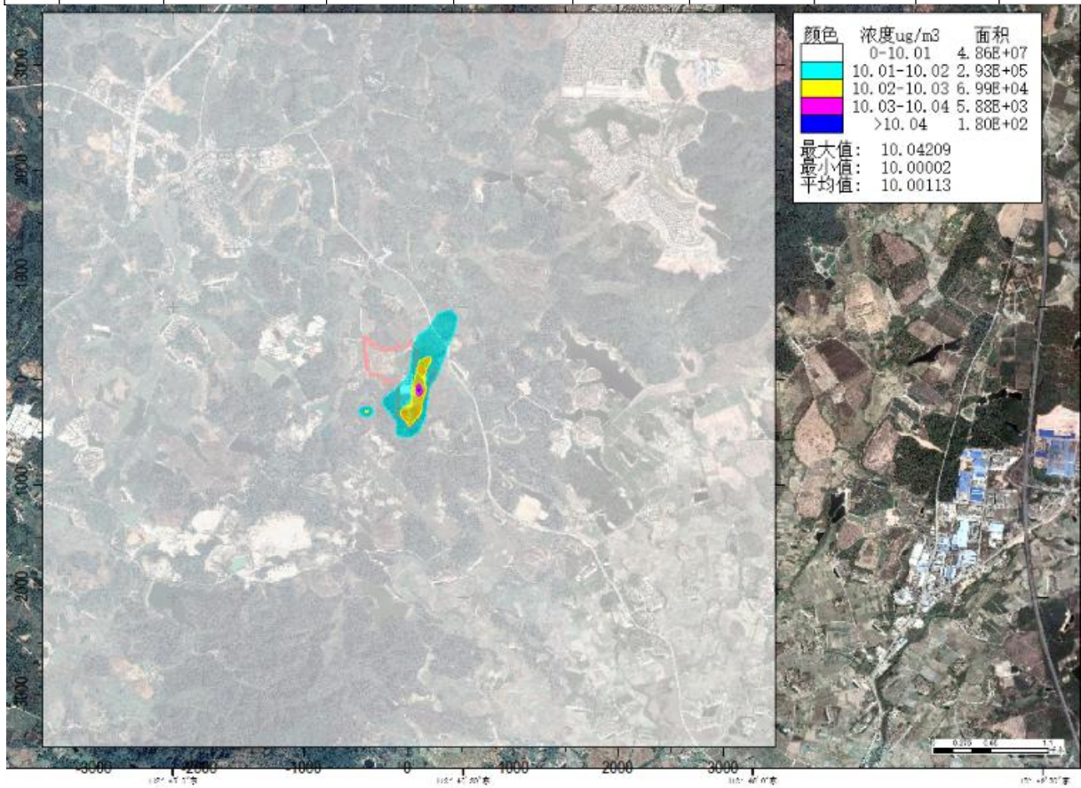
图 6.1-17a 叠加后 SO 2 98%保证率日平均最大落地浓度分布图
