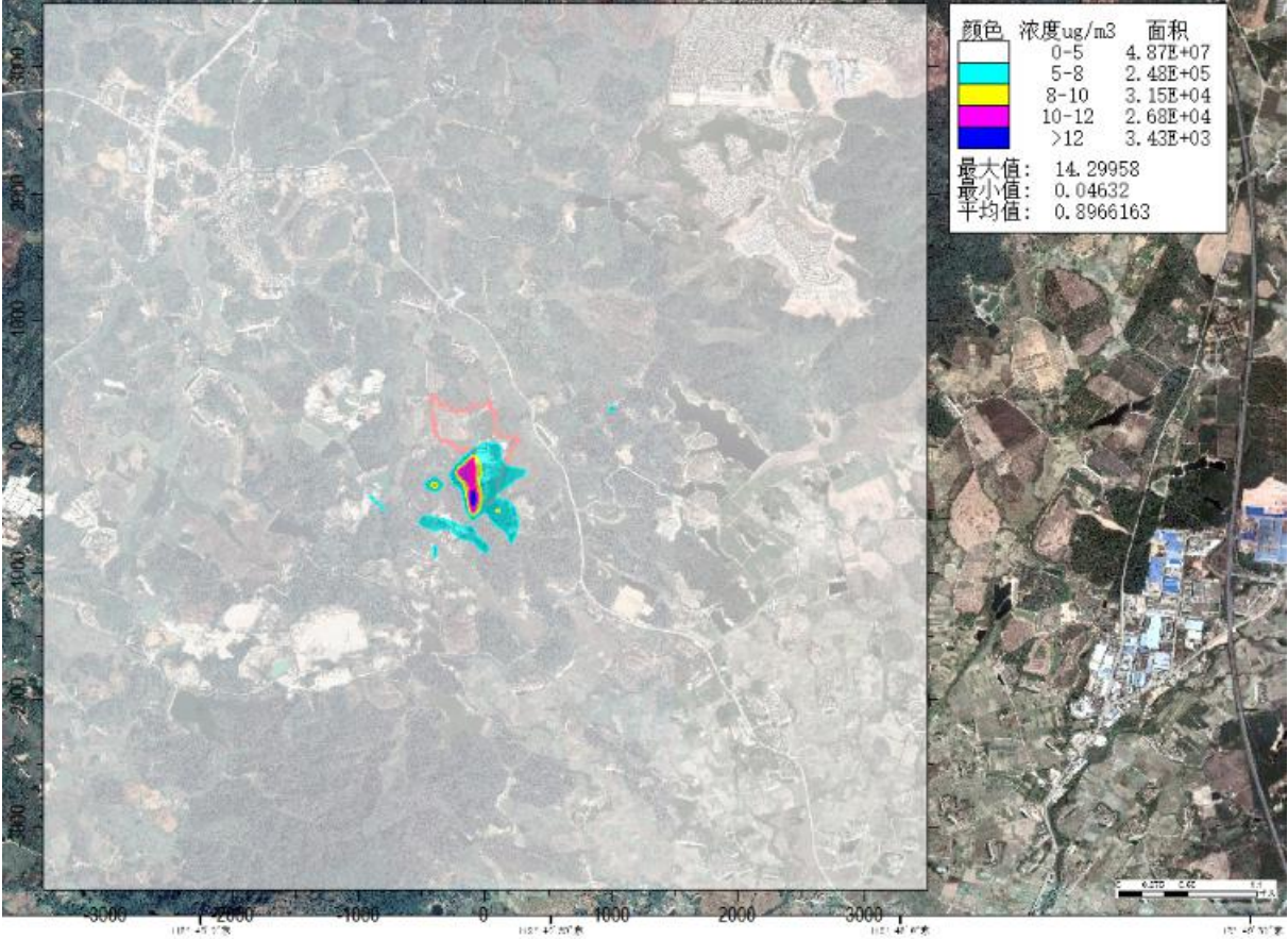
图 6.1-12a NO 2 新增污染源最大 1 小时均值浓度分布图
