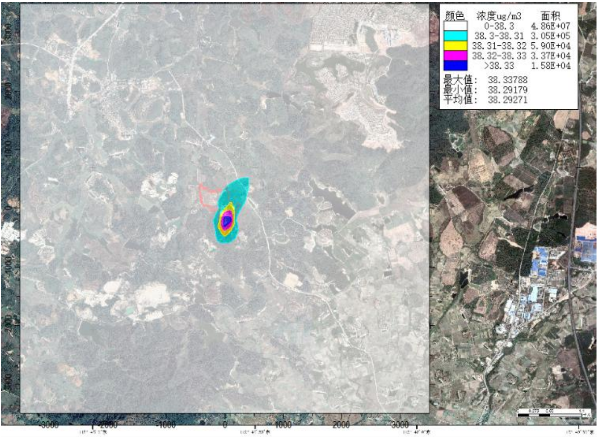
图 6.1-19b 叠加后 PM 10 年平均最大落地浓度分布图
