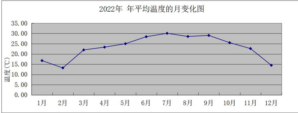
图 6.1-6 台山市 2022 年各月平均温度变化曲线图
