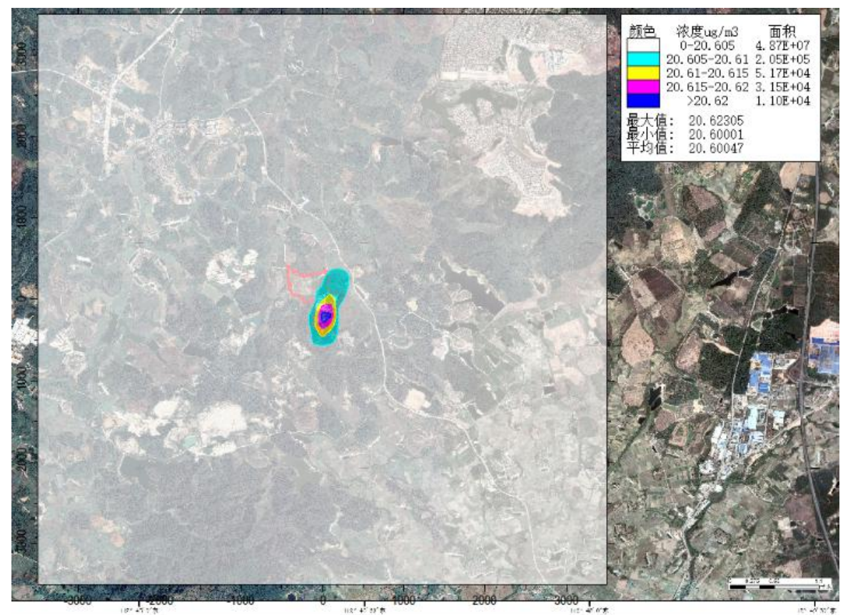
图 6.2-20b 叠加后 PM 2.5 年平均最大落地浓度分布图
