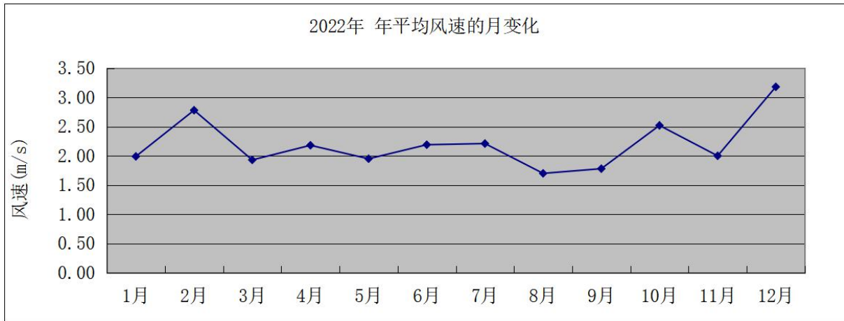
图 6.1-7 台山市 2022 年各月平均风速变化曲线图
