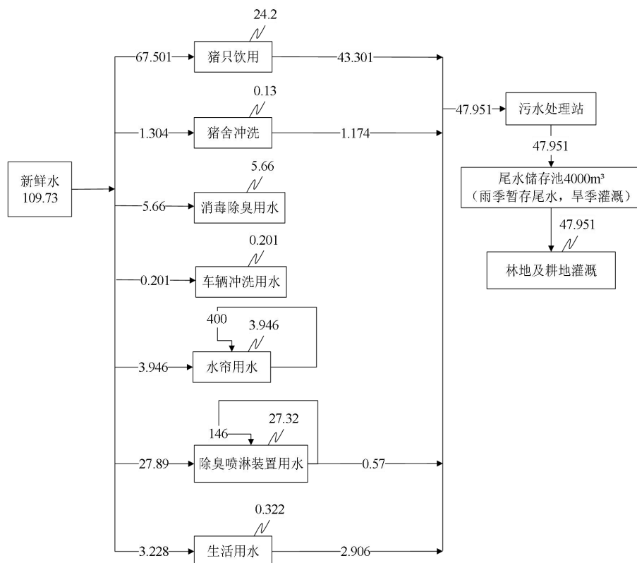
图 3.4-2 本项目建设完成后全场水平衡图 单位：m³/d
