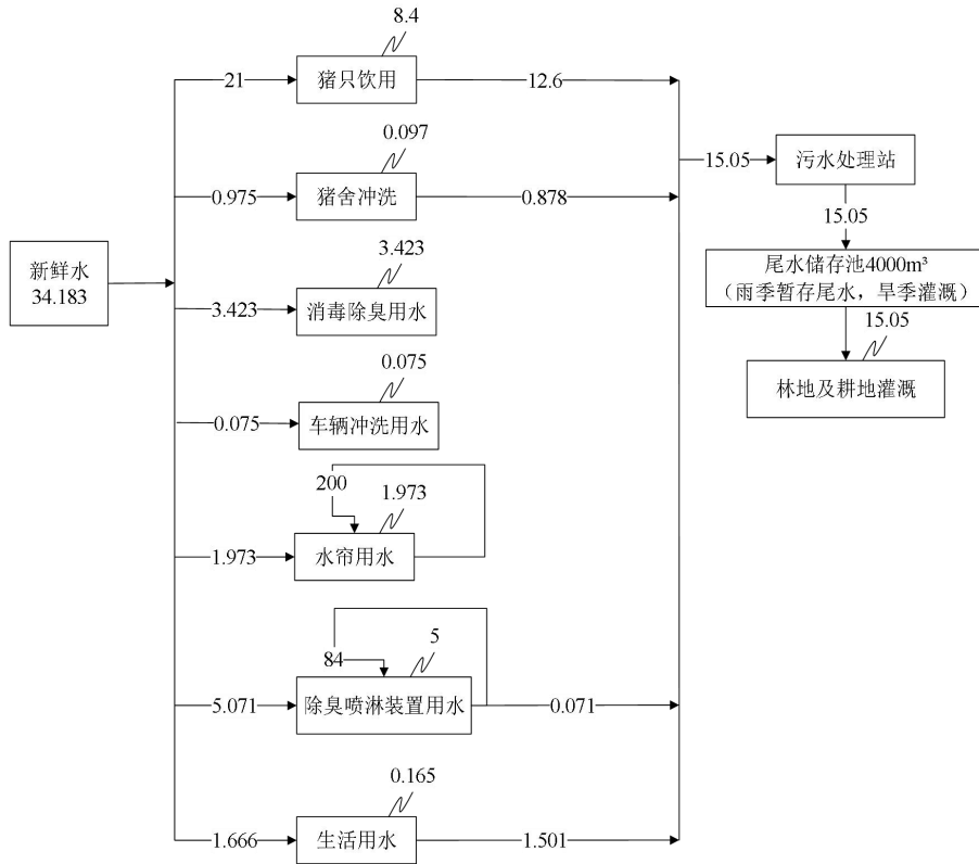
图 2.4-2 现有项目水平衡图 单位：m³/d
