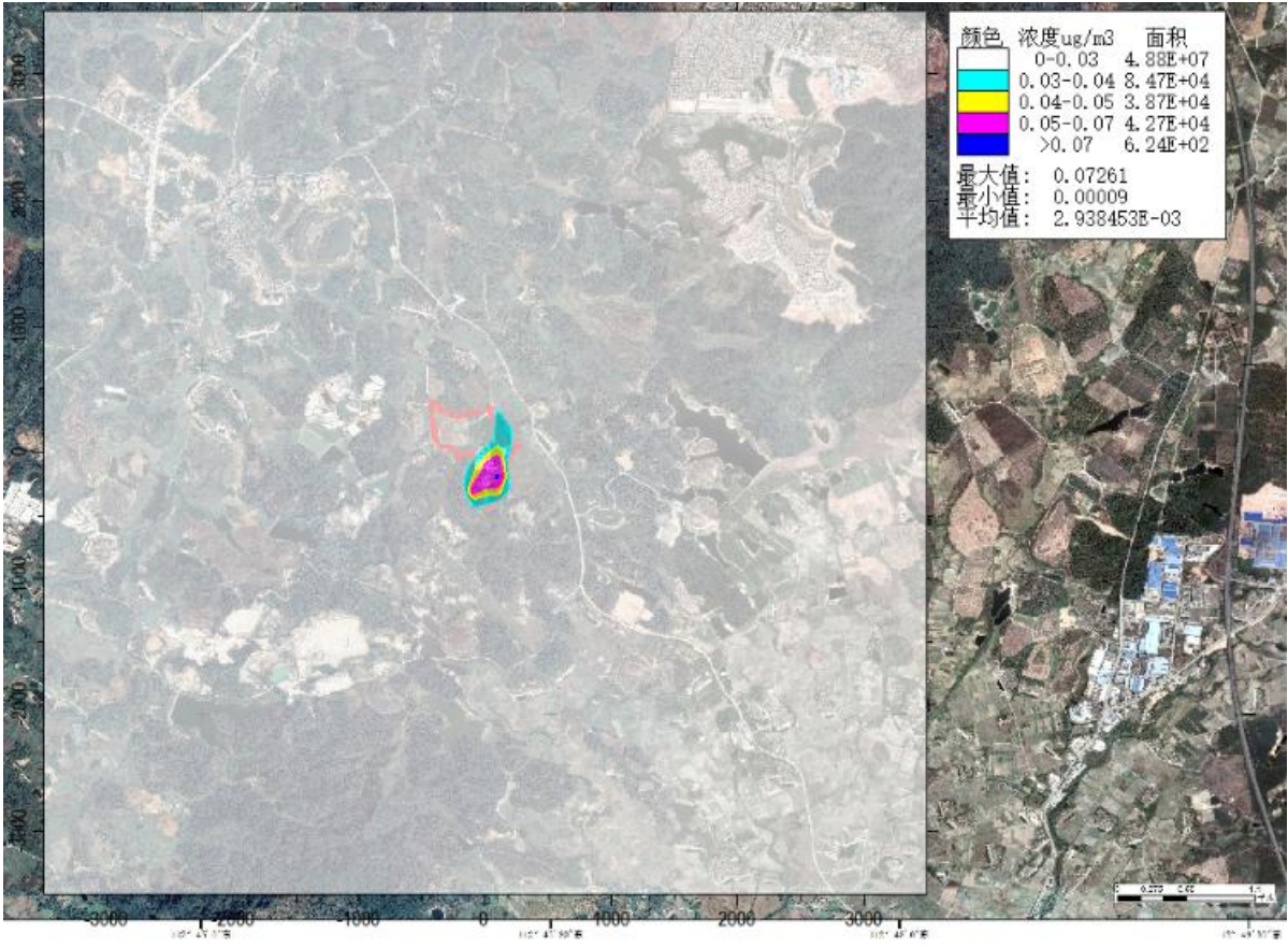
图 6.1-11b SO 2 新增污染源最大日均值浓度分布图
