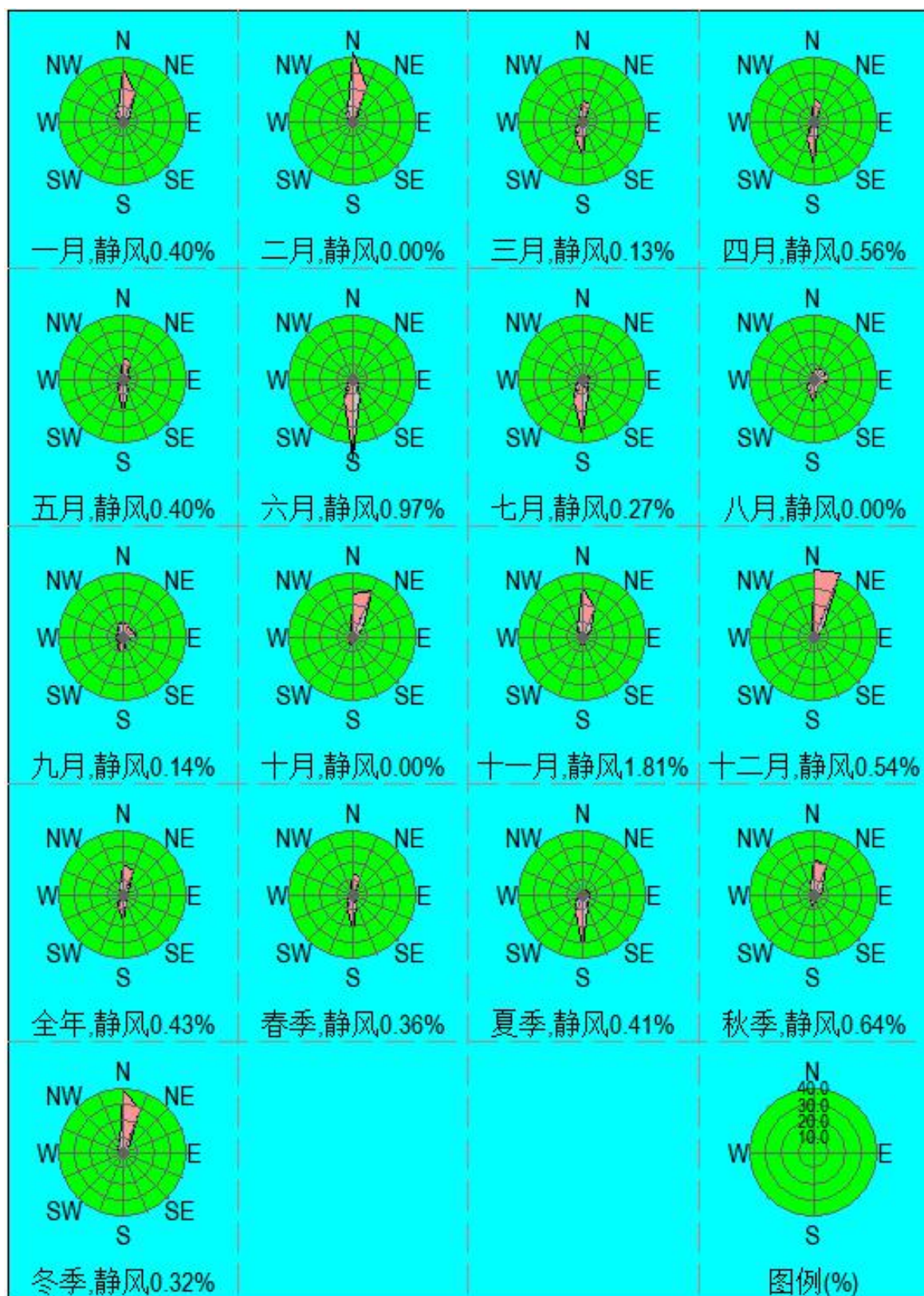
图 6.1-8 台山市 2022 年地面风向玫瑰图
