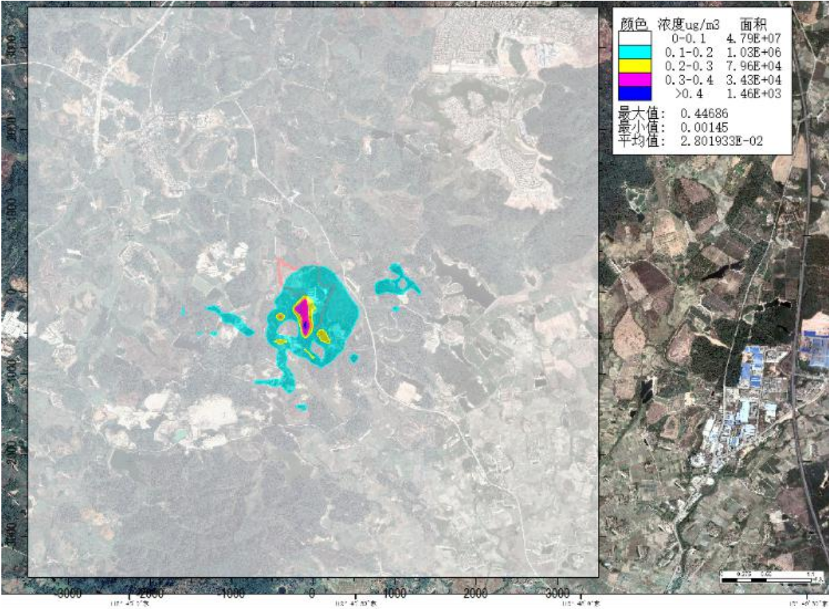
图 6.1-11a SO 2 新增污染源最大 1 小时均值浓度分布图
