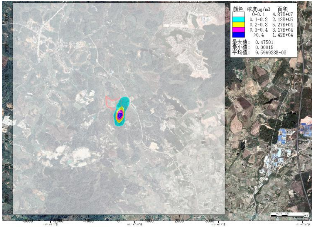
图 6.1-12c NO 2 新增污染源最大年均值浓度分布图
