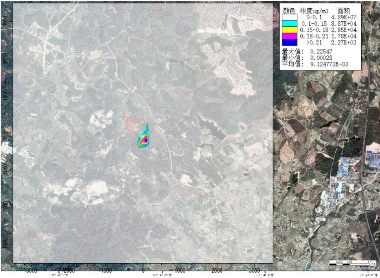
图 6.1-13a \text{PM}_{10} 新增污染源最大日均值浓度分布图
