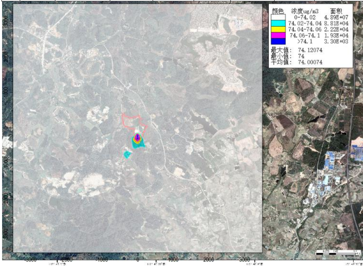
图 6.1-19a 叠加后 \text{PM}_{10} 95%保证率日平均最大落地浓度分布图
