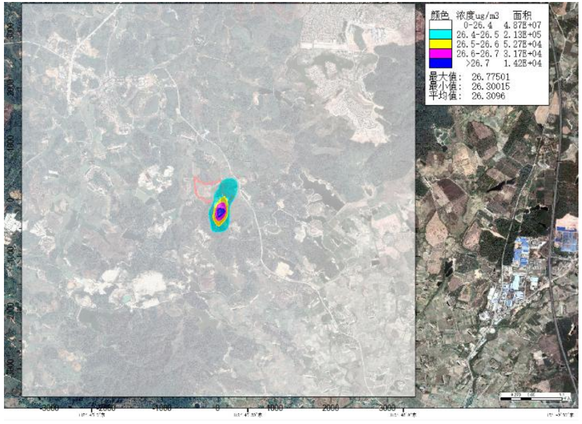
图 6.1-18b 叠加后 NO 2 年平均最大落地浓度分布图
