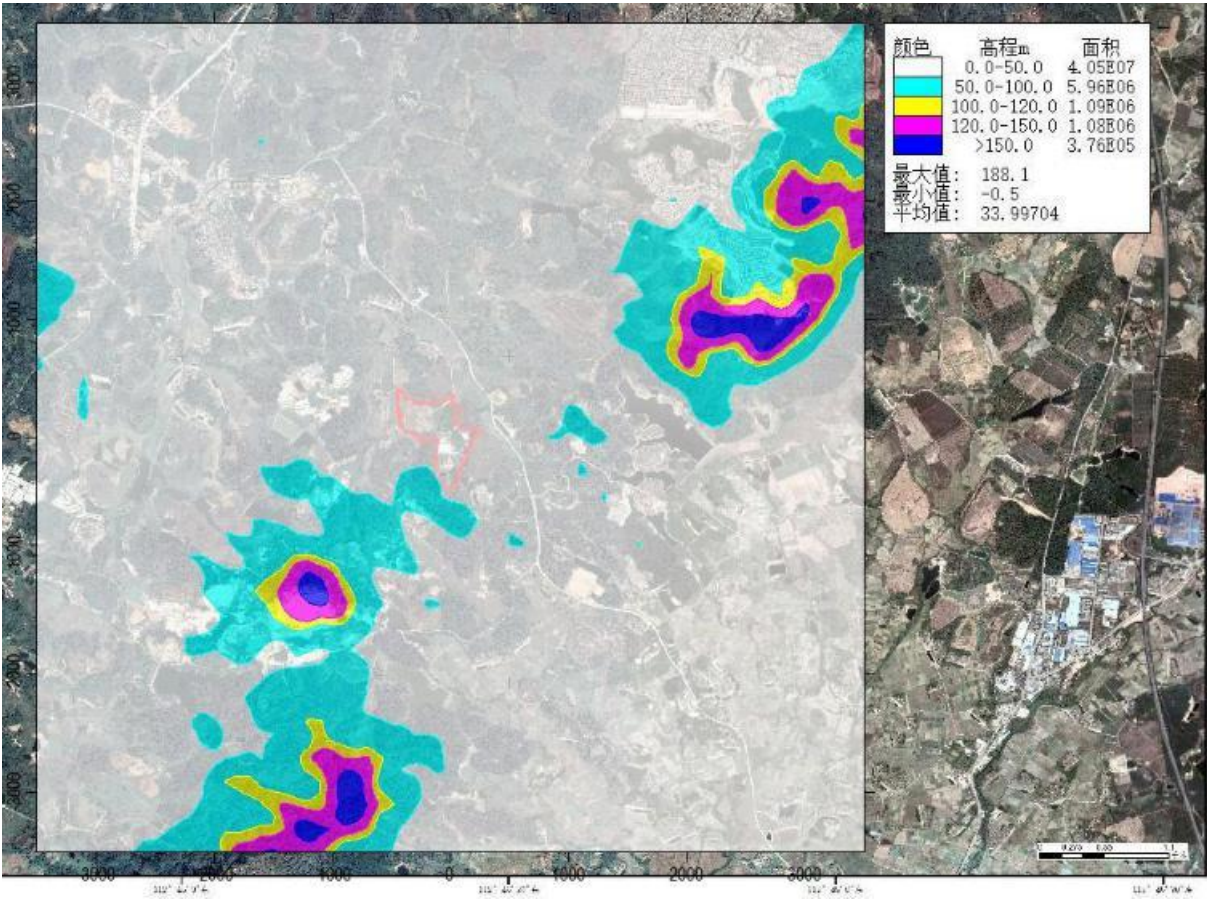
图 6.1-10 本项目大气预测范围地形等高线图
