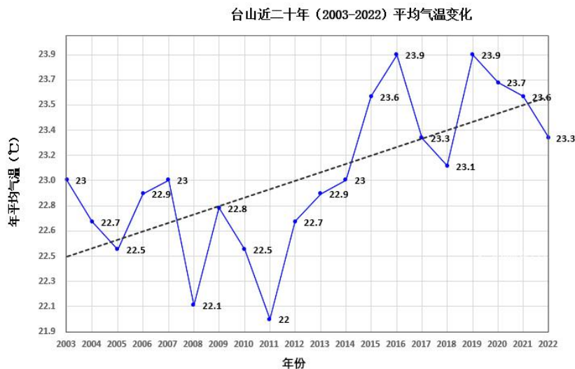
图 6.1-5 台山市（2003-2022）年平均气温（虚线为趋势线）
