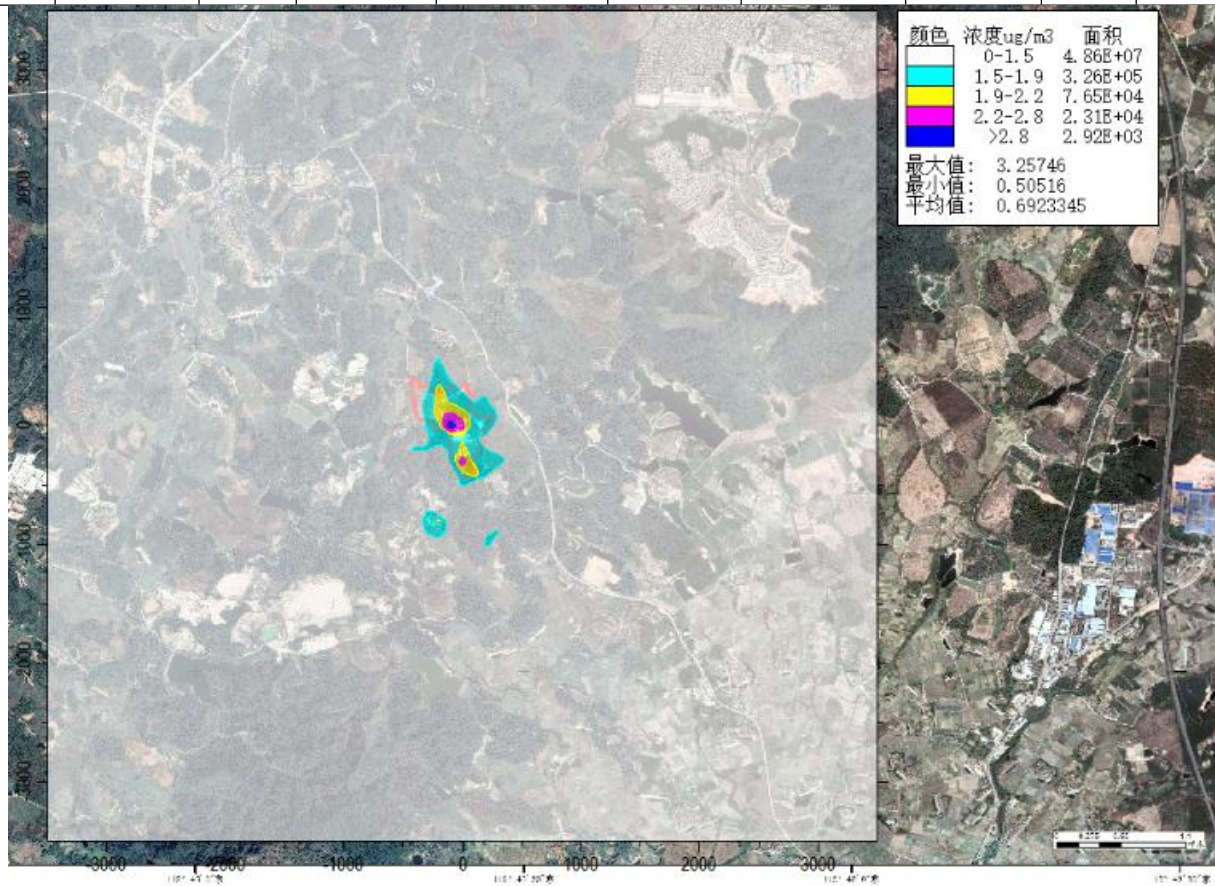
图 6.1-22 叠加后硫化氢 1 小时浓度分布图
