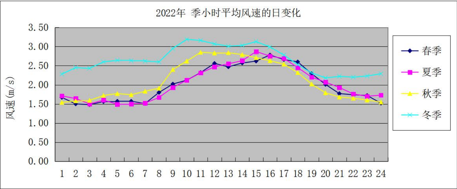
图6.1-9 台山市2022年季小时平均风速的变化图
