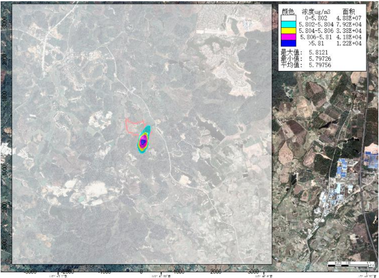
图 6.1-17b 叠加后 SO 2 年平均最大落地浓度分布图
