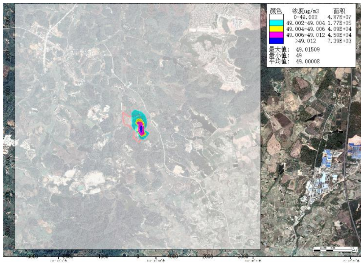
图 6.2-20a 叠加后 PM 2.5 95%保证率日平均最大落地浓度分布图
