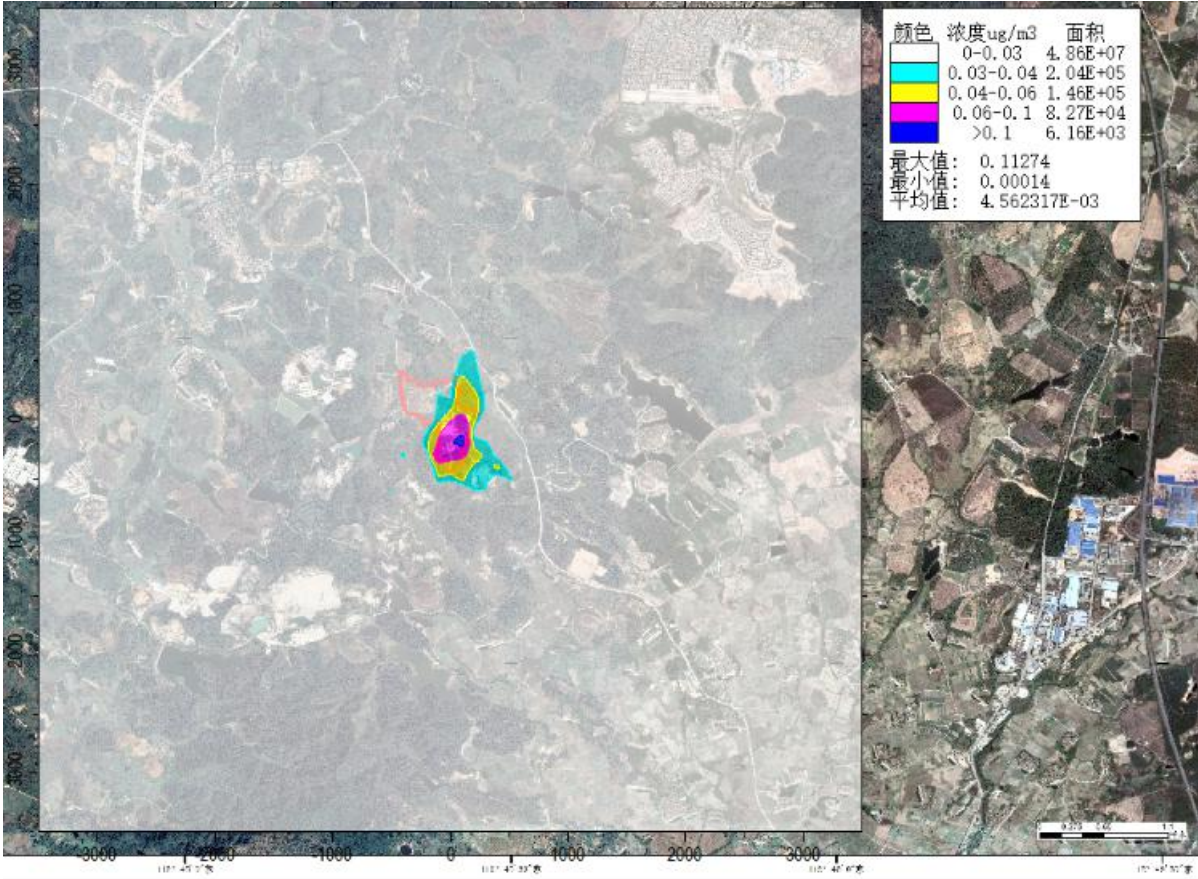
图 6.1-14a PM 2.5 新增污染源最大日均值浓度分布图
