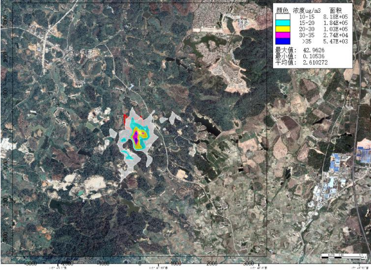
图 6.1-23 氨最大 1h 贡献浓度分布图（非正常工况）
