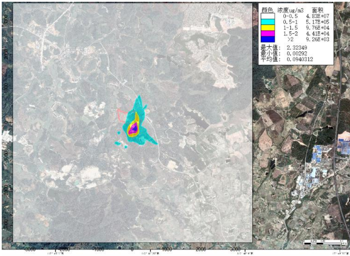
图 6.1-12b NO 2 新增污染源最大日均值浓度分布图
