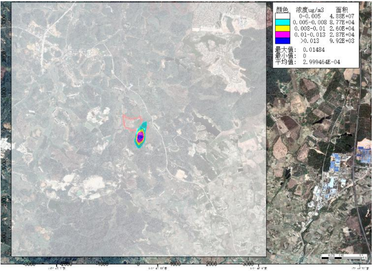
图 6.1-11c SO 2 新增污染源最大年均值浓度分布图
