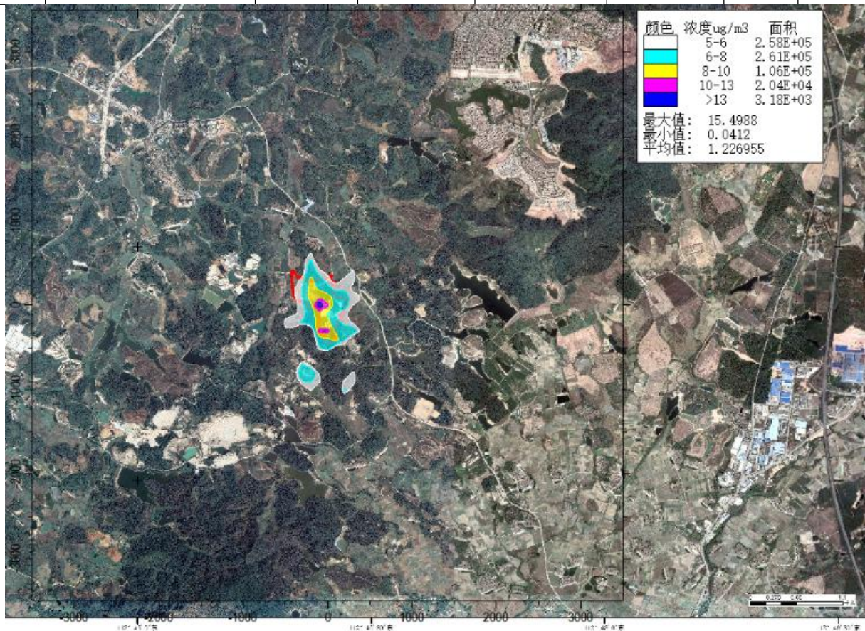
图 6.1-15 氨新增污染源最大 1 小时均值浓度分布图
