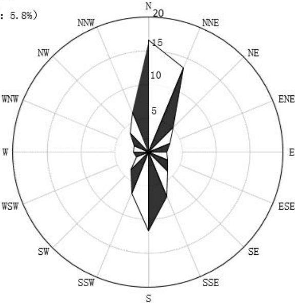
图 6.1-1 台山气象站风向玫瑰图（统计年限：2003-2022 年）
