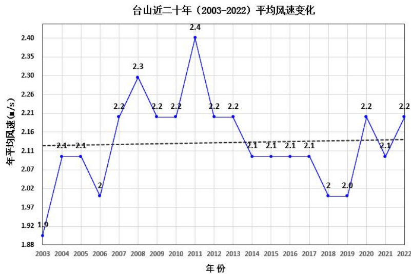
图 6.1-3 台山市（2003-2022）年平均风速（虚线为趋势线）
