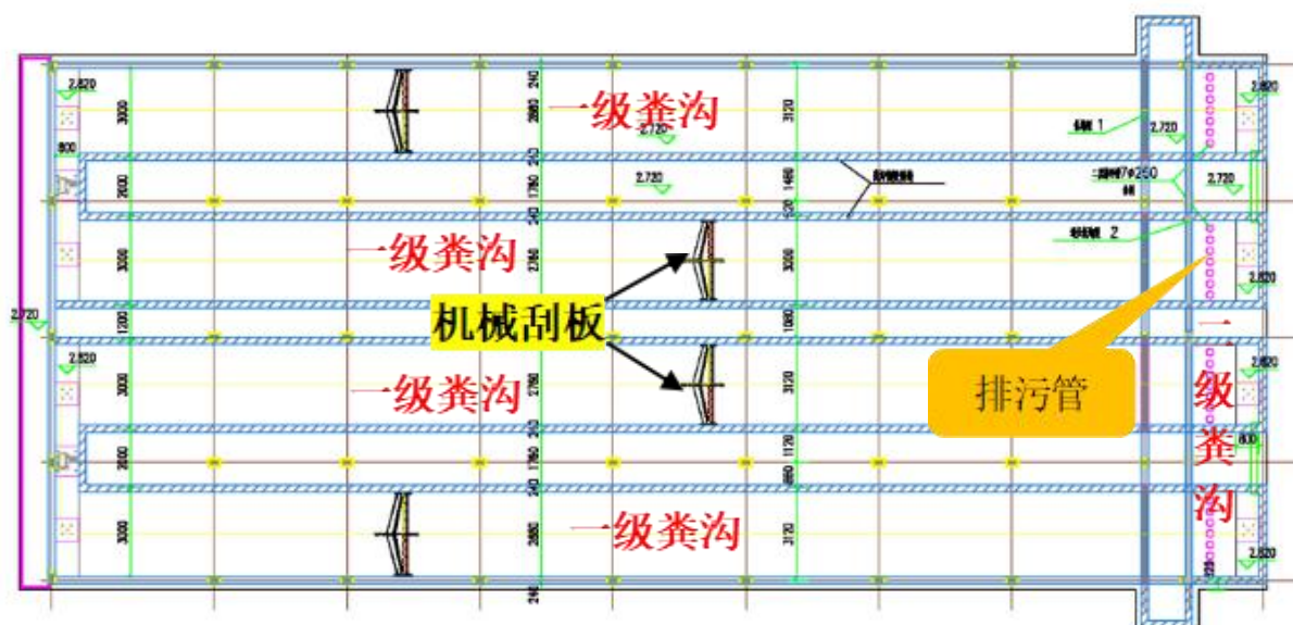
图 2.3-2 粪沟分布示意图
