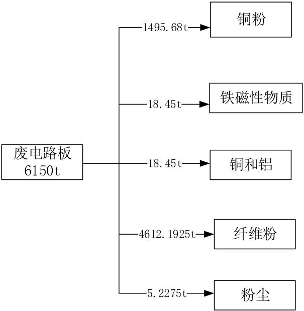
图 4.7-1 本项目总物料平衡图
