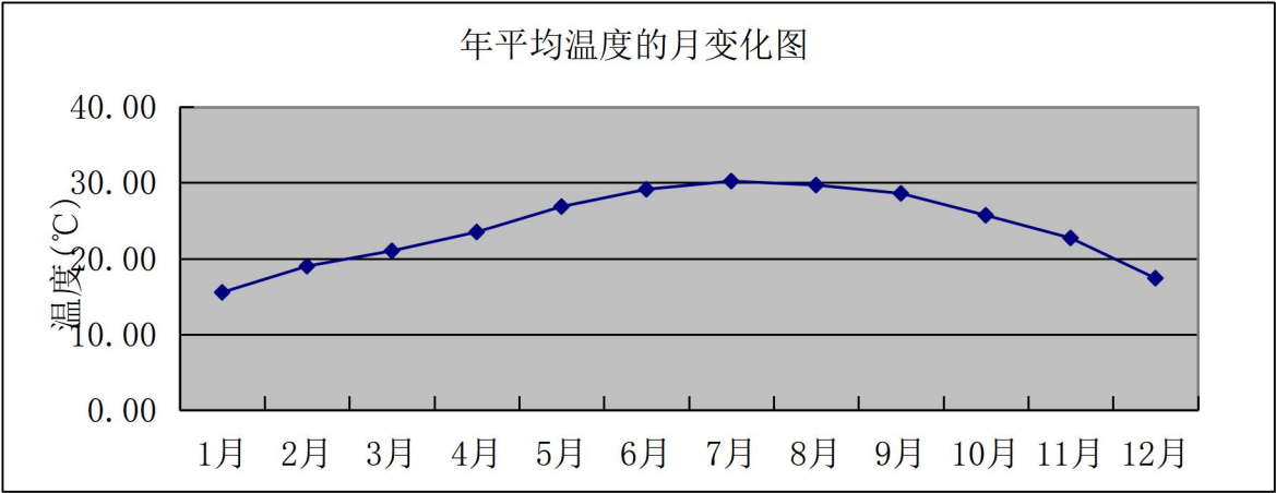
图 7.2-2 新会 2023 年月平均气温变化曲线
