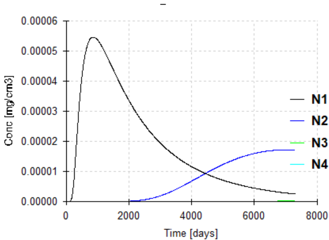
图 5.7.3-3 苯胺浓度—时间曲线图
