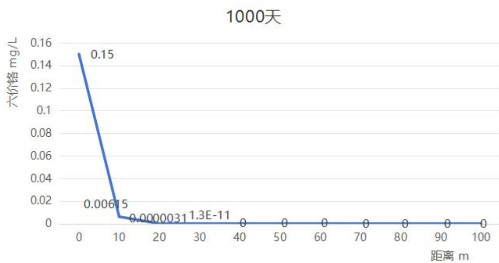
图5.3.3-6 污水六价铬渗漏1000d后，下游不同距离的六价铬浓度分布
