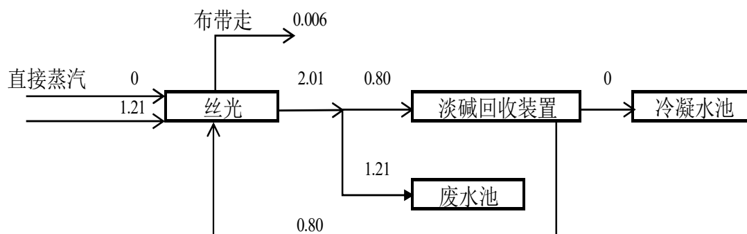
图 3.2.2-8 丝光过程碱平衡图 (单位: t/d)
