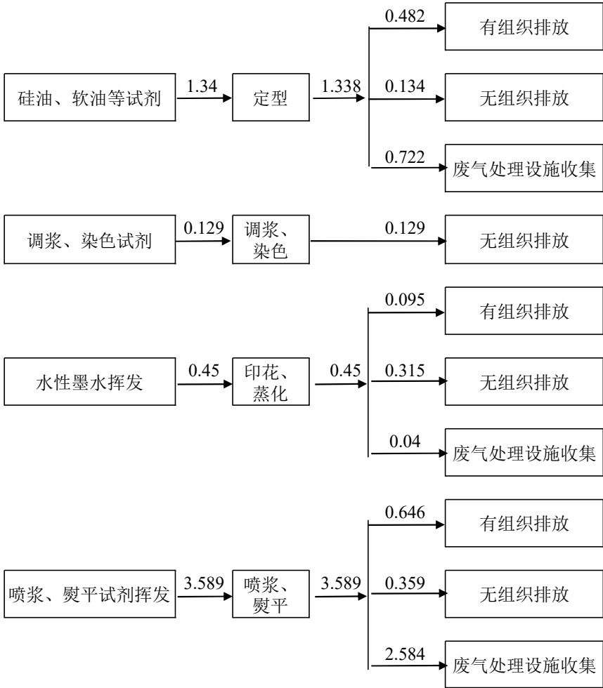
图 3.2.2-14 VOCs 平衡图
