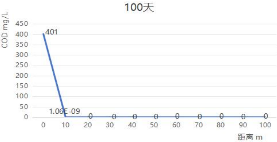
图5.3.3-1 污水COD渗漏100d后，下游不同距离的COD浓度分布
