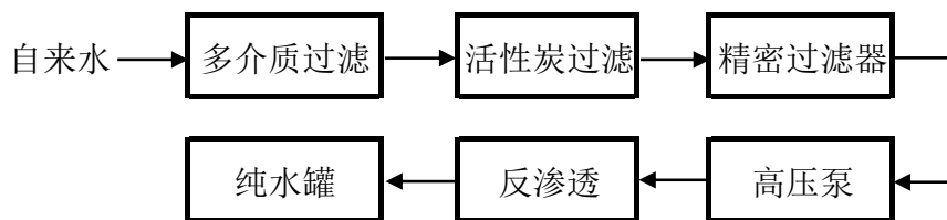
图 3.2.2-11 本项目制纯水系统生产工艺流程图
