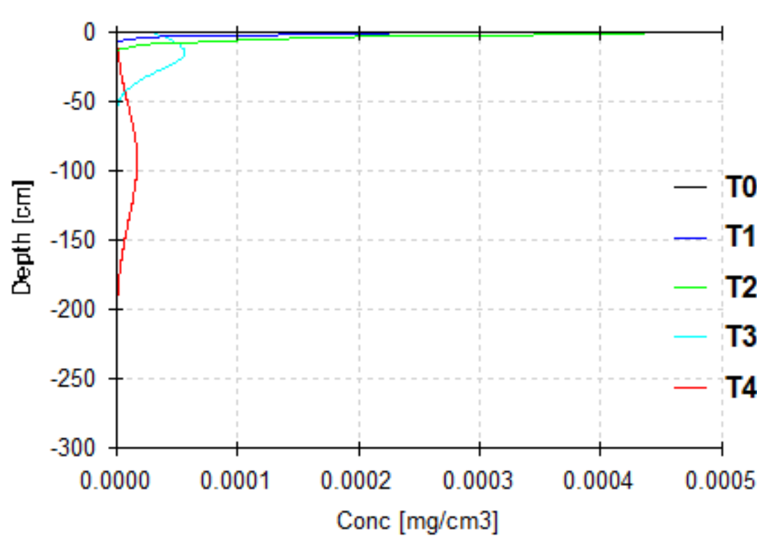
图 5.7.3-4 苯胺深度—深度曲线图
