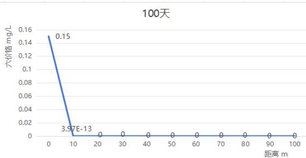
图5.3.3-5 污水六价铬渗漏100d后，下游不同距离的六价铬浓度分布
