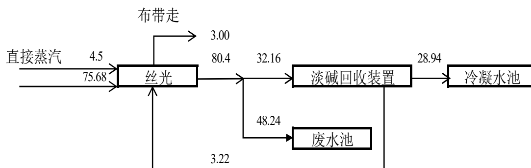
图 3.2.2-7 丝光过程水量平衡图（单位：t/d）
