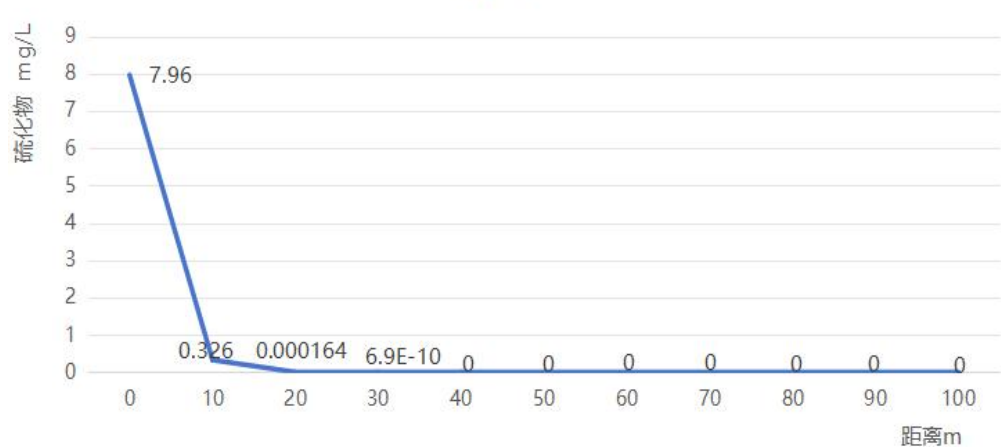
图5.3.3-4 污水硫化物渗漏1000d后，下游不同距离的硫化物浓度分布
