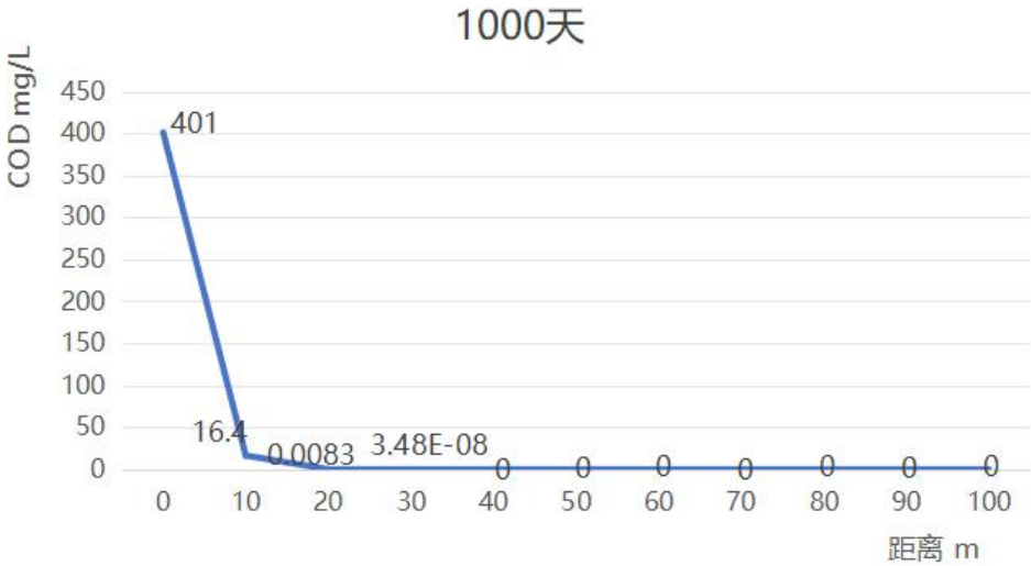
图5.3.3-2 污水COD渗漏1000d后，下游不同距离的COD浓度分布
