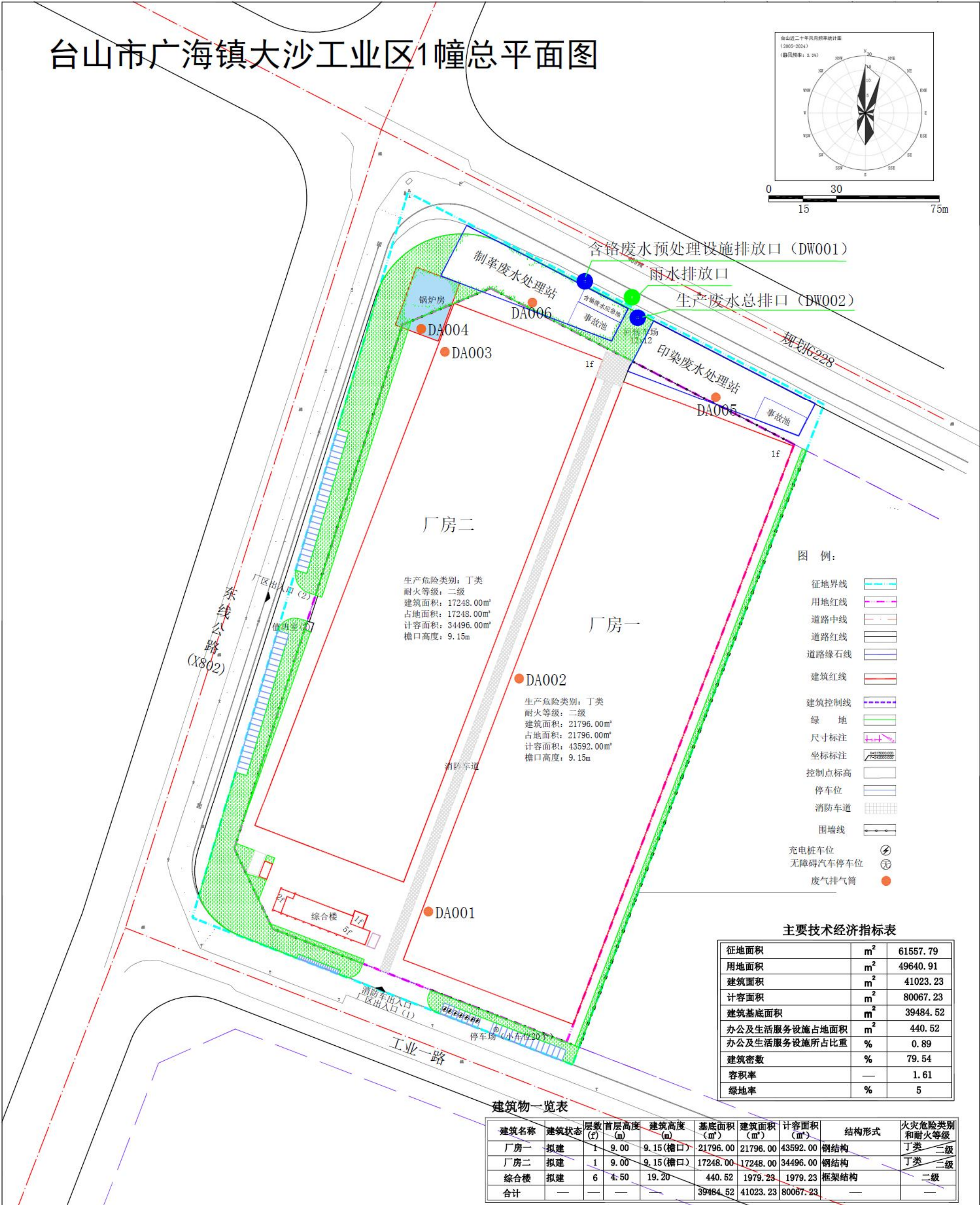
图 3.1.2-1 总平面布置图
