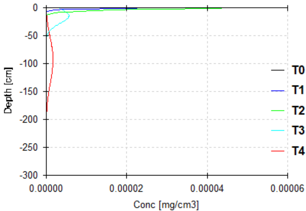
图 5.7.3-6 六价铬深度—深度曲线图
