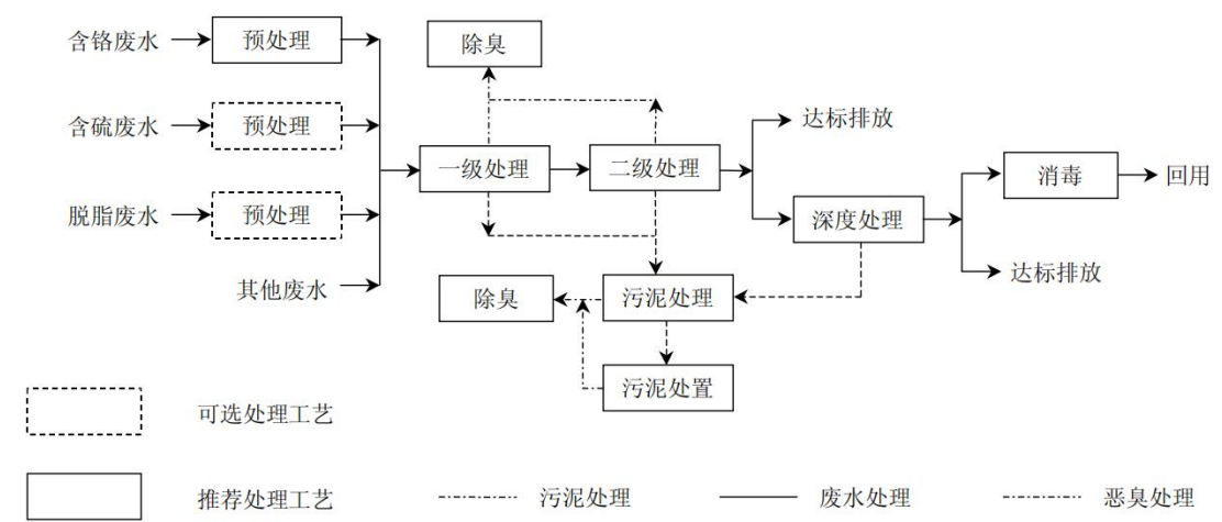
图 6.1.2-1 制革加工废水治理工程工艺流程图
