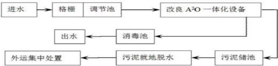
图 4-1 月山镇污水处理厂污水处理工艺流程图
