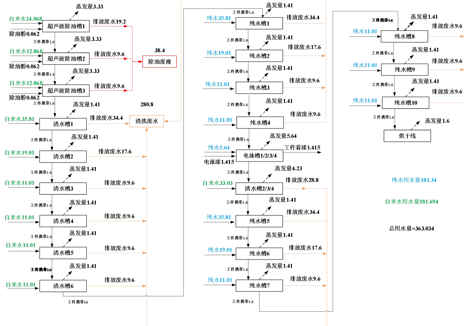
图 2-3 电泳线水平衡图 (单位: m³/a)
