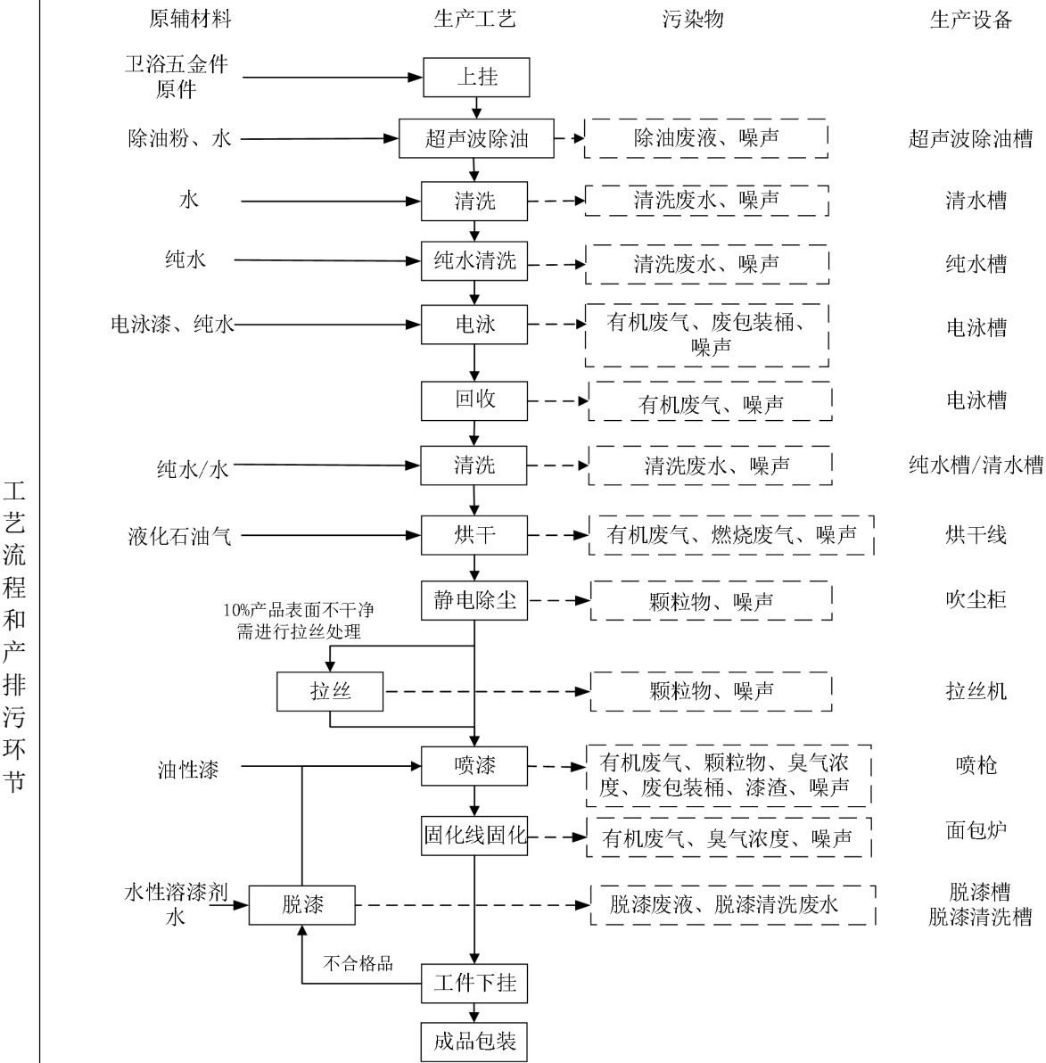
图 2-5 生产工艺流程及产污环节图
