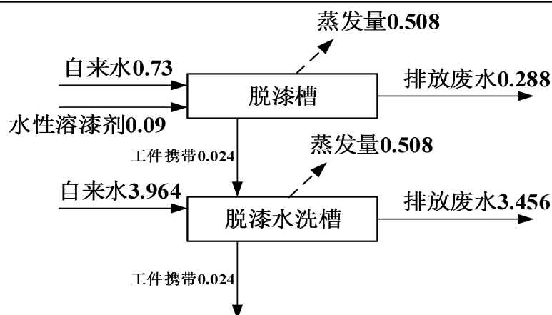
图 2-1 脱漆线水平衡图
