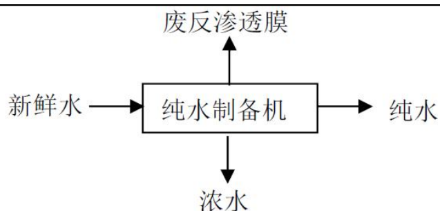
图 2-6 纯水制备工艺流程及产污环节示意图
