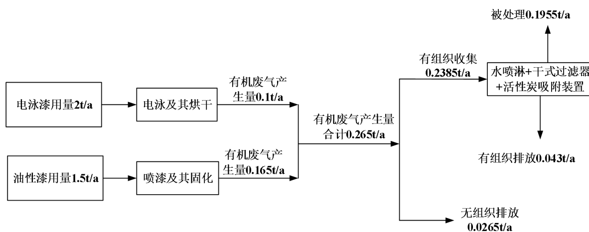
图 2-4 项目 VOCs 平衡图（单位：t/a）
