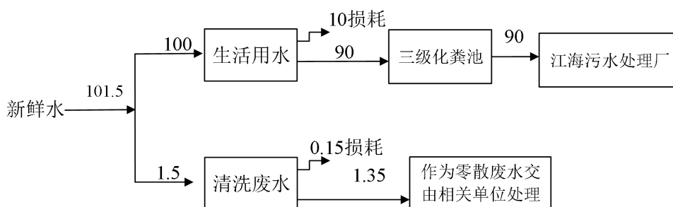
图 2-1 项目水平衡图 ( \text{m}^3/\text{a} )
