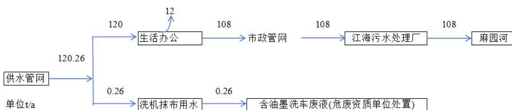
图 2-2 水量平衡图
