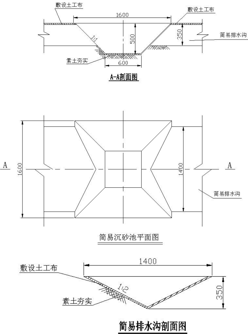
专项图 6 典型生态保护措施设计图（简易排水沟与沉砂池）
