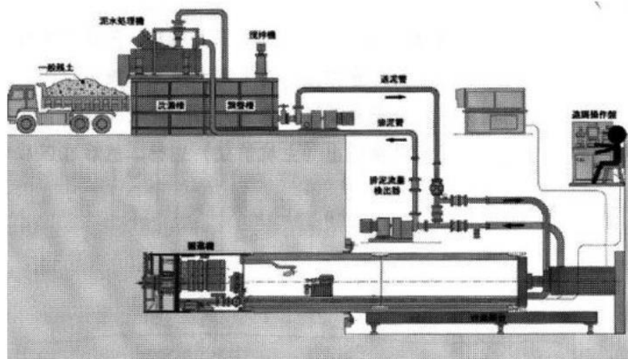
图 2-6 顶管施工工艺示意图
