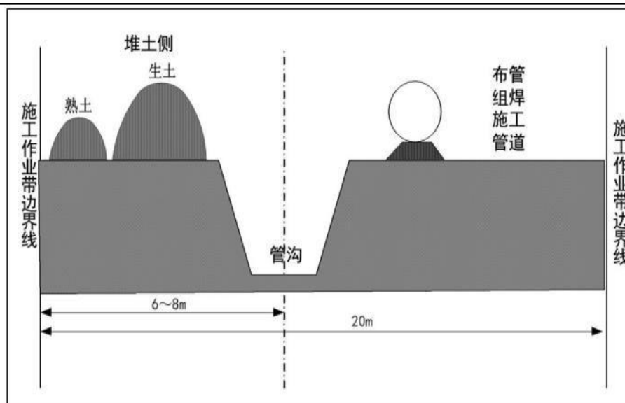
图 2-5 大开挖工程施工流程示意图
