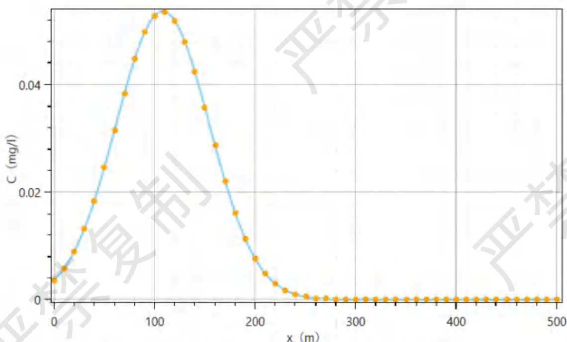
图6.2-4b 污水池渗漏1000d后，下游不同距离的氨氮浓度分布
