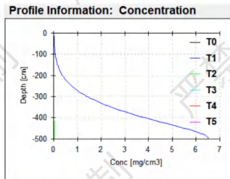
图 6.7-2 观测点甲酚浓度与深度曲线图
