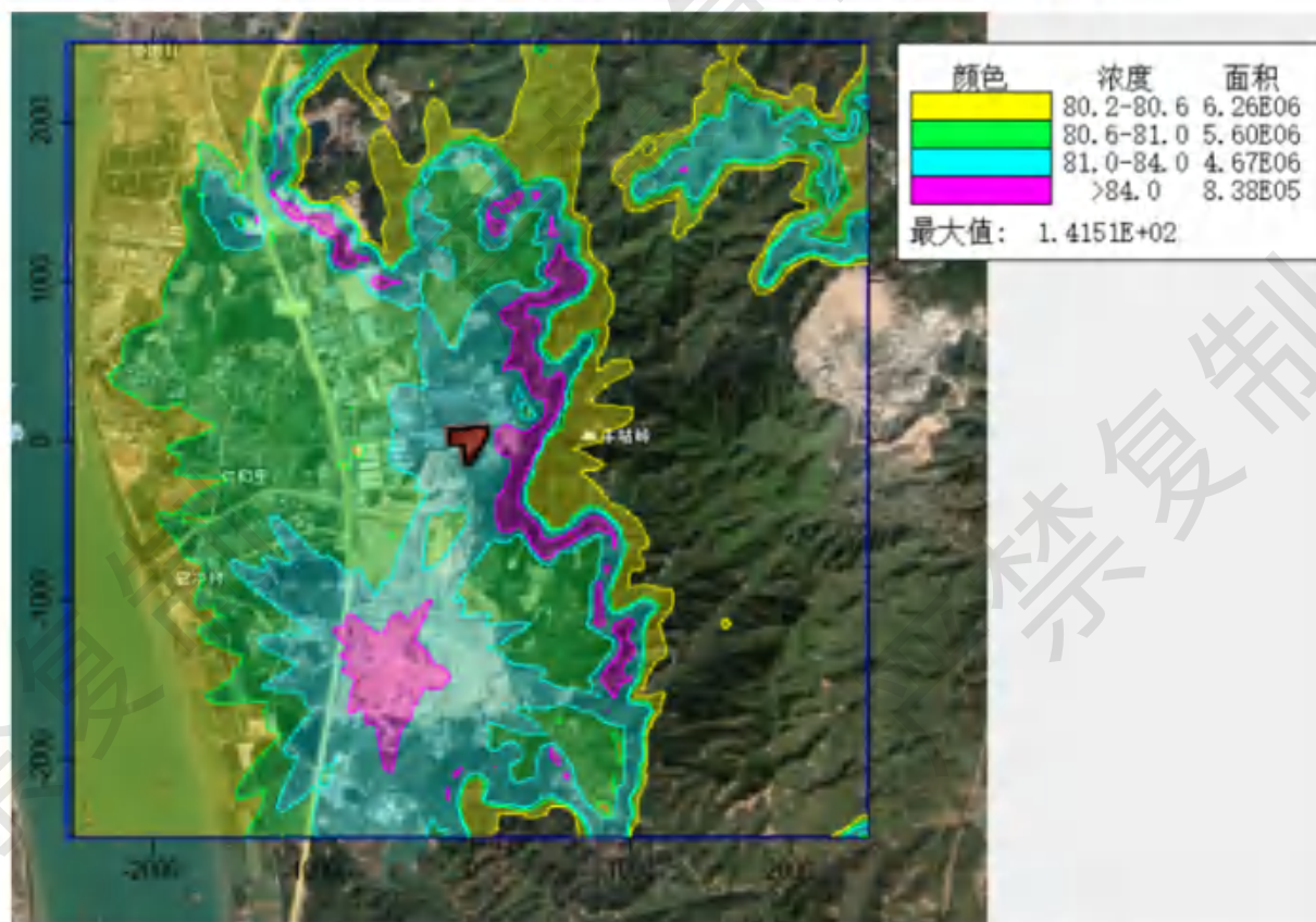
图 6.3-11L 氨叠加现状值后小时平均质量浓度分布图 (单位 \mu\text{g}/\text{m}^3 )
