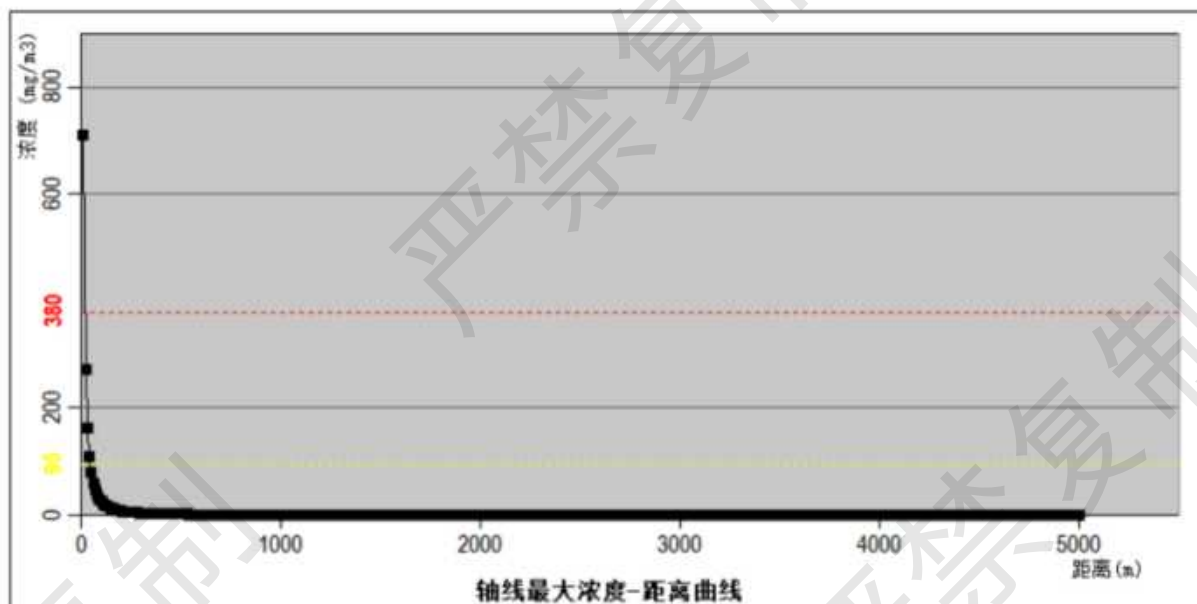
图 6.6-9a 最常见气象条件下乙类罐组异丁醇燃烧产生 CO 下风向不同距离处的最大浓度
