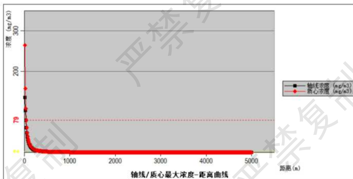
图 6.6-14a 最不利气象条件下甲类仓库 1 物料燃烧产生二氧化硫下风向不同距离处的最大浓度
