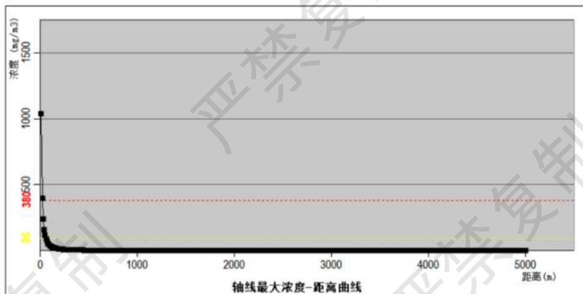
图 6.6-7a 最常见气象条件下甲类罐组甲酚燃烧产生 CO 下风向不同距离处的最大浓度
