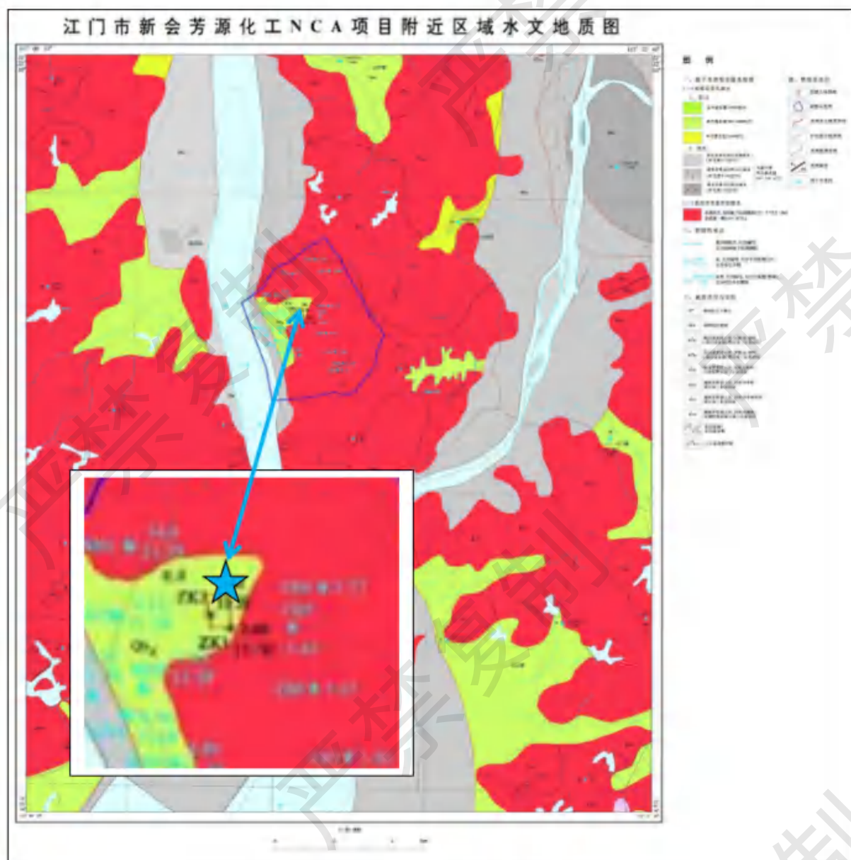
图6.2-2 区域水文地质图
