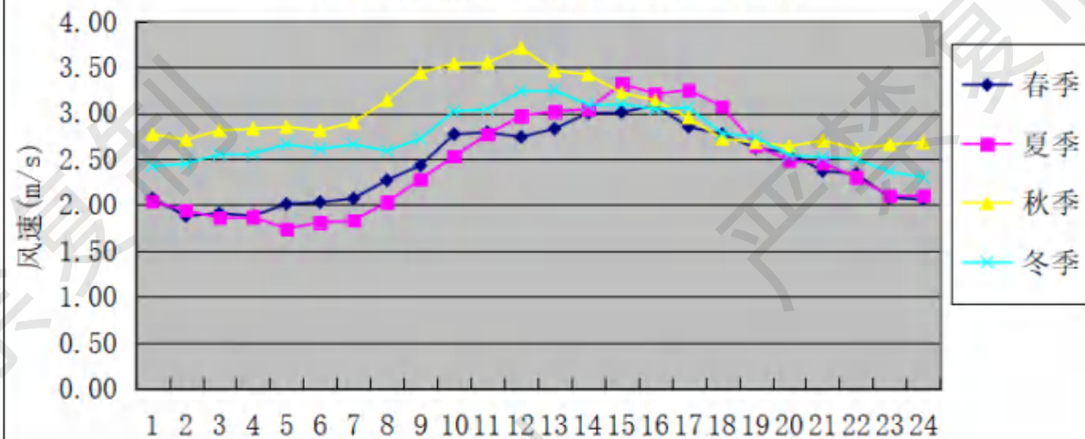
图 6.3-4d 新会一般气象站 (59476) 2024 年季小时平均风速的日变化图
