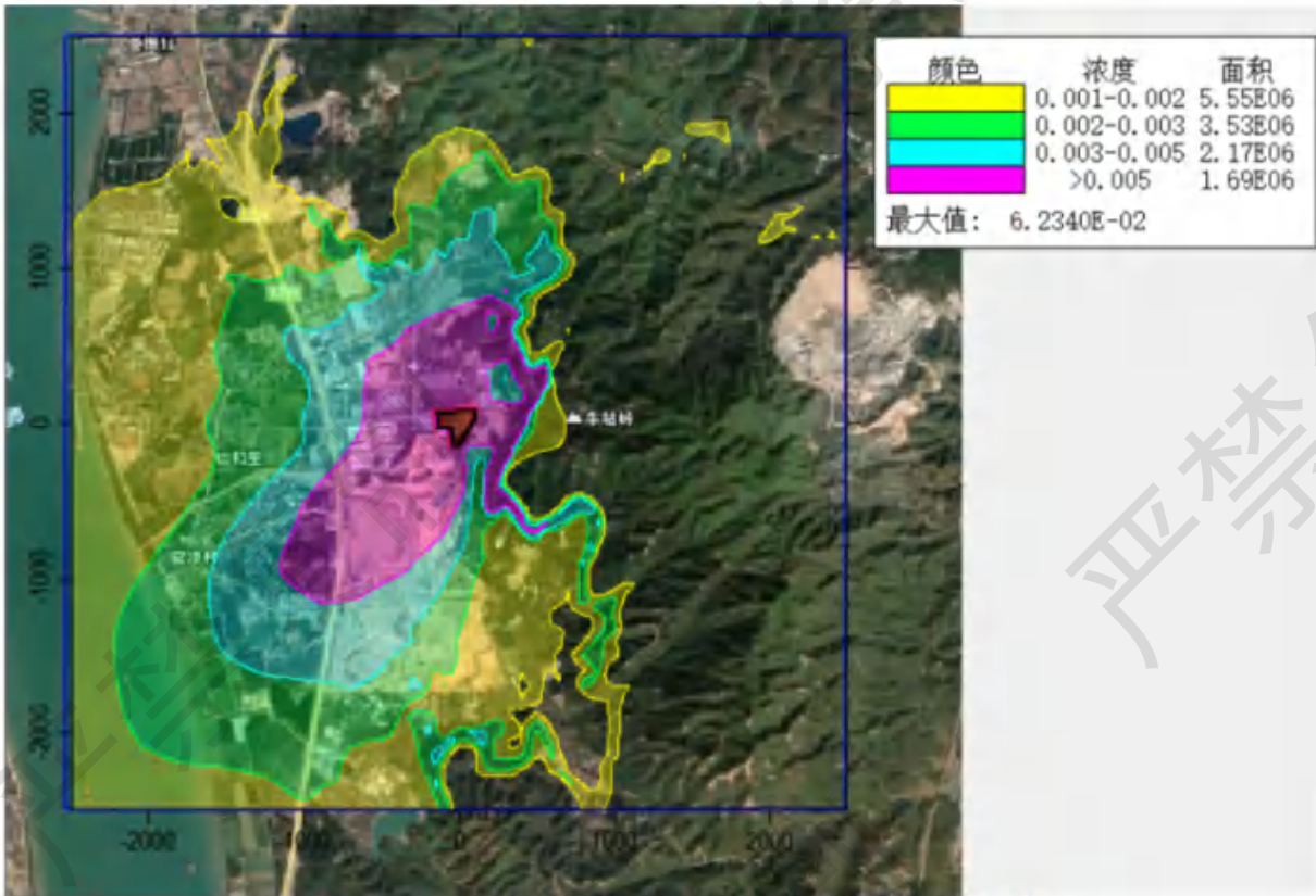
图 6.3-10b NO 2 年均浓度最大增值等值线图 (单位 \mu\text{g}/\text{m}^3 )
