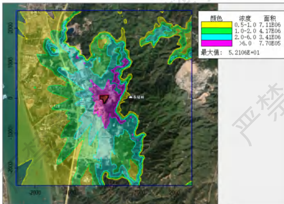
图 6.3-8d 非甲烷总烃小时浓度最大增值等值线图 (单位 \mu\text{g}/\text{m}^3 )
