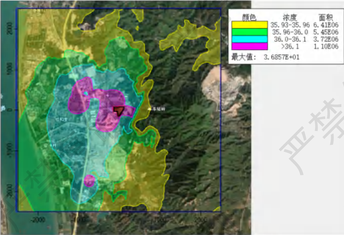
图 6.3-11g PM 10 叠加现状值后年均质量浓度分布图 (单位 \mu\text{g}/\text{m}^3 )
