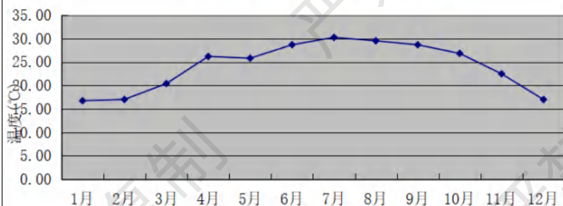
图 6.3-4b 新会一般气象站 (59476) 2024 年平均温度月变化图
