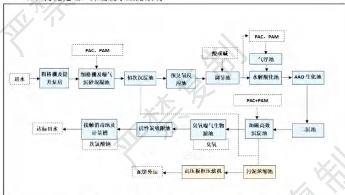
图 6.1-3 江门市新会古井新材料集聚区污水处理厂工艺流程图
