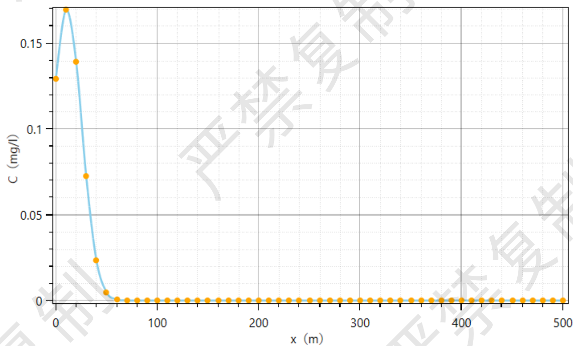
图6.2-4a 污水池渗漏100d后，下游不同距离的氨氮浓度分布
