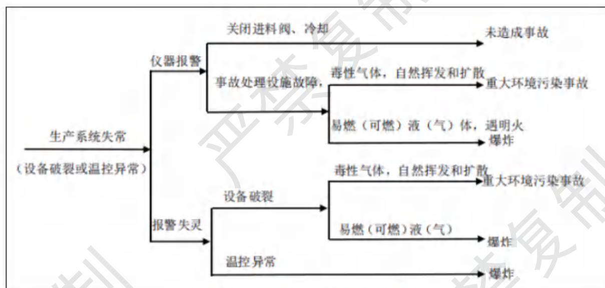
图 6.6-5 生产系统事件树示意图
