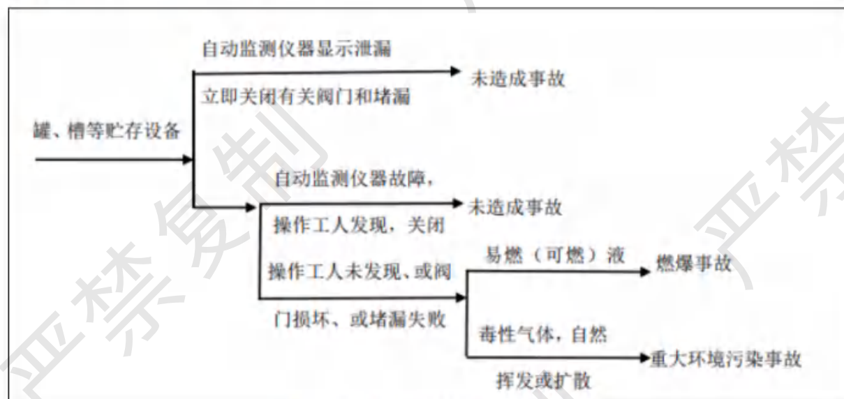
图 6.6-4 储罐系统事件树示意图
