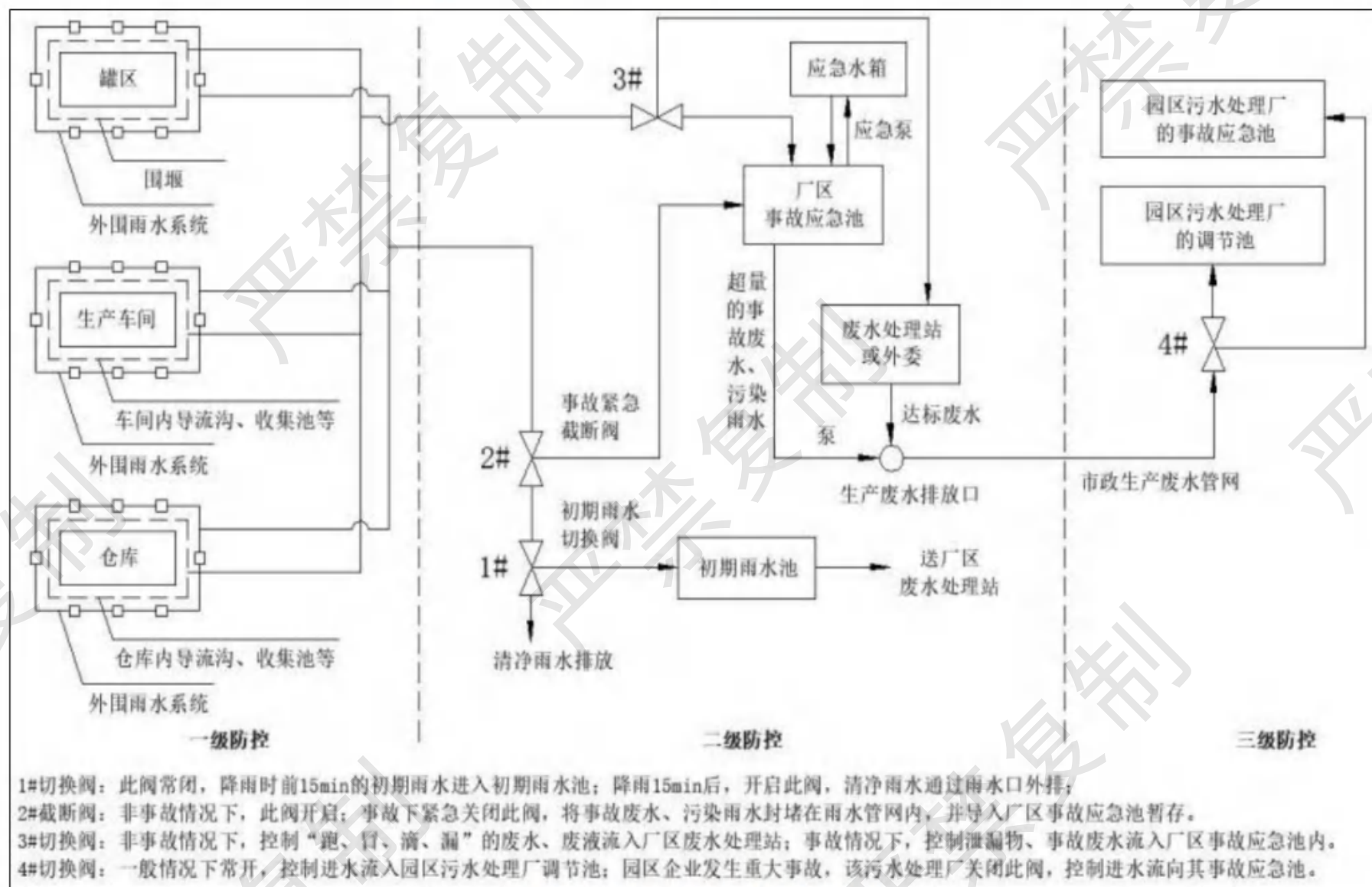
图 6.6-20 项目“三级”防控体系示意图
