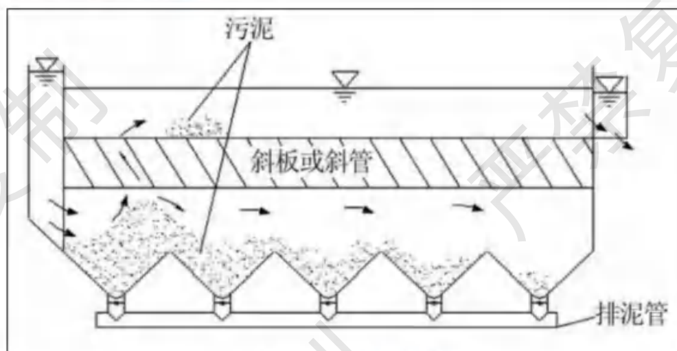
图 7.2-3 沉淀池示意图
