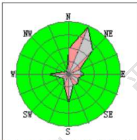
图 6.3-4a 新会一般气象站（59476）累年各季风向玫瑰图（统计年限：2005～2024 年）
