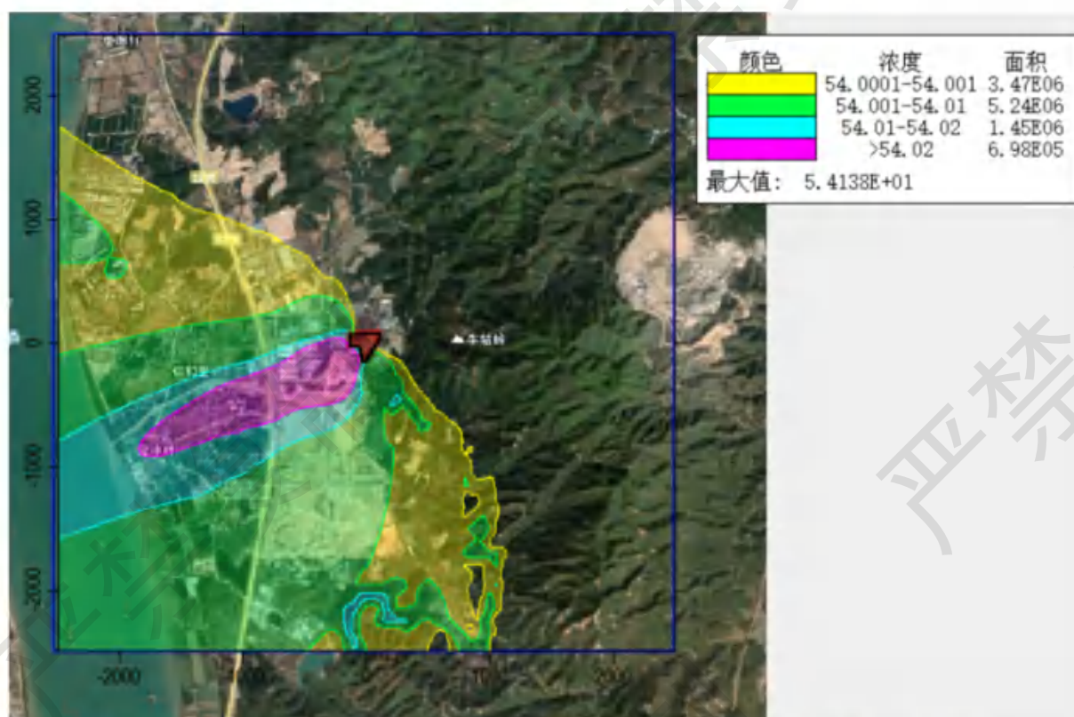
图6.3-11c NO 2 叠加现状值后98%保证率日均质量浓度分布图 (单位 \mu\text{g}/\text{m}^3 )
