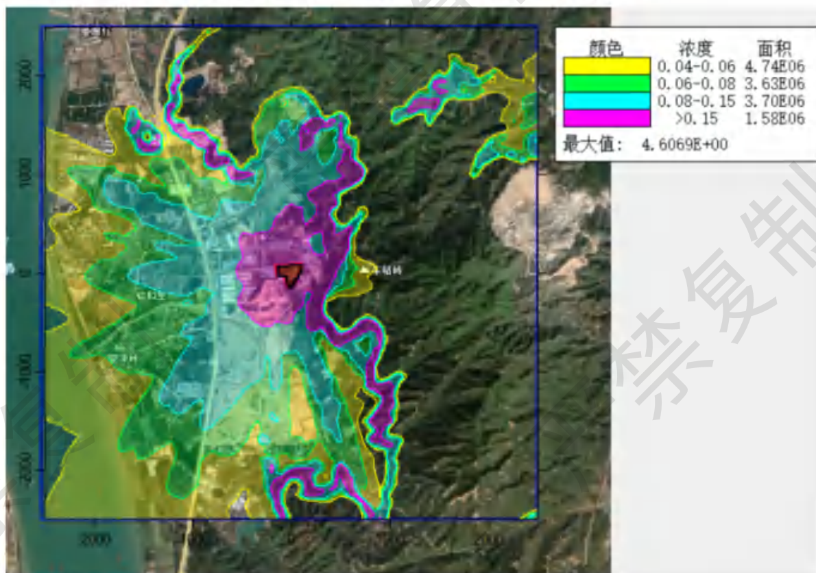
图 6.3-9f 氯化氢日均浓度最大增值等值线图 (单位 \mu g/m^3 )
