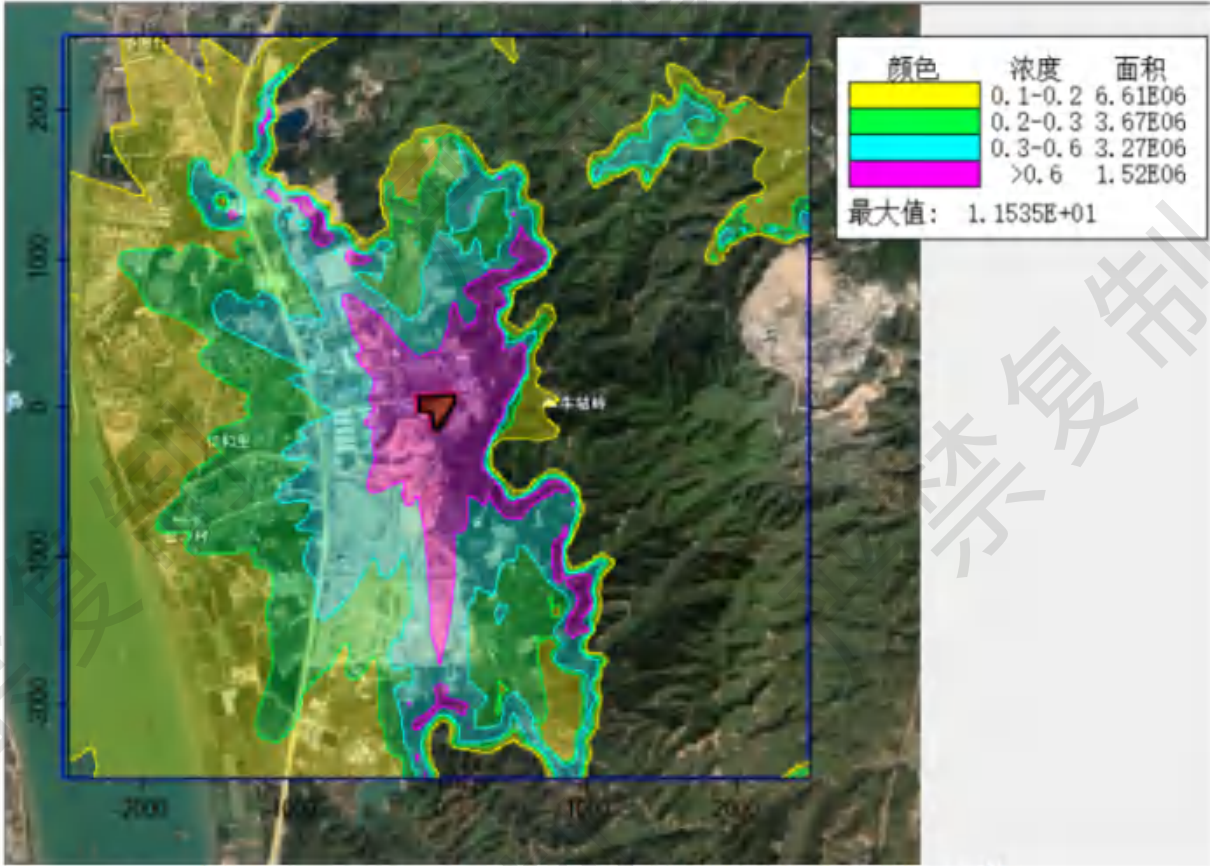
图 6.3-8c TVOC 8 小时平均浓度最大增值等值线图 (单位 \mu\text{g}/\text{m}^3 )
