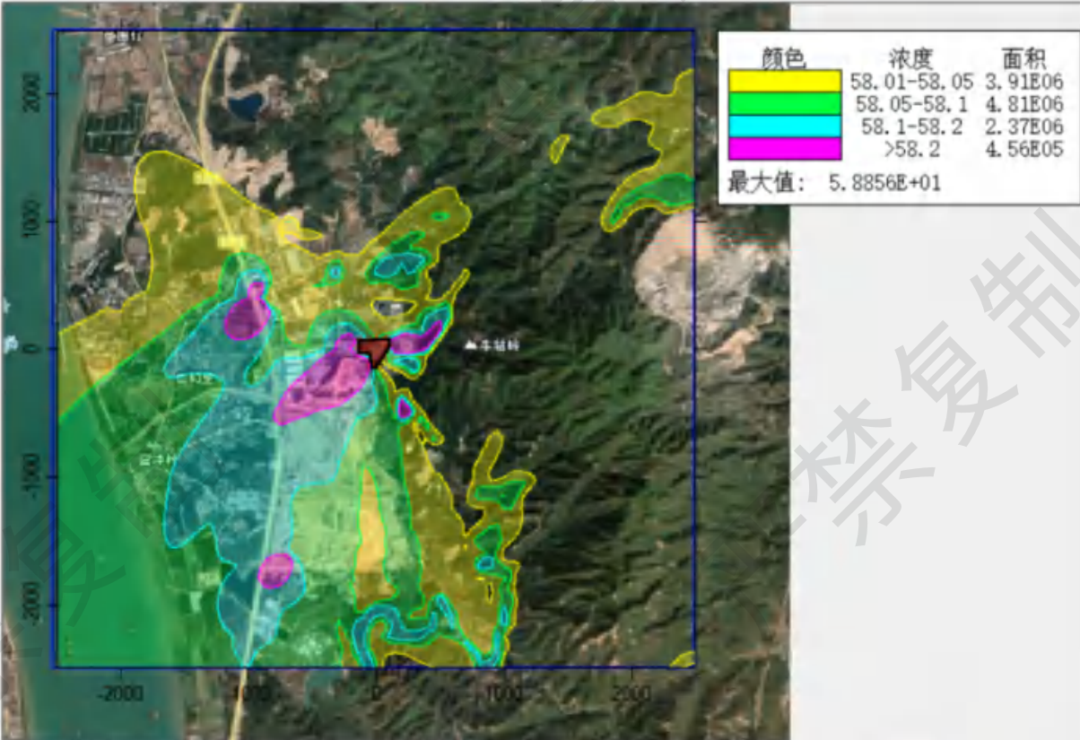
图 6.3-11h PM 2.5 叠加现状值后 95%保证率日均质量浓度分布图 (单位 \mu\text{g}/\text{m}^3 )
