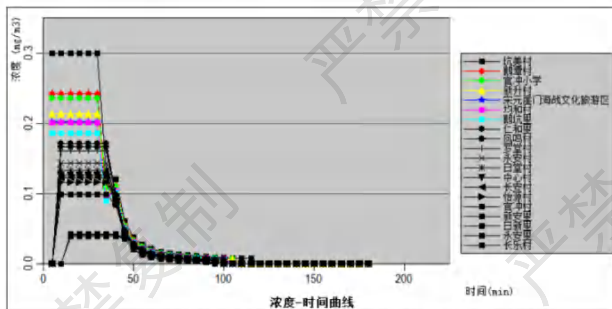
图 6.6-15c 各敏感点甲类仓库 1 物料燃烧产生二氧化硫浓度随时间变化情况
