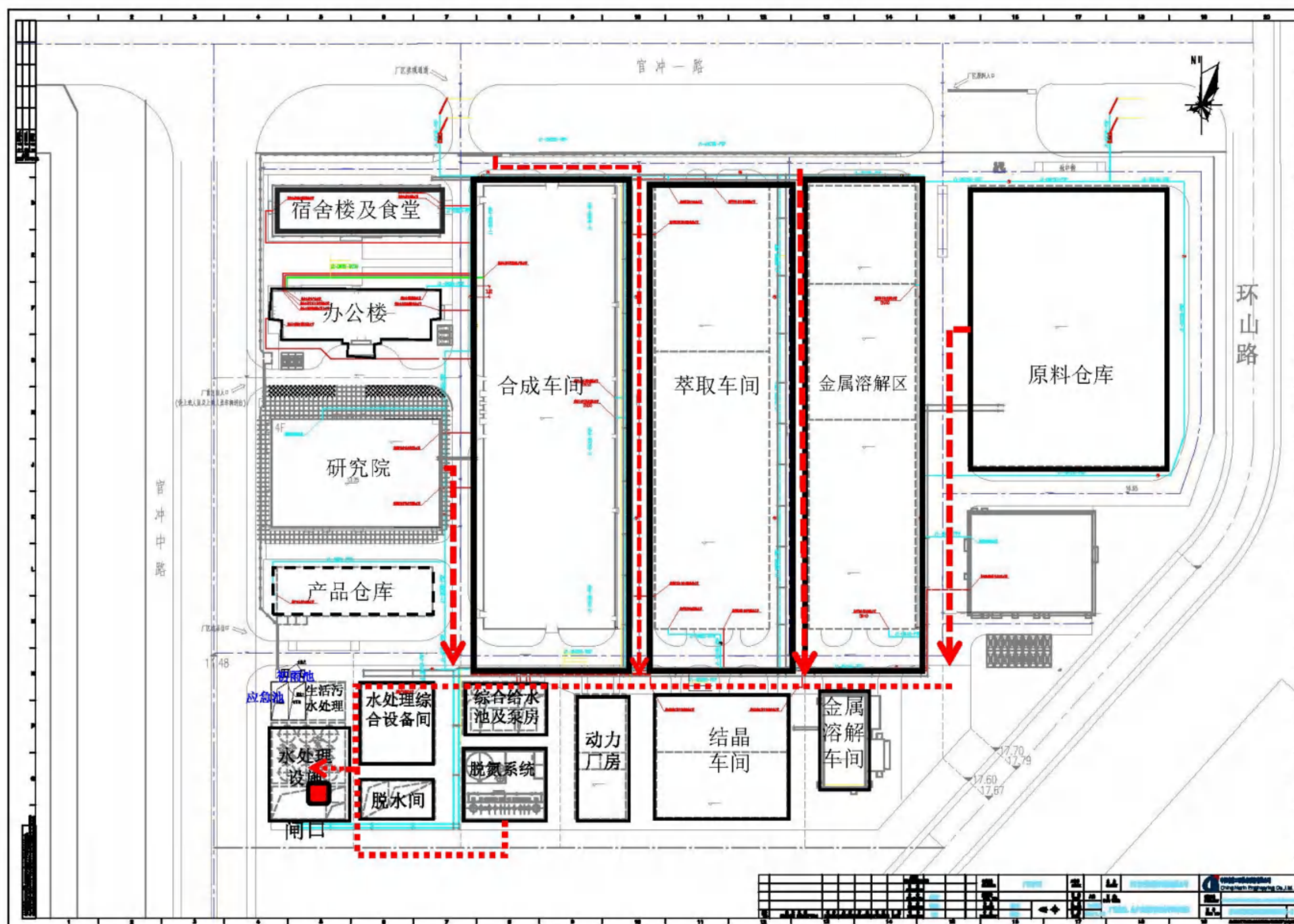
图 9.6-19 生产废水收集管网示意图
