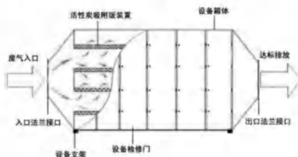
图 10.2-1 活性炭吸附器结构示意图
