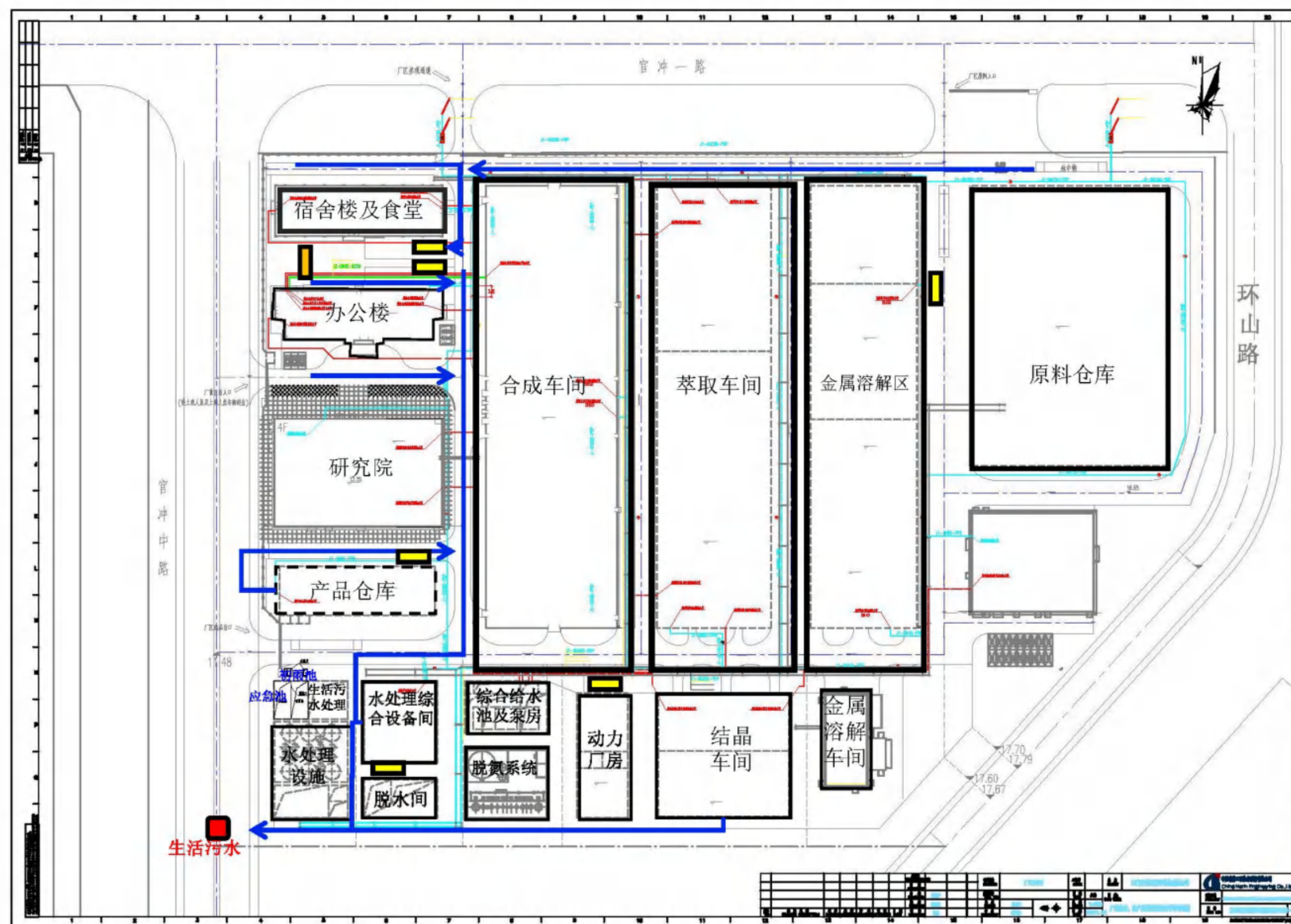
图 9.6-18 生活污水收集管网示意图
