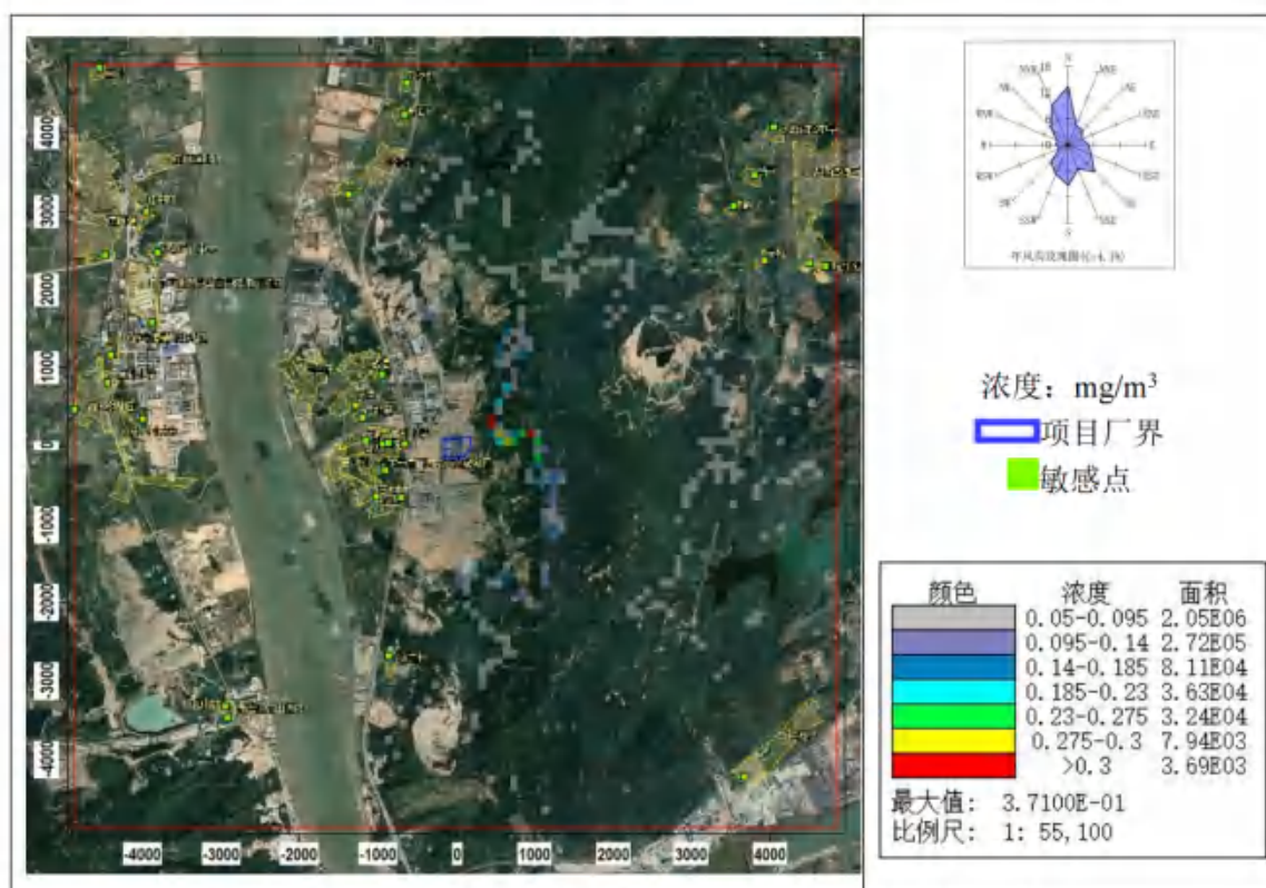
图 8.2-54 锰及其化合物小时平均浓度分布图（非正常排放状况）
