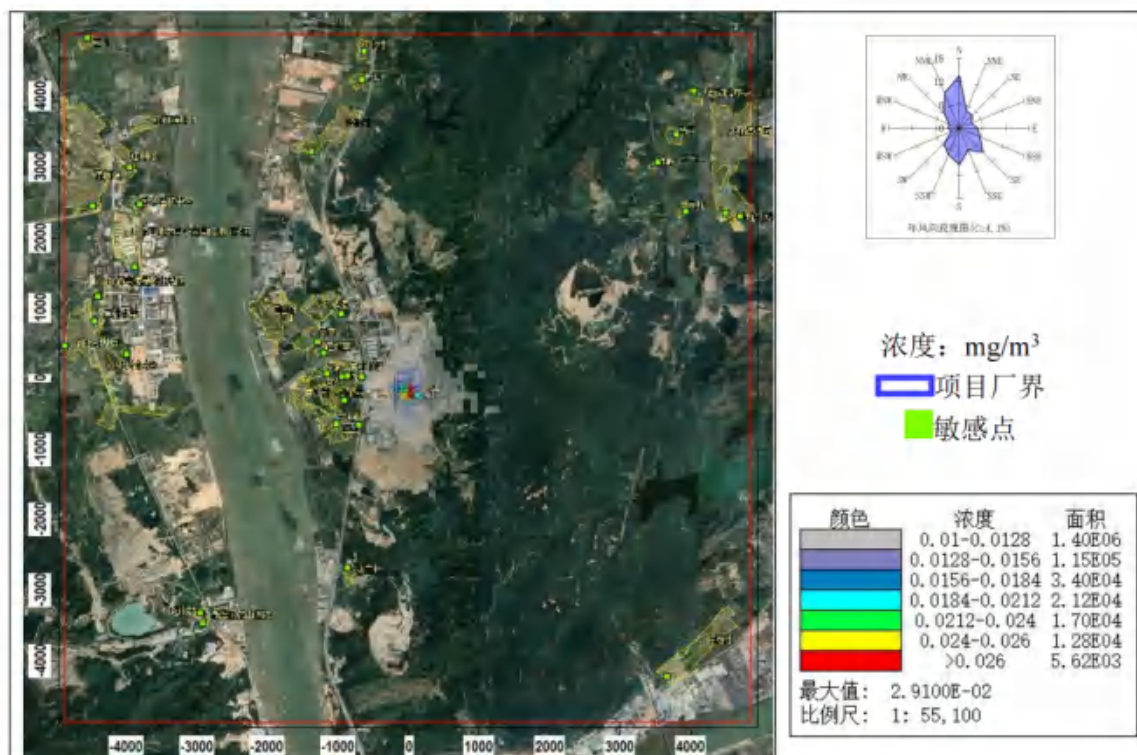
图 8.2-30 硫酸雾日平均浓度分布图（叠加在建、拟建源及背景后）
