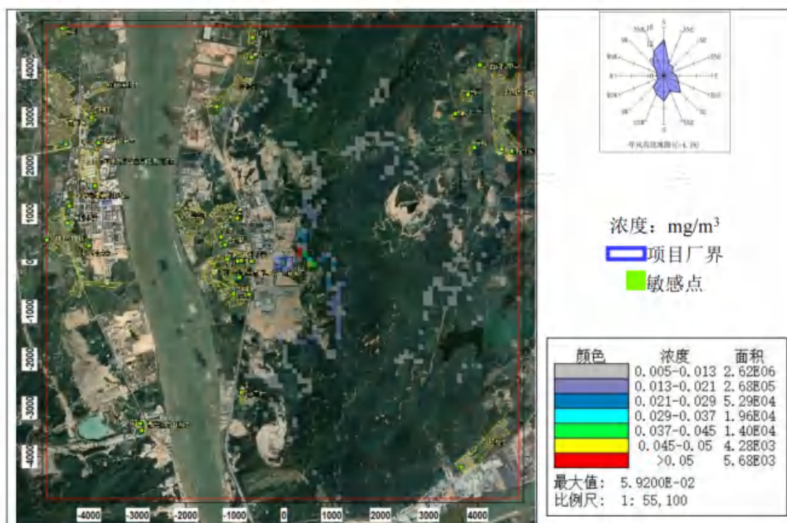
图 8.2-58 硫化氢小时平均浓度分布图（非正常排放状况）
