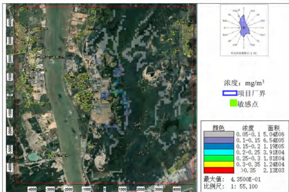
图 8.2-46 \text{NO}_2 小时平均浓度分布图 (非正常排放状况)
