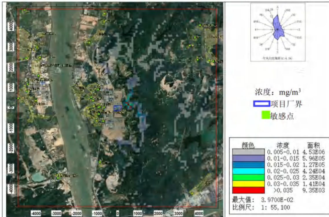
图 8.2-23 NMHC 小时平均浓度分布图
