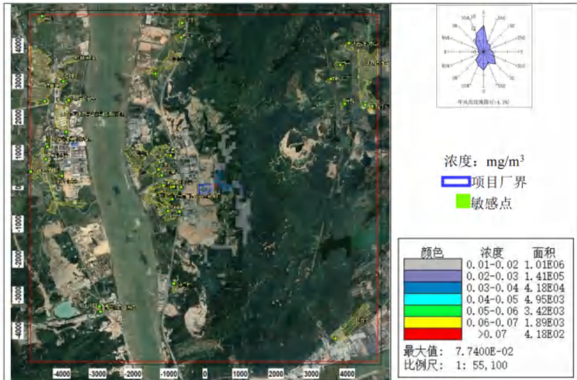
图 8.2-27 硫酸雾小时平均浓度分布图
