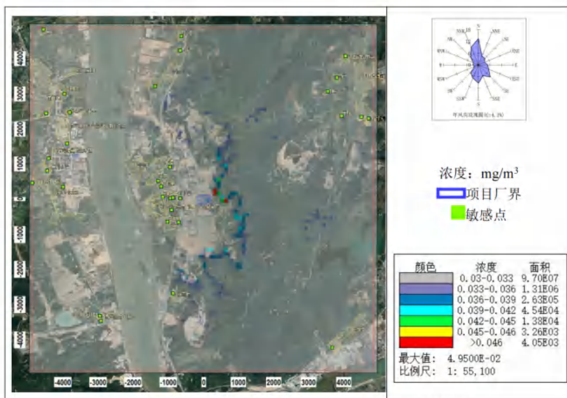
图 8.2-33 HCl 小时平均浓度分布图（叠加在建、拟建源及背景后）
