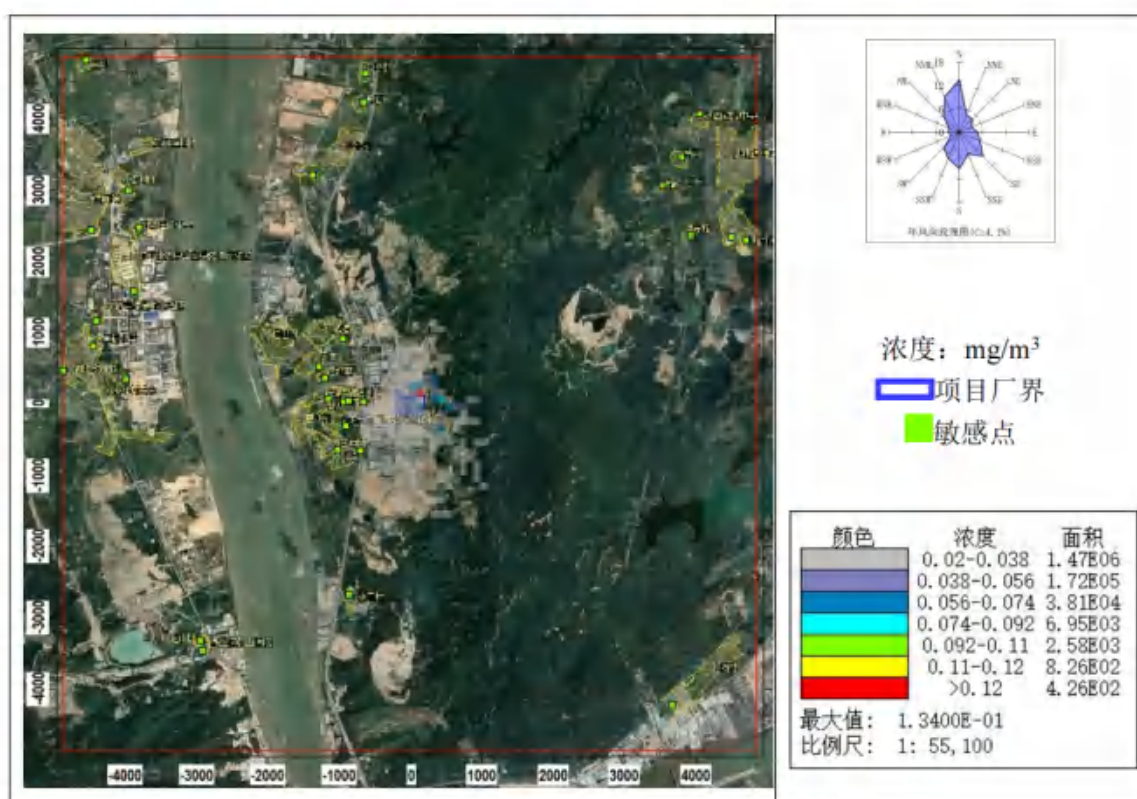
图 8.2-55 氨小时平均浓度分布图（非正常排放状况）
