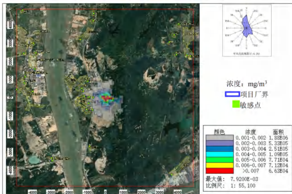
图 8.2-11 TSP 日平均浓度分布图
