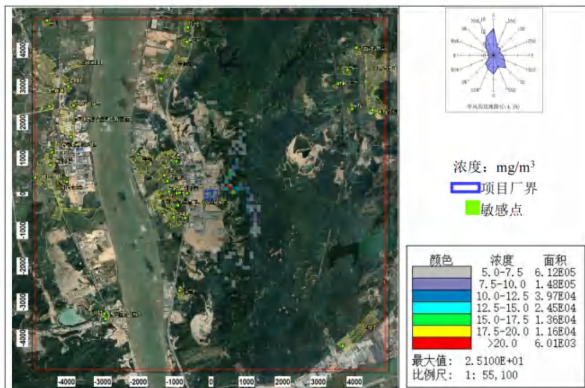
图 8.2-50 NMHC 小时平均浓度分布图 (非正常排放状况)
