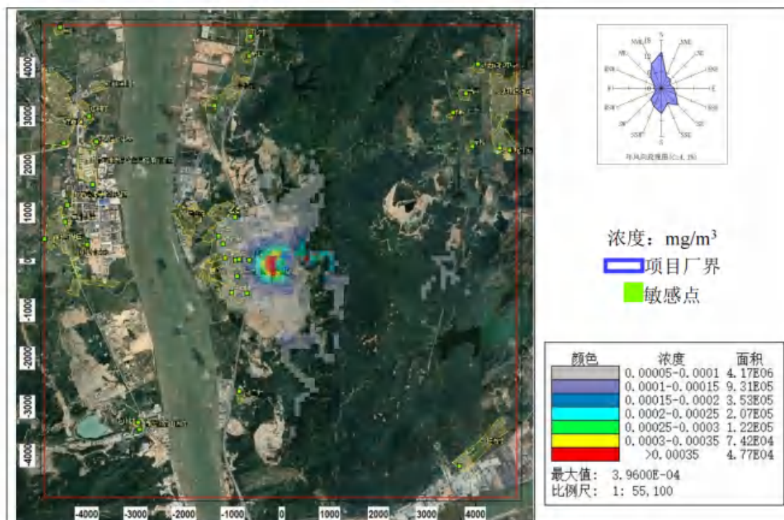
图 8.2-16 \text{PM}_{10} 年平均浓度分布图
