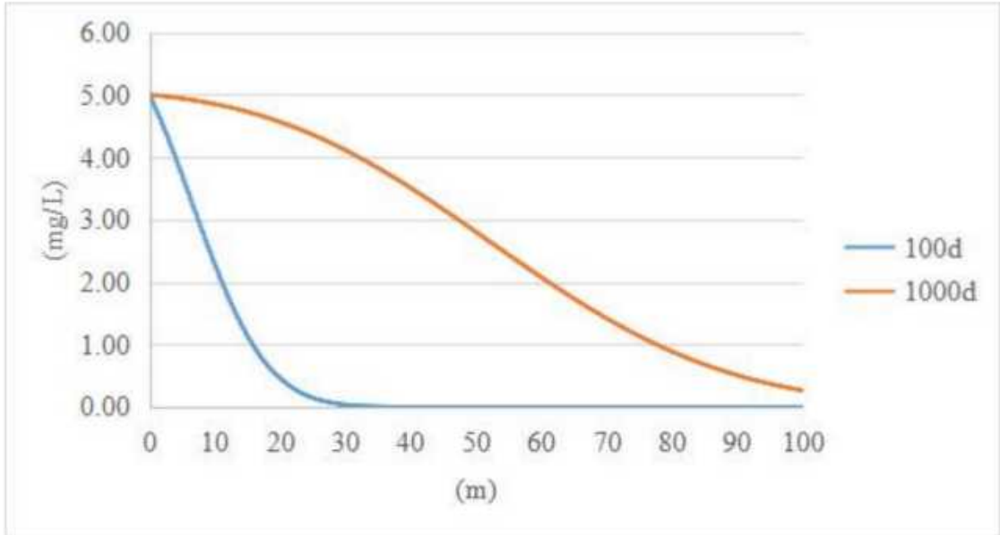
图 8.4-5 污染物连续渗漏情况预测统计图（钴）
