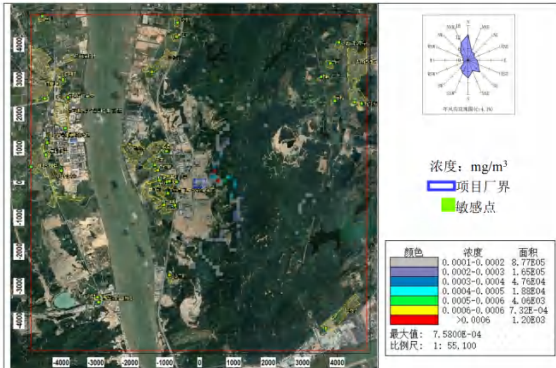
图 8.2-41 硫化氢小时平均浓度分布图
