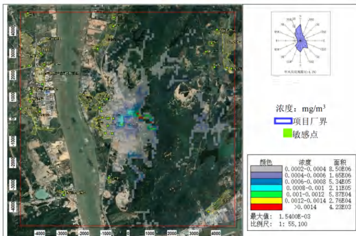
图 8.2-19 \text{PM}_{2.5} 日平均浓度分布图
