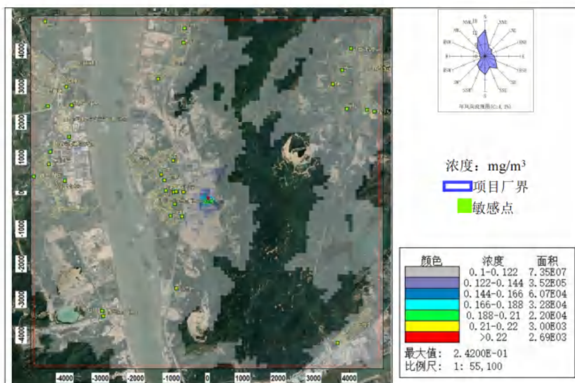
图 8.2-26 TVOC 8 小时平均浓度分布图 (叠加在建、拟建源及背景后)
