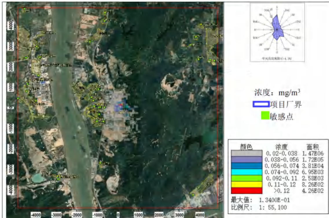
图 8.2-37 氨气小时平均浓度分布图
