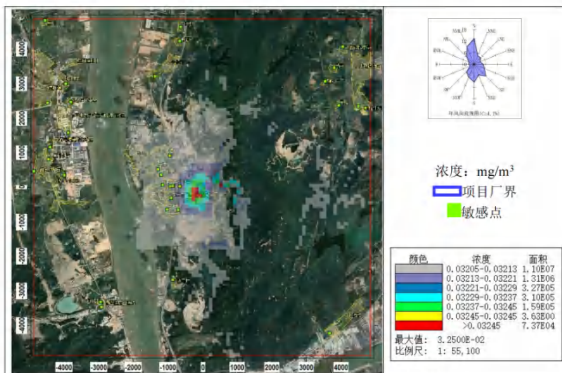
图 8.2-18 \text{PM}_{10} 年平均浓度分布图 (叠加在建、拟建源及背景后)
