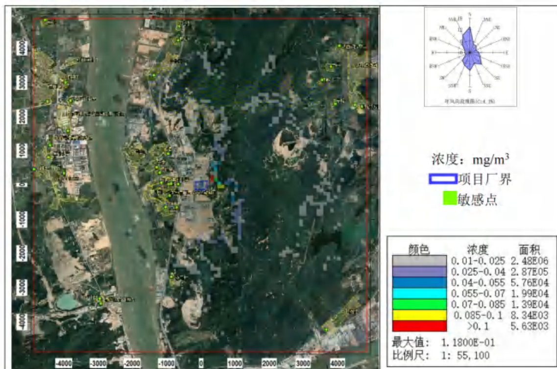
图 8.2-51 TVOC 小时平均浓度分布图 (非正常排放状况)
