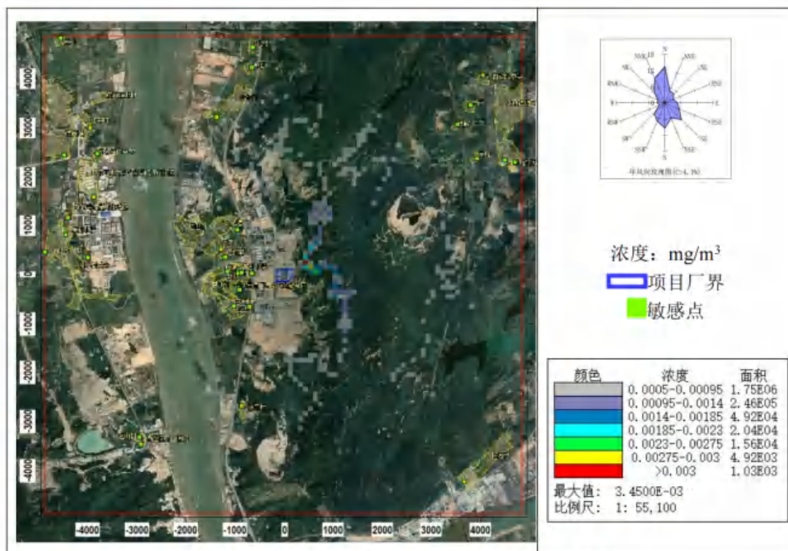
图 8.2-56 二噁英小时平均浓度分布图（非正常排放状况）
