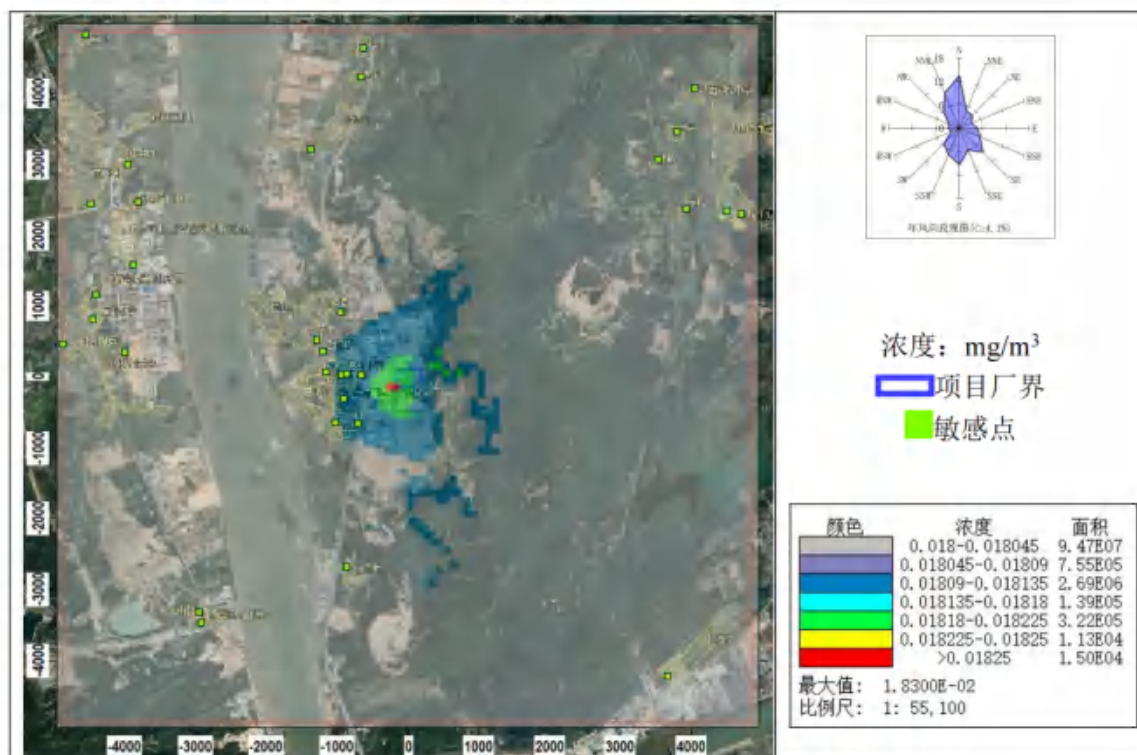
图 8.2-22 \text{PM}_{2.5} 年平均浓度分布图 (叠加在建、拟建源及背景后)
