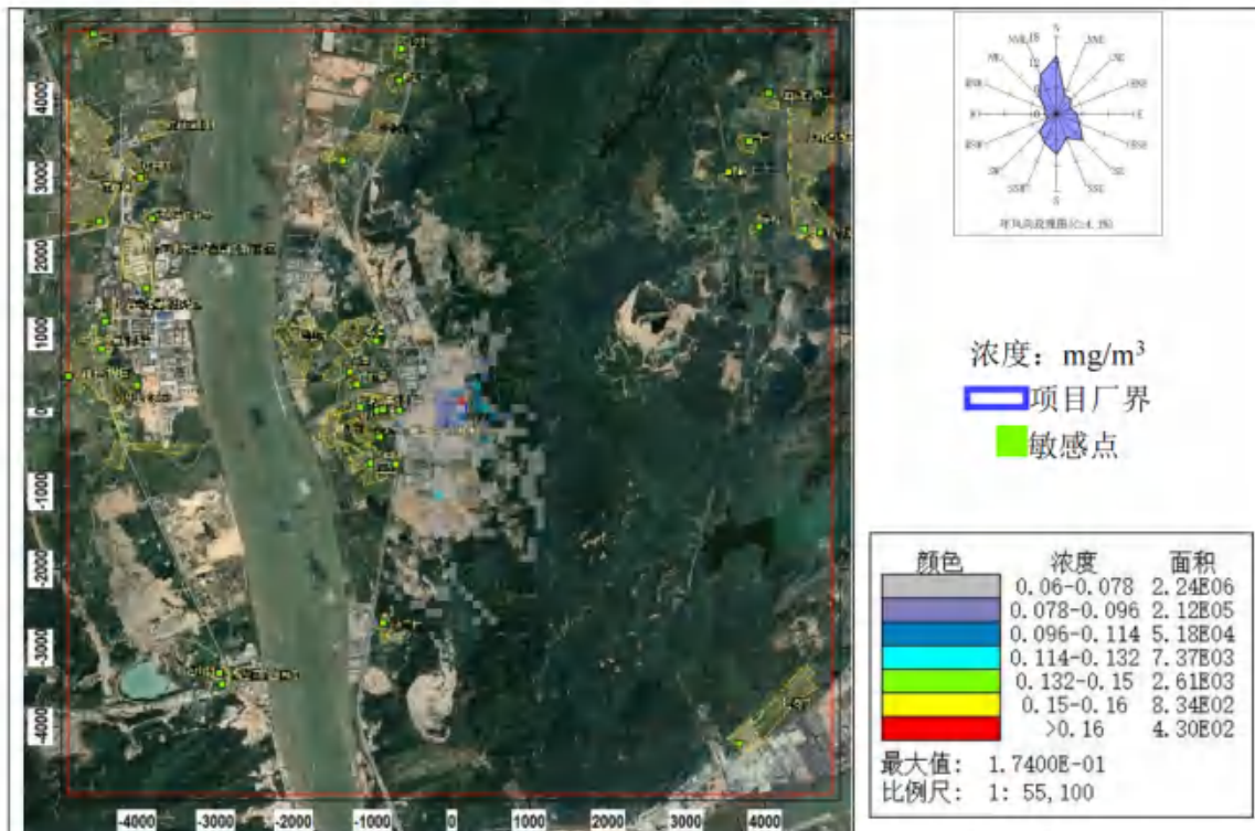
图 8.2-38 氨气小时平均浓度分布图（叠加在建、拟建源及背景后）
