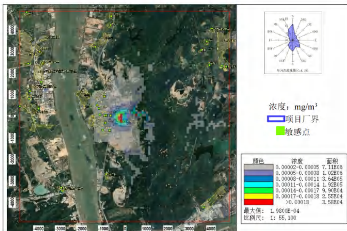
图 8.2-20 \text{PM}_{2.5} 年平均浓度分布图
