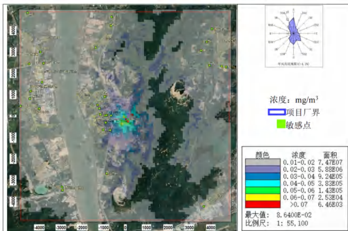
图 8.2-29 硫酸雾小时平均浓度分布图（叠加在建、拟建源及背景后）
