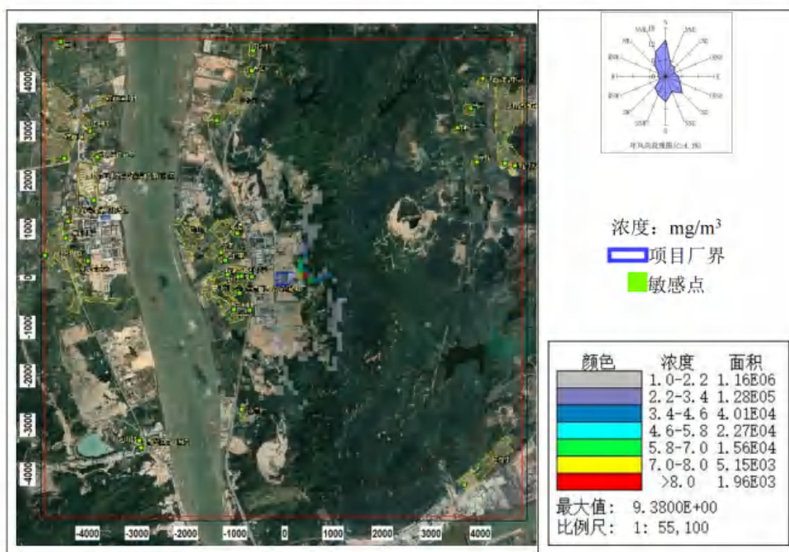
图 8.2-53 HCl 小时平均浓度分布图（非正常排放状况）
