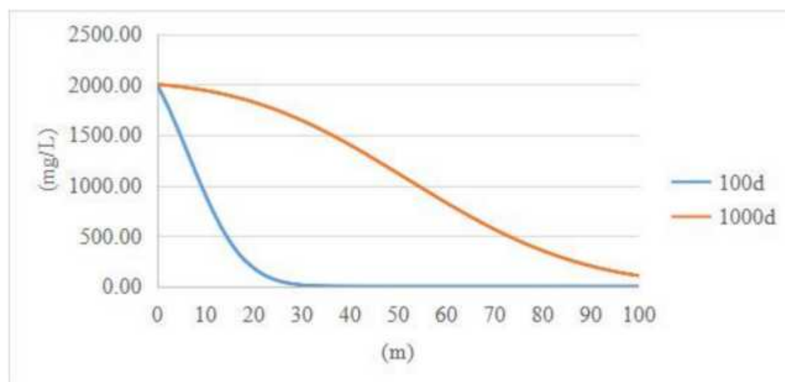
图 8.4-3 污染物连续渗漏情况预测统计图（氟化物）
