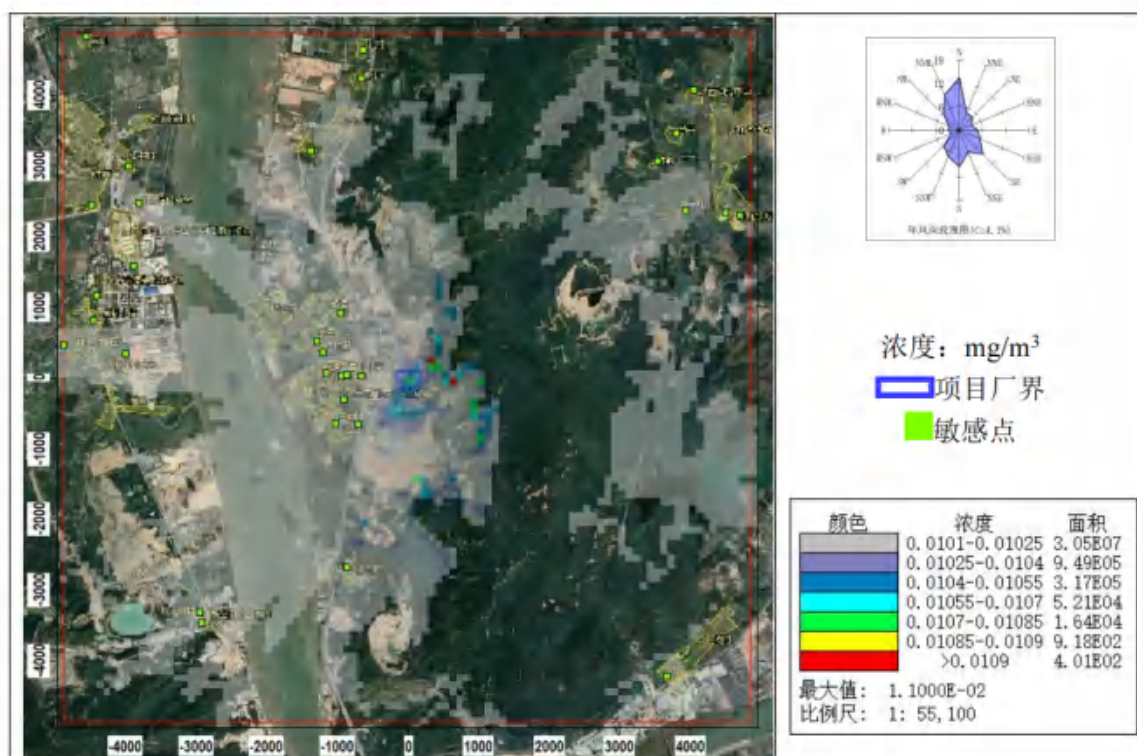
图 8.2-34 HCl 日平均浓度分布图（叠加在建、拟建源及背景后）
