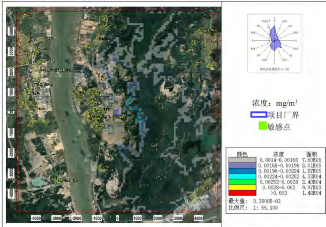
图 8.2-39 氟化物小时平均浓度分布图（叠加在建、拟建源及背景后）
