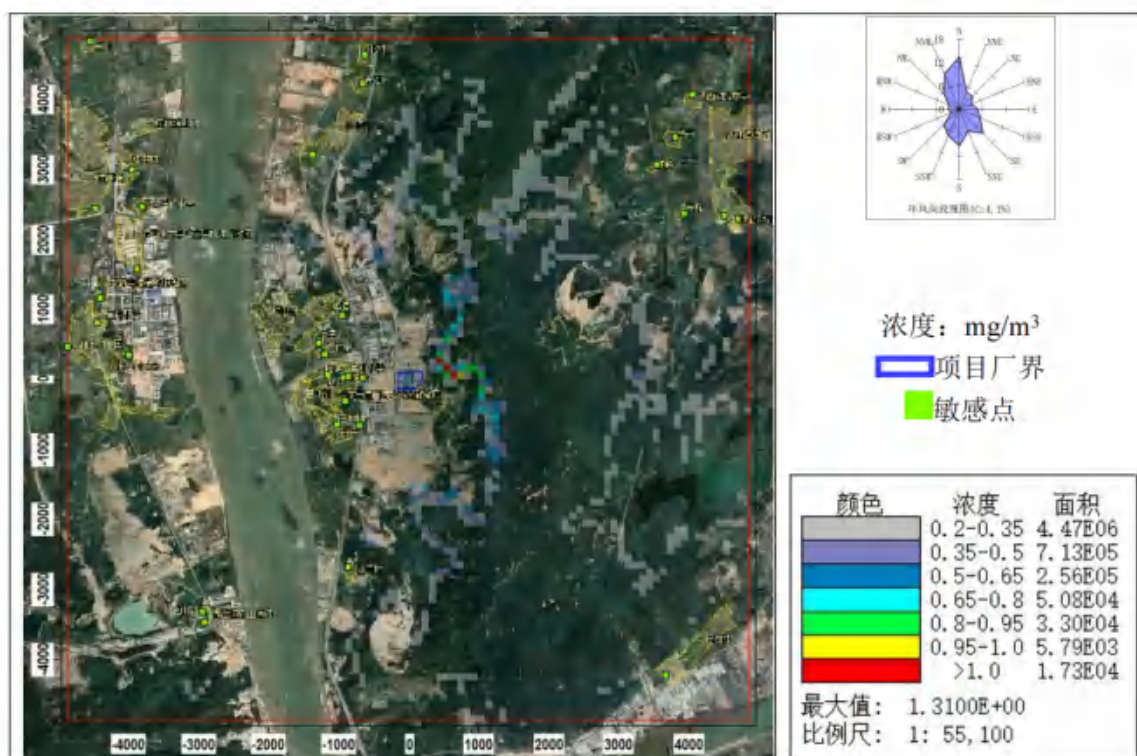
图 8.2-49 \text{PM}_{2.5} 小时平均浓度分布图 (非正常排放状况)
