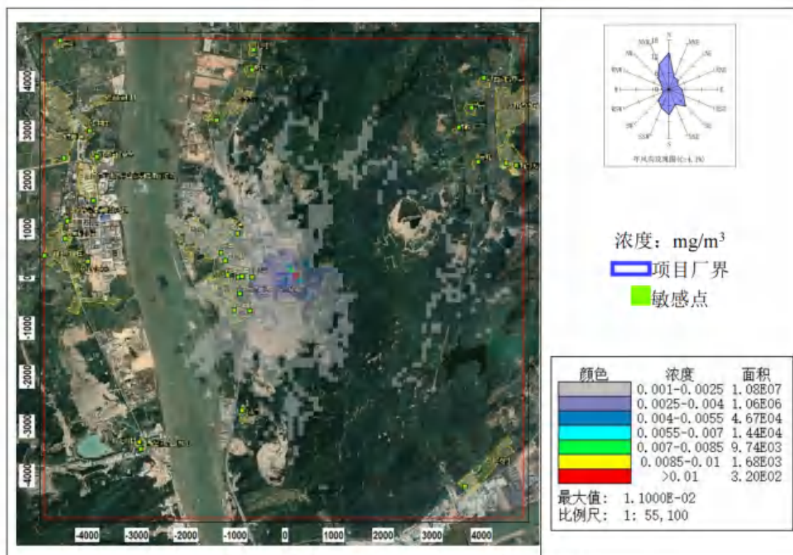
图 8.2-43 镍及其化合物小时平均浓度分布图
