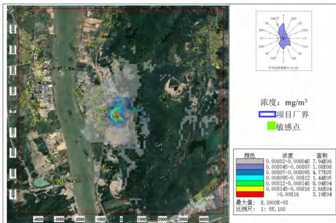
图 8.2-8 \text{SO}_2 年平均浓度分布图 (叠加在建、拟建源及背景后)
