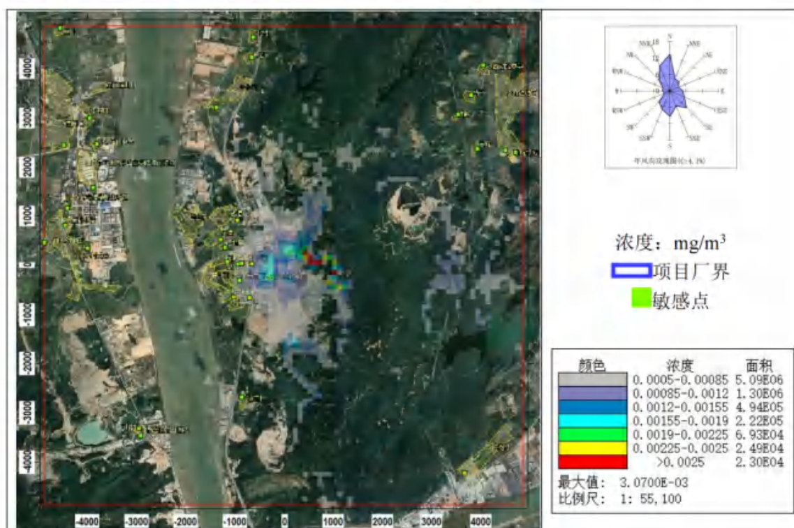
图 8.2-15 \text{PM}_{10} 日平均浓度分布图
