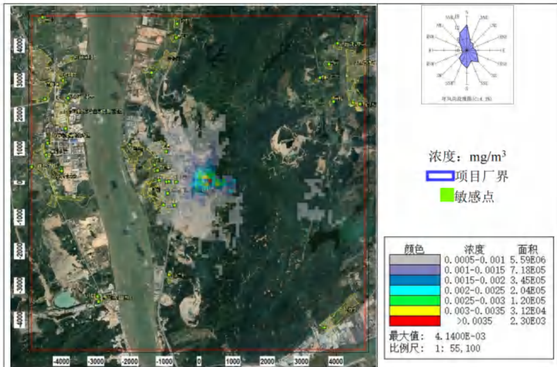
图 8.2-28 硫酸雾日平均浓度分布图
