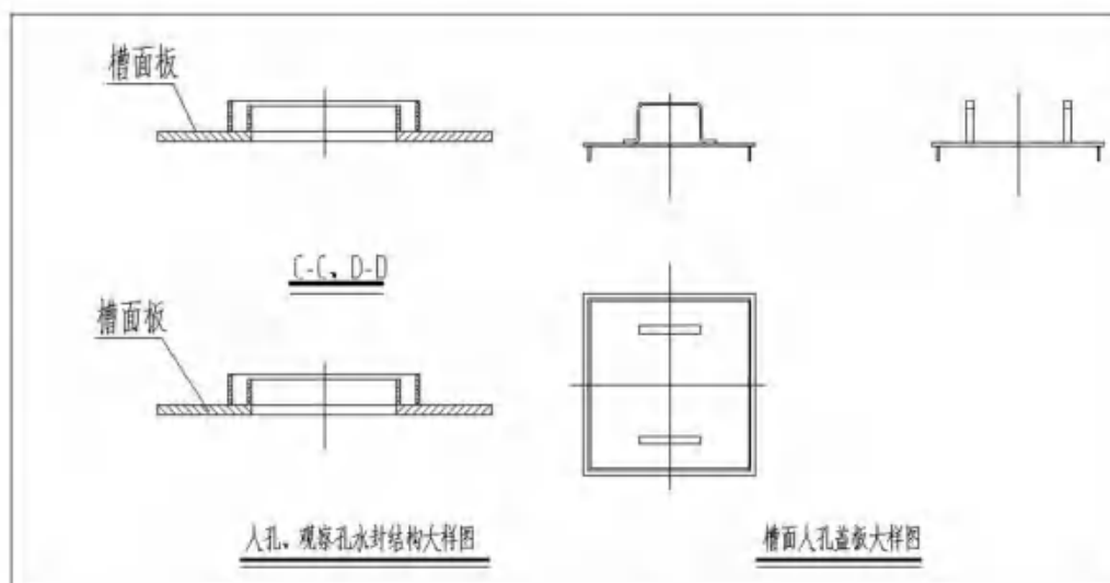
图 4.6-1 萃取槽封闭方式示意图
