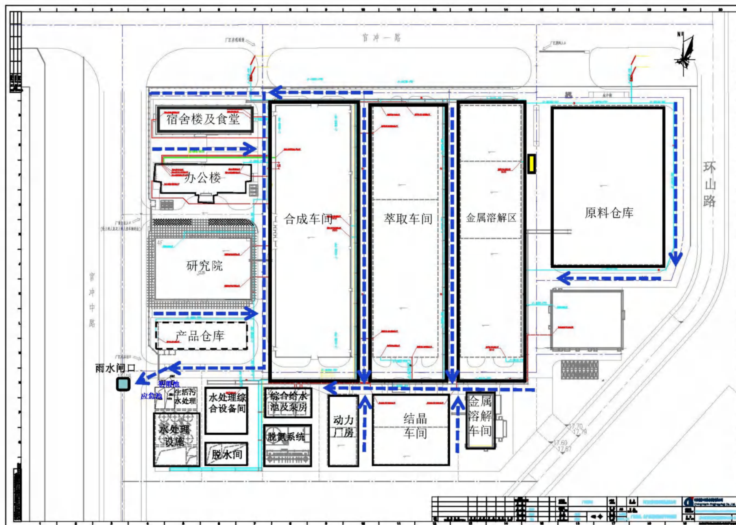
图 9.6-17 雨水收集管网示意图
