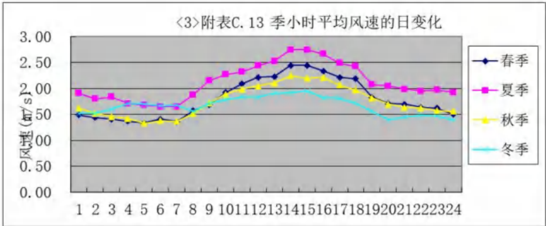
图 8.2-4 季小时平均风速的日变化曲线图
