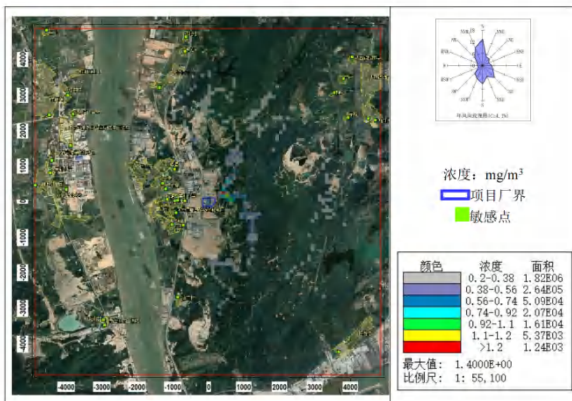
图 8.2-57 氟化物小时平均浓度分布图（非正常排放状况）
