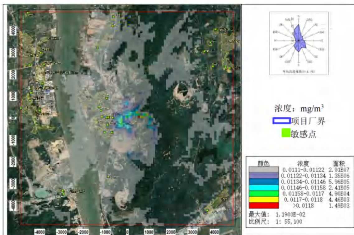
图 8.2-7 \text{SO}_2 日平均浓度分布图 (叠加在建、拟建源及背景后)
