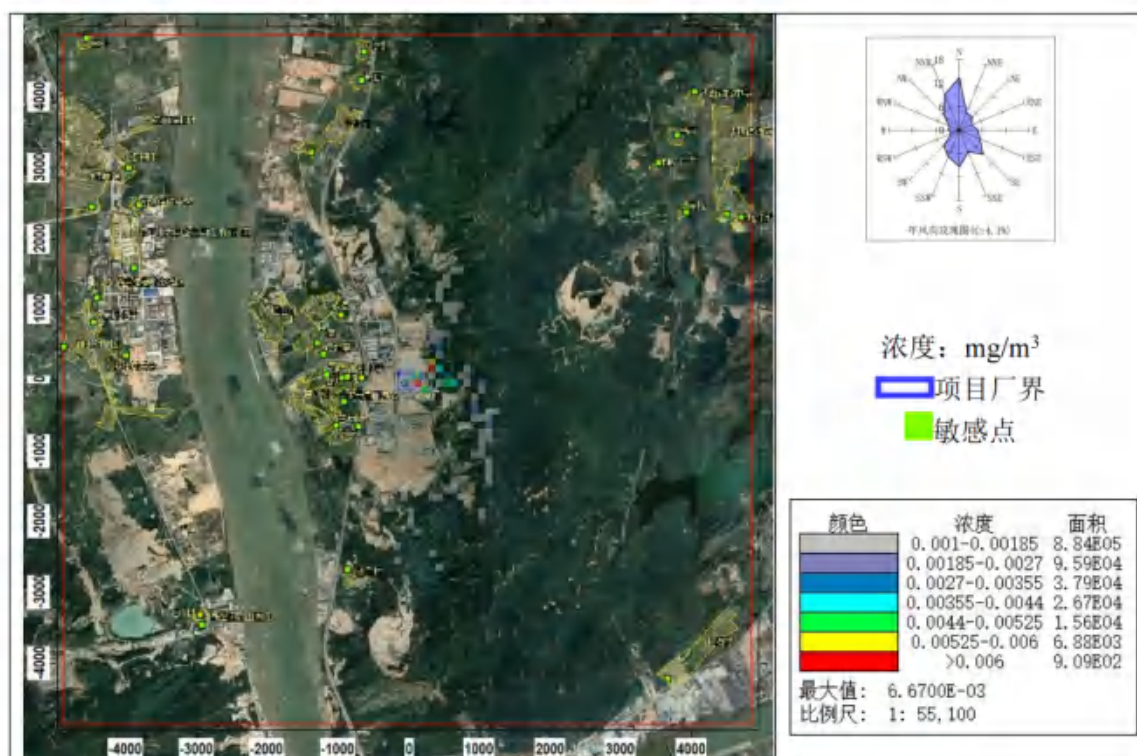
图 8.2-31 HCl 小时平均浓度分布图
