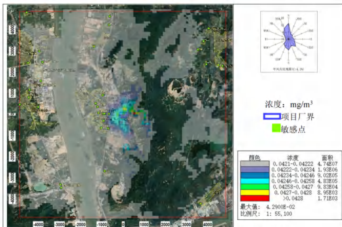
图 8.2-21 \text{PM}_{2.5} 日平均浓度分布图 (叠加在建、拟建源及背景后)
