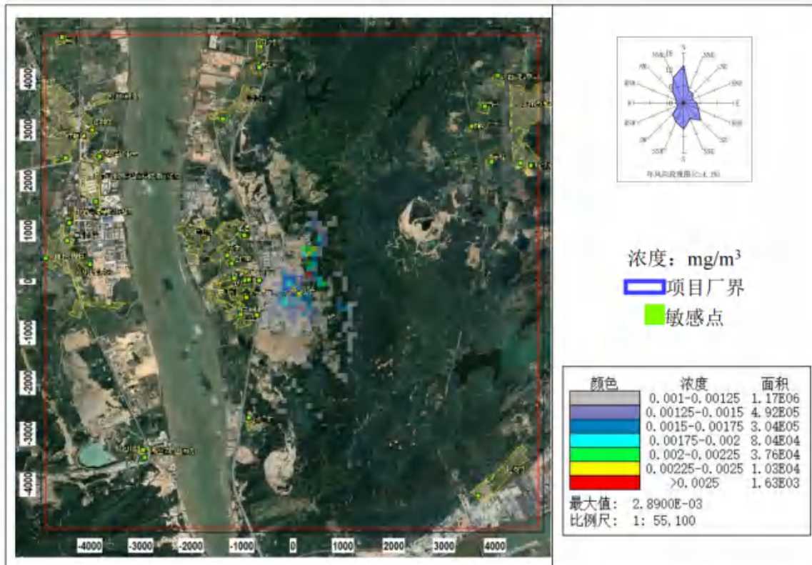
图 8.2-42 硫化氢小时平均浓度分布图（叠加在建、拟建源及背景后）
