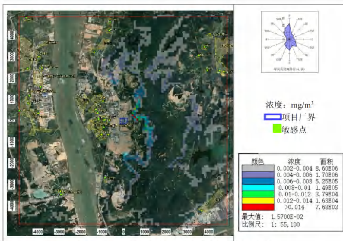
图 8.2-45 \text{SO}_2 小时平均浓度分布图 (非正常排放状况)
