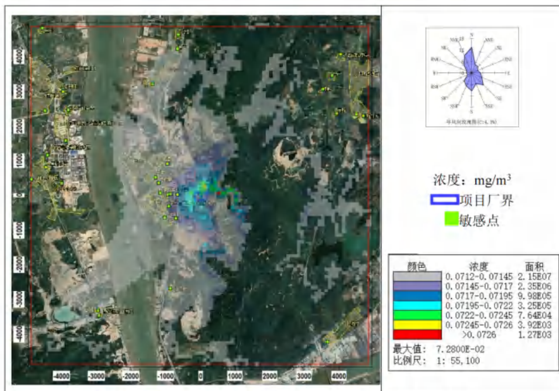
图 8.2-17 \text{PM}_{10} 日平均浓度分布图 (叠加在建、拟建源及背景后)
