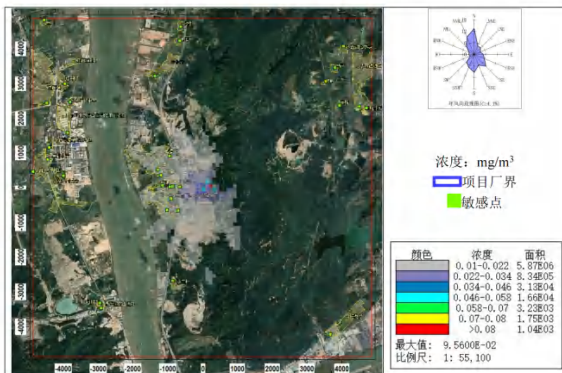
图 8.2-47 TSP 小时平均浓度分布图 (非正常排放状况)
