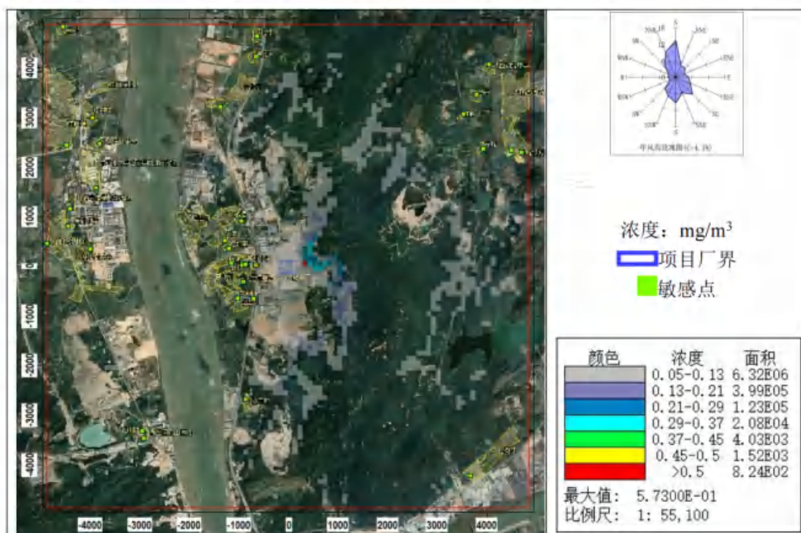
图 8.2-52 硫酸雾小时平均浓度分布图（非正常排放状况）
