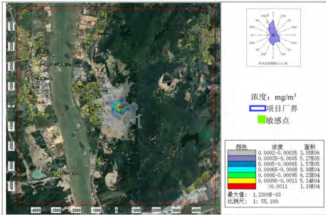
图 8.2-36 锰及其化合物日平均浓度分布图（叠加在建、拟建源及背景后）
