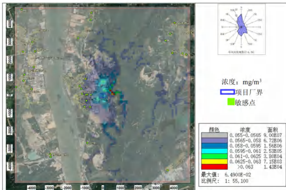
图 8.2-9 \text{NO}_2 日平均浓度分布图 (叠加在建、拟建源及背景后)
