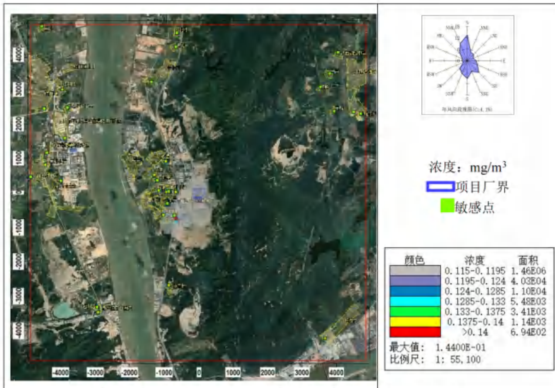
图 8.2-14 TSP 年平均浓度分布图（叠加在建、拟建源及背景后）
