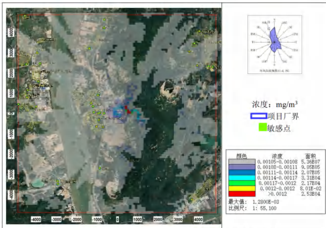
图 8.2-40 氟化物日平均浓度分布图（叠加在建、拟建源及背景后）
