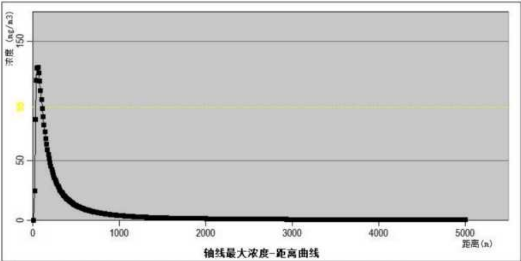
图 9.6-13 电池包仓火灾最不利气象条件下主要受影响关心点的浓度随时间变化（CO） 单位：mg/m 3
