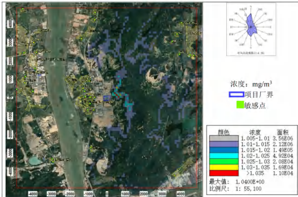
图 8.2-24 NMHC 小时平均浓度分布图（叠加在建、拟建源及背景后）
