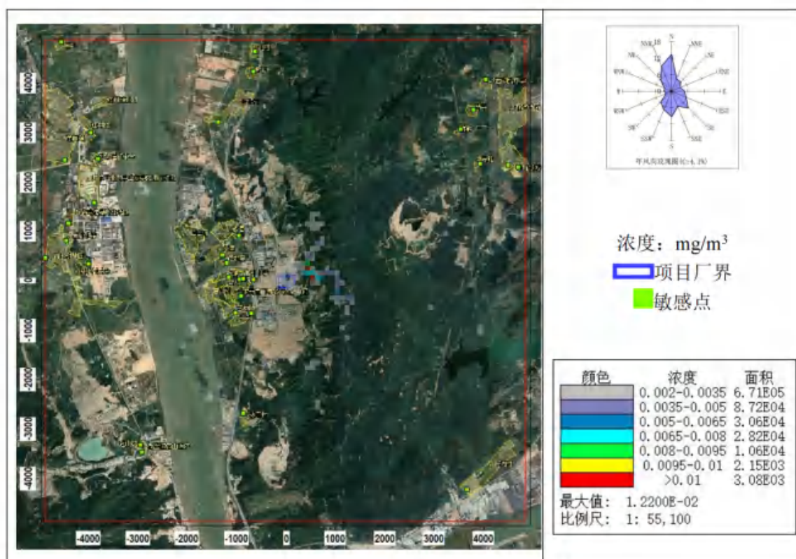
图 8.2-25 TVOC 8 小时平均浓度分布图
