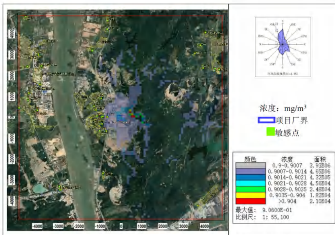
图 8.2-44 CO 日平均浓度分布图 (叠加在建、拟建源及背景后)
