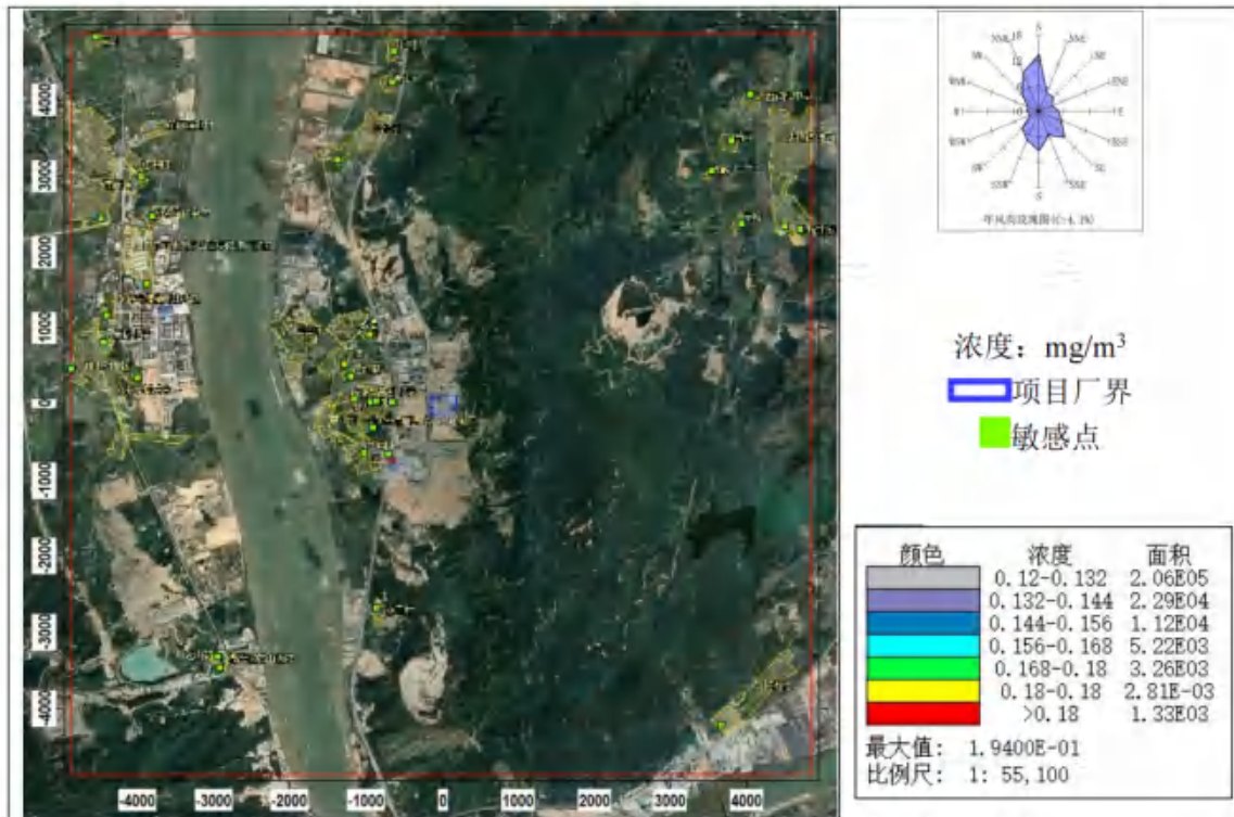
图 8.2-13 TSP 日平均浓度分布图（叠加在建、拟建源及背景后）
