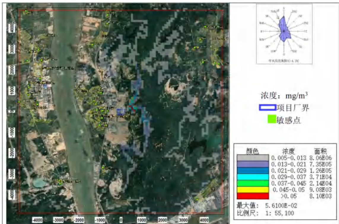
图 8.2-60 CO 小时平均浓度分布图（非正常排放状况）
