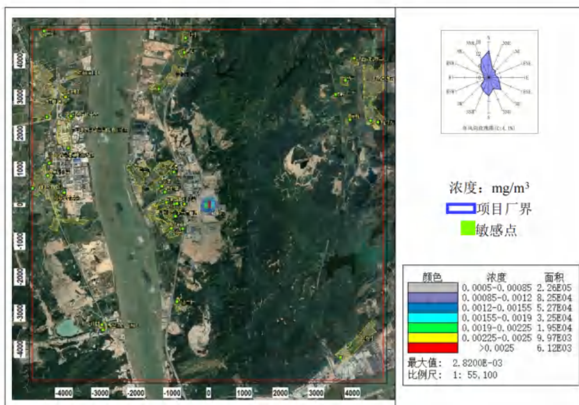
图 8.2-12 TSP 年平均浓度分布图
