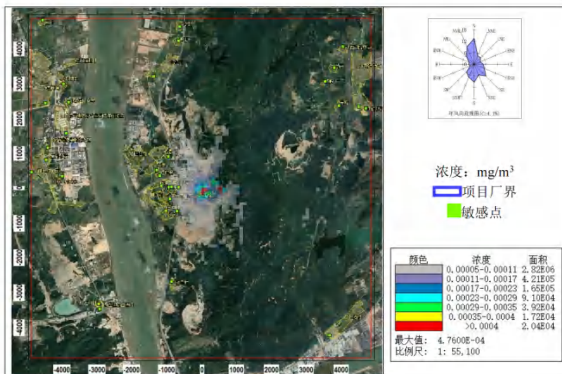
图 8.2-32 HCl 日平均浓度分布图
