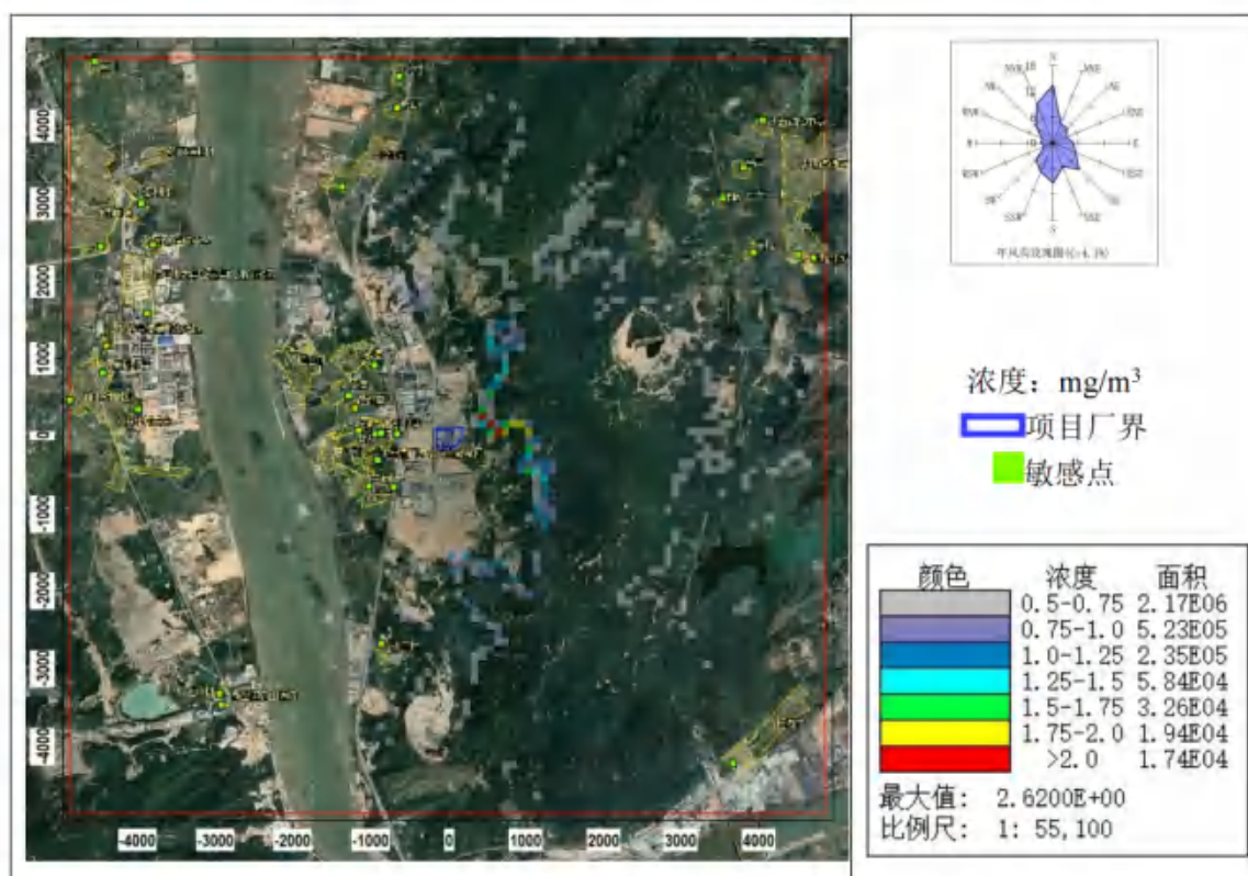
图 8.2-48 \text{PM}_{10} 小时平均浓度分布图 (非正常排放状况)
