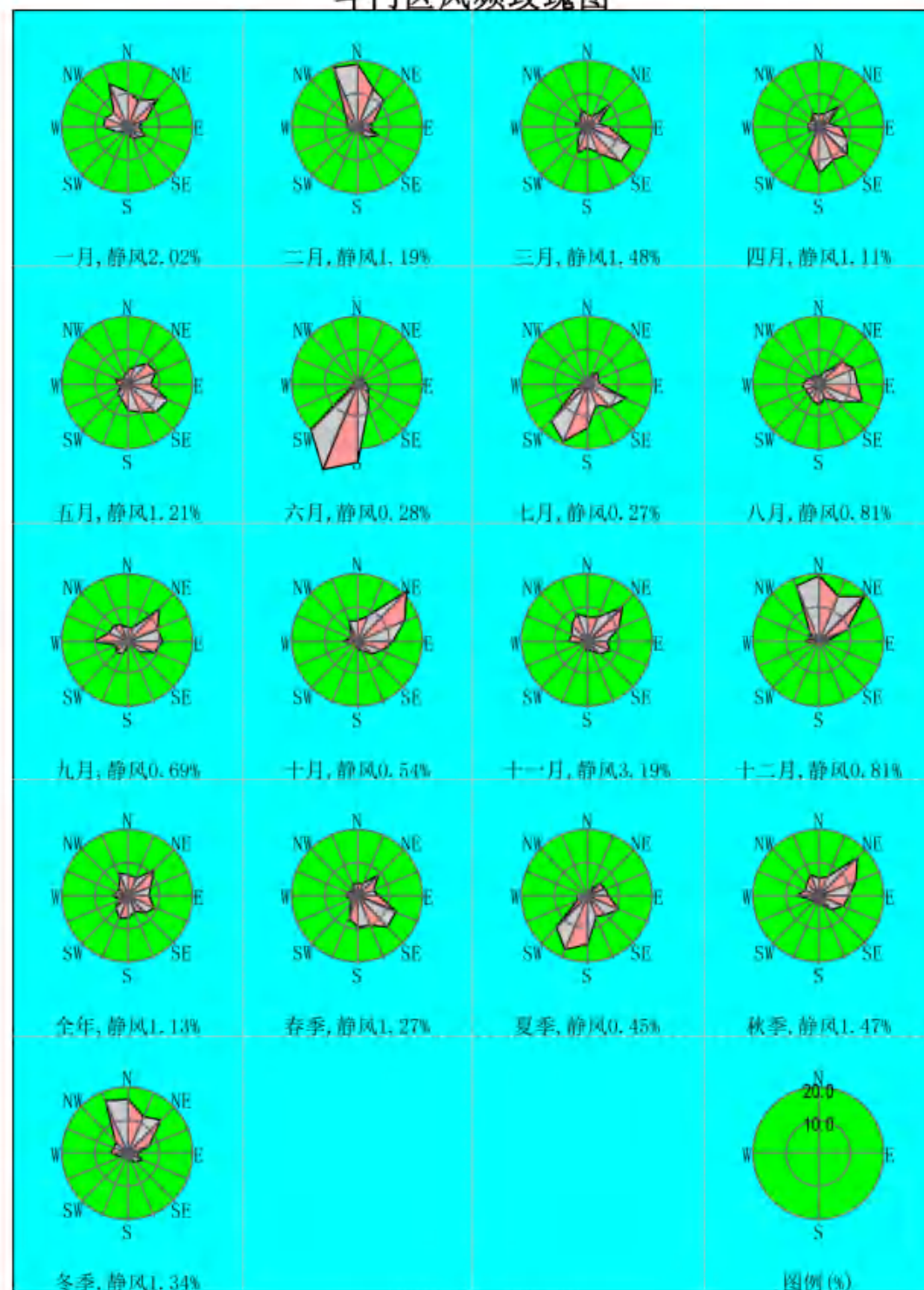
图 8.2-5 风频玫瑰图
