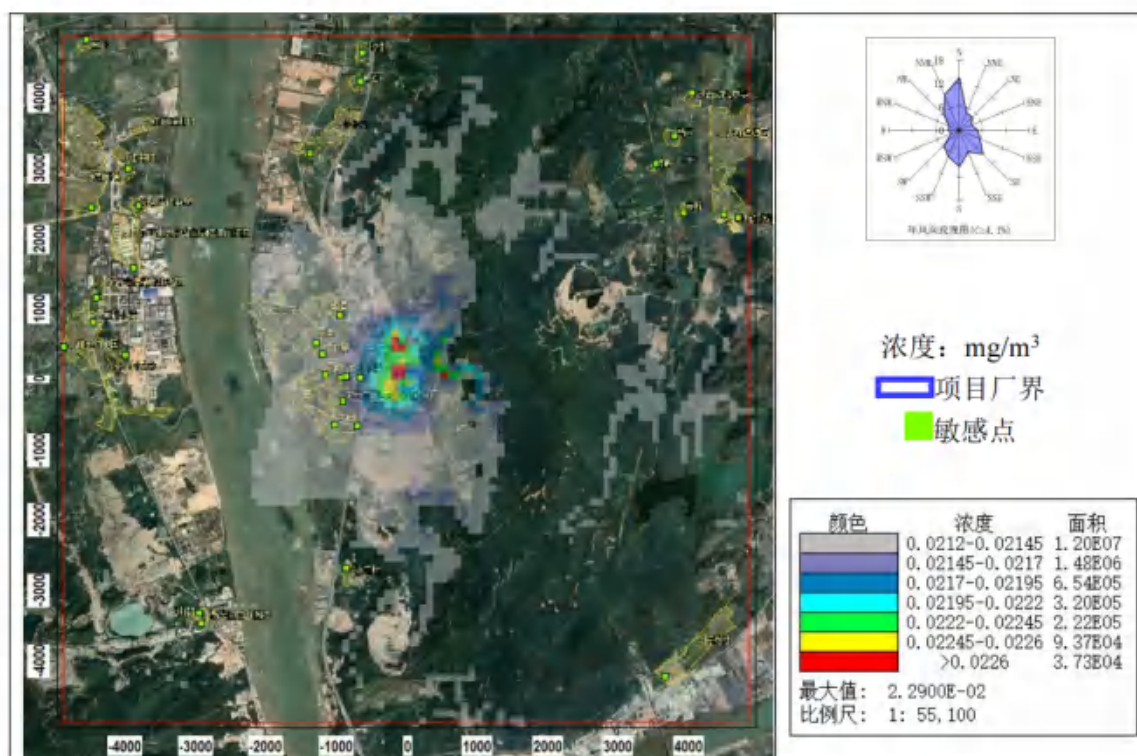
图 8.2-10 \text{NO}_2 年平均浓度分布图 (叠加在建、拟建源及背景后)
