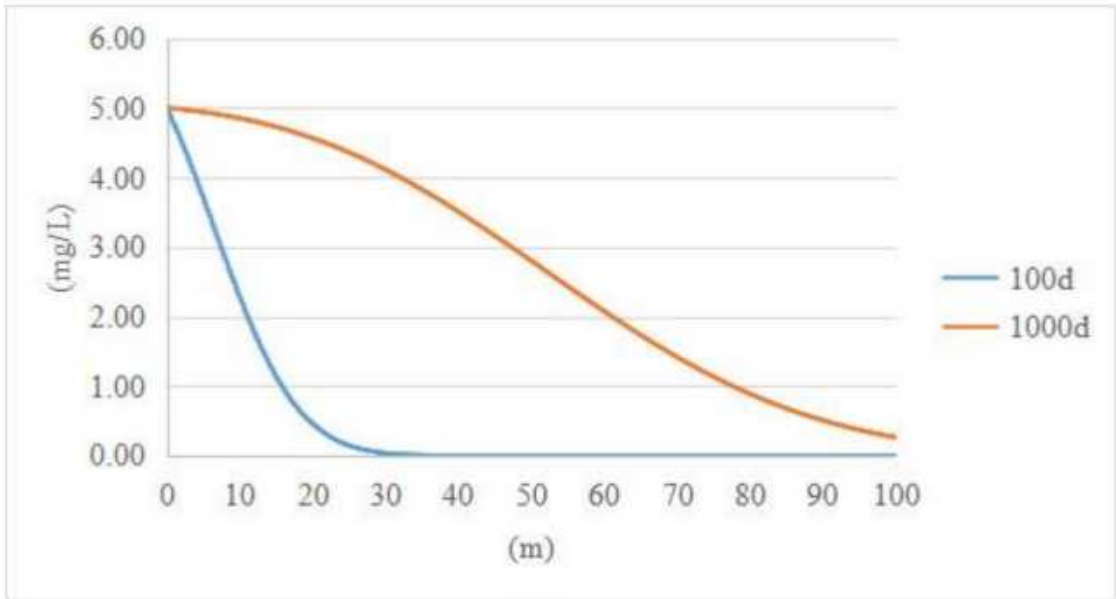
图 8.4-4 污染物连续渗漏情况预测统计图（镍）
