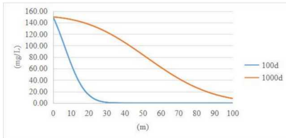
图 8.4-2 污染物连续渗漏情况预测统计图（氨氮）
