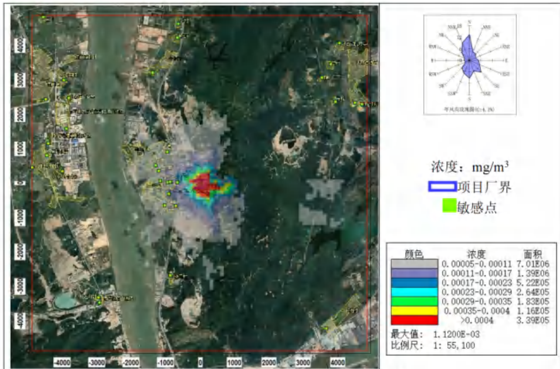
图 8.2-35 锰及其化合物日平均浓度分布图
