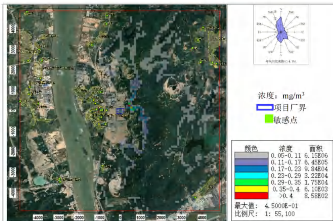
图 8.2-59 镍及其化合物小时平均浓度分布图（非正常排放状况）
